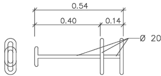
CLAVILLA D'UNIO
