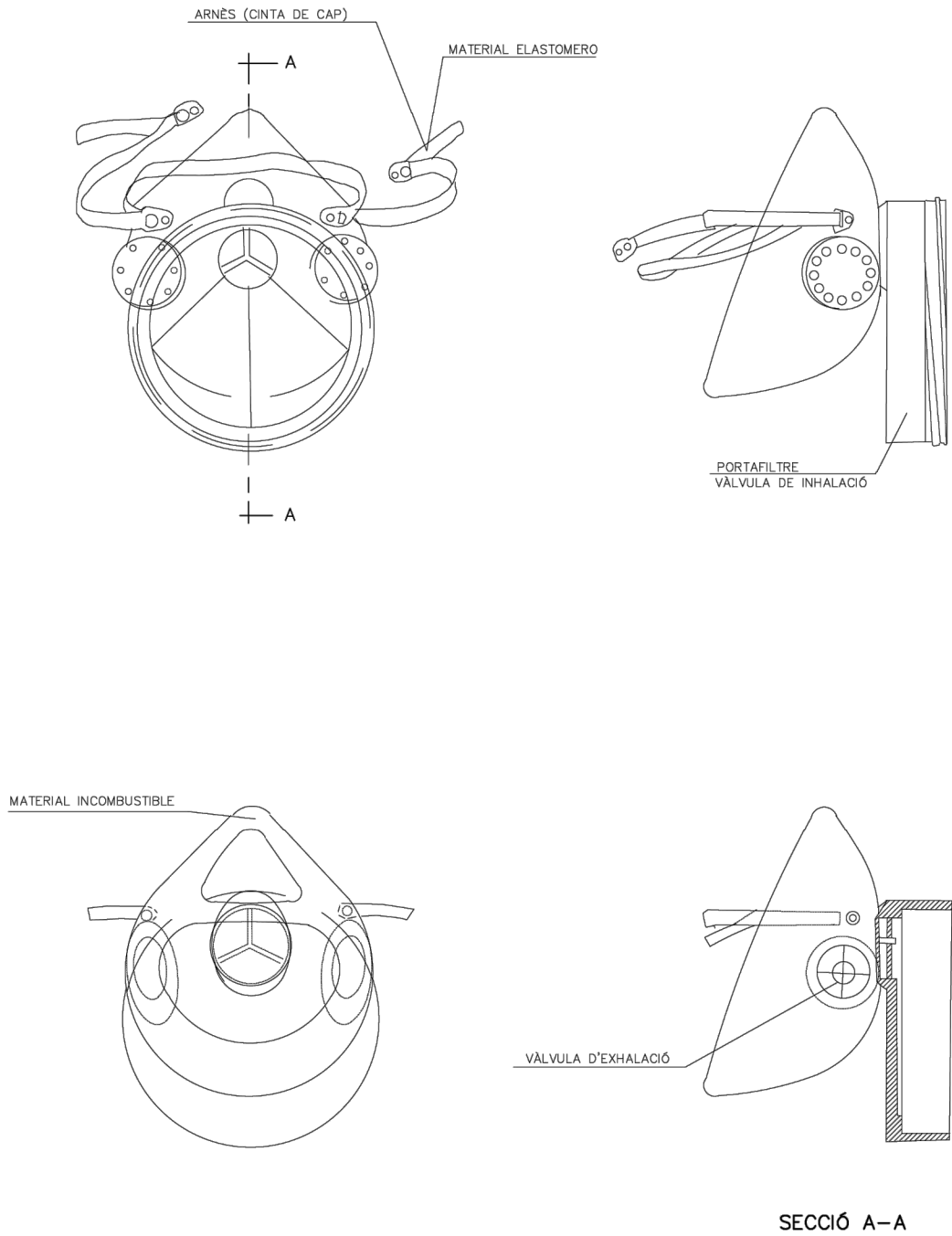
SECCIÓ A-A
