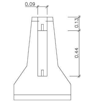
ALÇAT TRANSVERSAL
