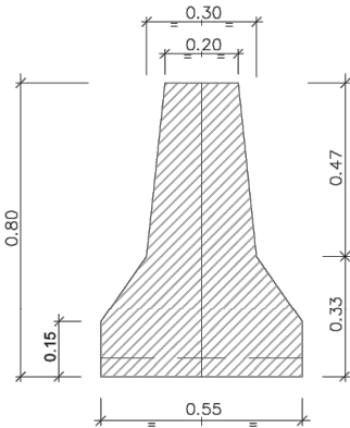
SECCIÓ A-A'
