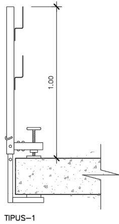
TIPUS-1
