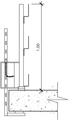
TIPUS-2
