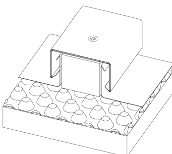
Juntes longitudinals de llistó
