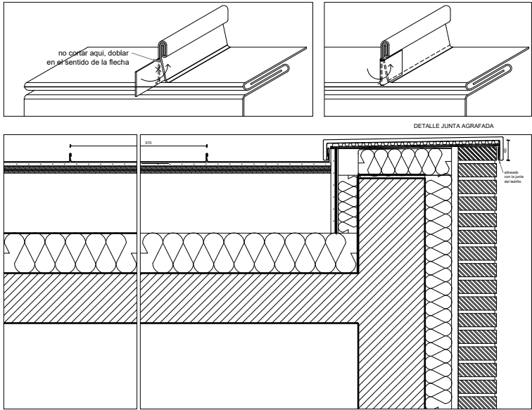
DETALLE 4_ CUBIERTA TIPO E
