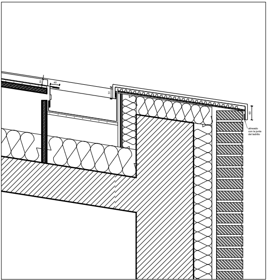
DETALLE 3_ CUBIERTA TIPO G (PUNTO MAS BAJO)
