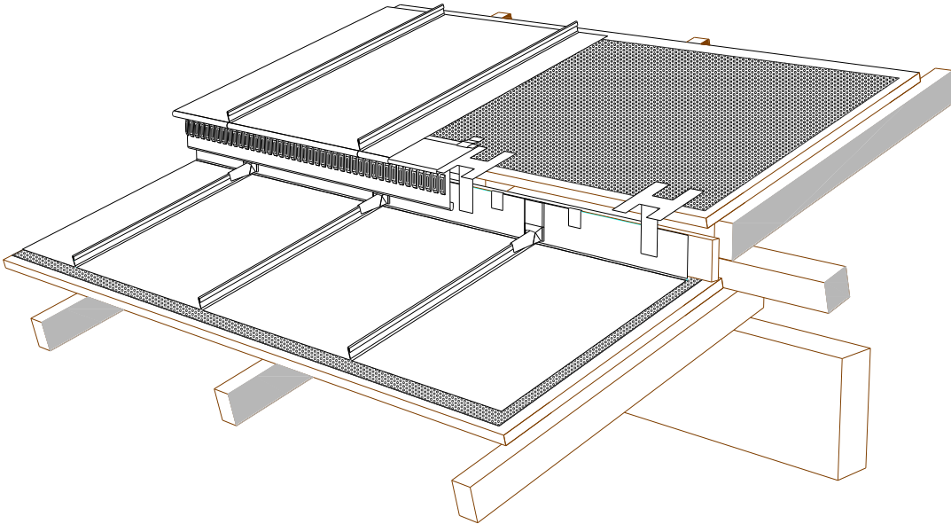
Figura 1. Ejemplo de faldón con junta alzada. Vistas generales y detalle.
