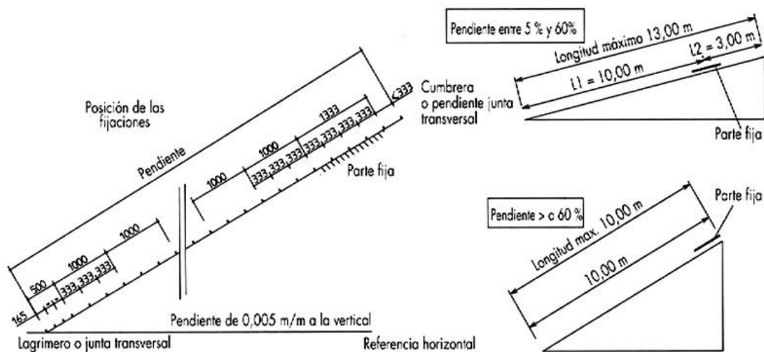
Figura 19. Reparto de patas fijas y correderas (junta alzada)
