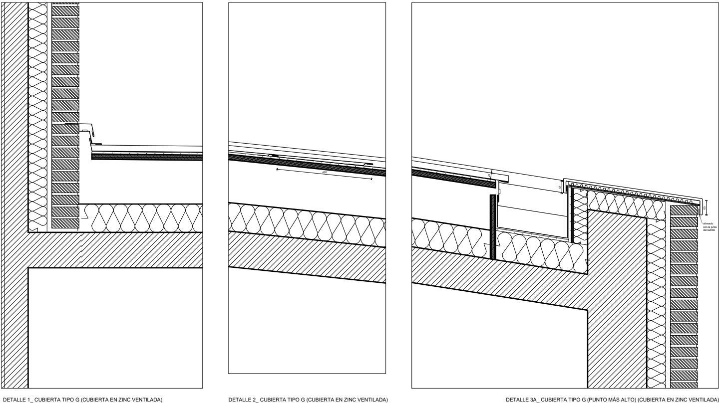
DETALLE 1_ CUBIERTA TIPO G (CUBIERTA EN ZINC VENTILADA)
