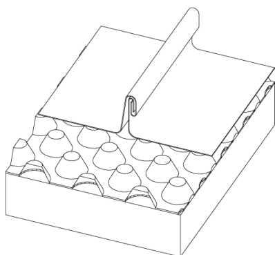
Juntes longitudinals alçades de doble engatillat
