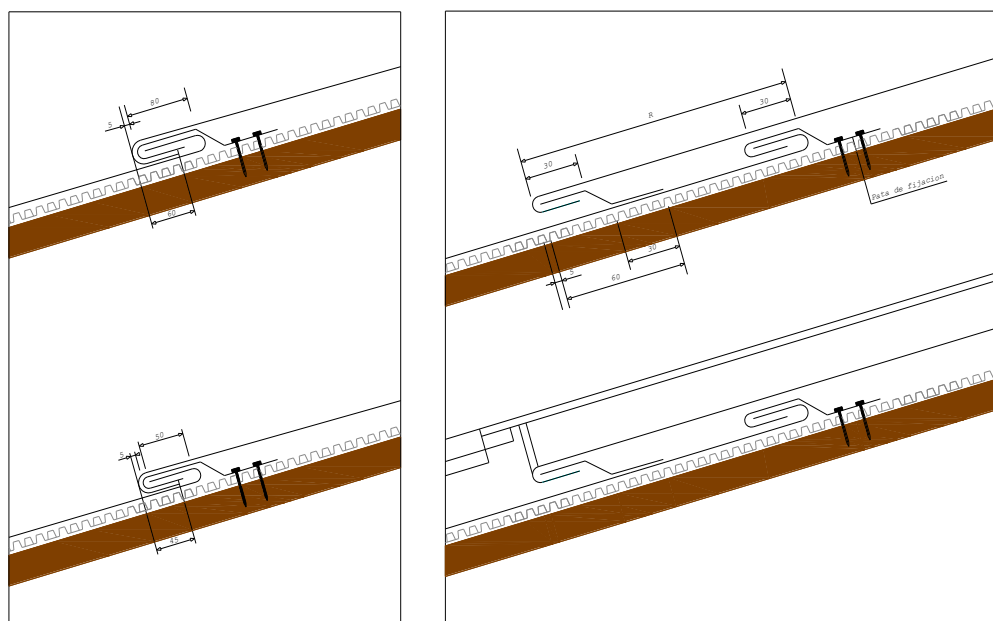
Figura 20: Solape sencillo y doble (bandeja larga)
