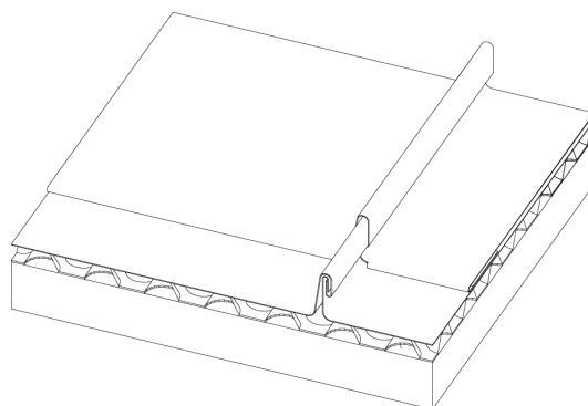
Juntes transversals de solapament
