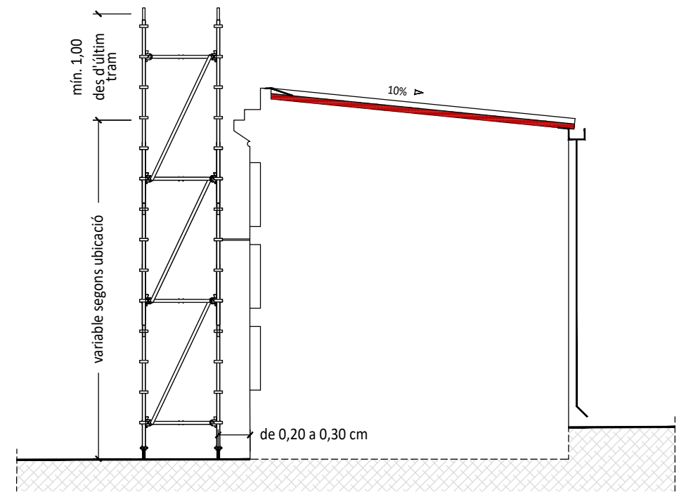
SECCIÓ TIPUS BASTIDA TUBULAR
