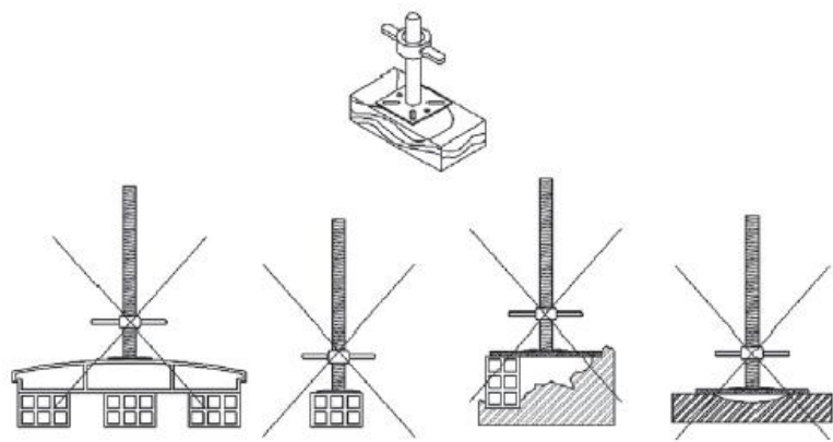
DETALL DE RECOLZAMENT DE LA BASTIDA
