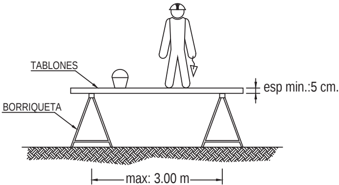
DETALLE DE ANDAMIO DE BORRIQUETAS
