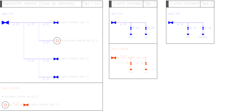
HS 4: Esquema de la instalación interior
