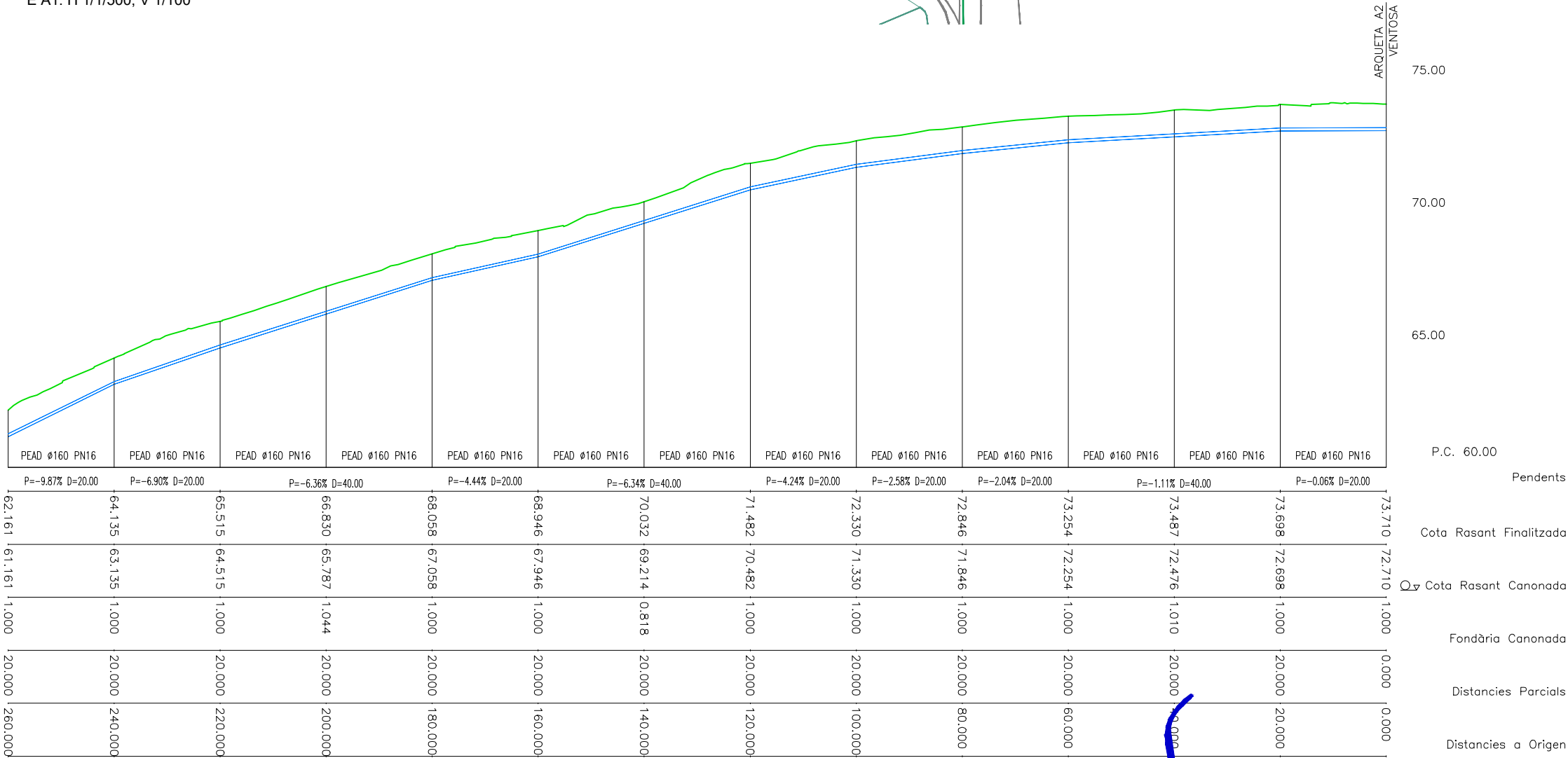
PERFIL LONGITUDINAL PK 0+0,0 - PK 0+260,00 E A3: H 1/1.000; V 1/200 E A1: H 1/1/500; V 1/100
