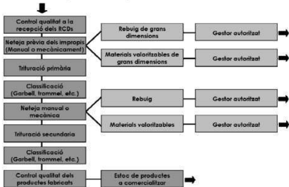
Planta de reciclatge de RCDs barrejats.
