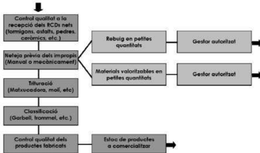
Planta de reciclatge de RCDs nets.
