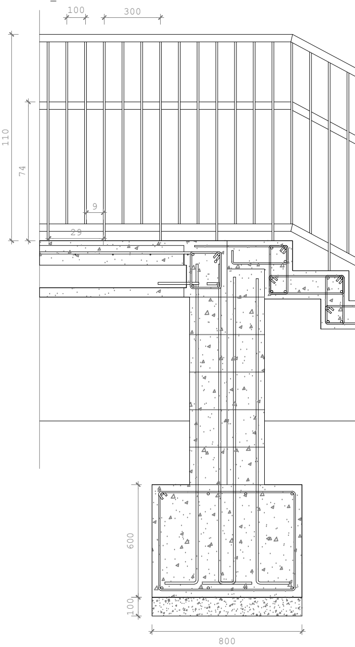
D3_detall secció escala i barana
