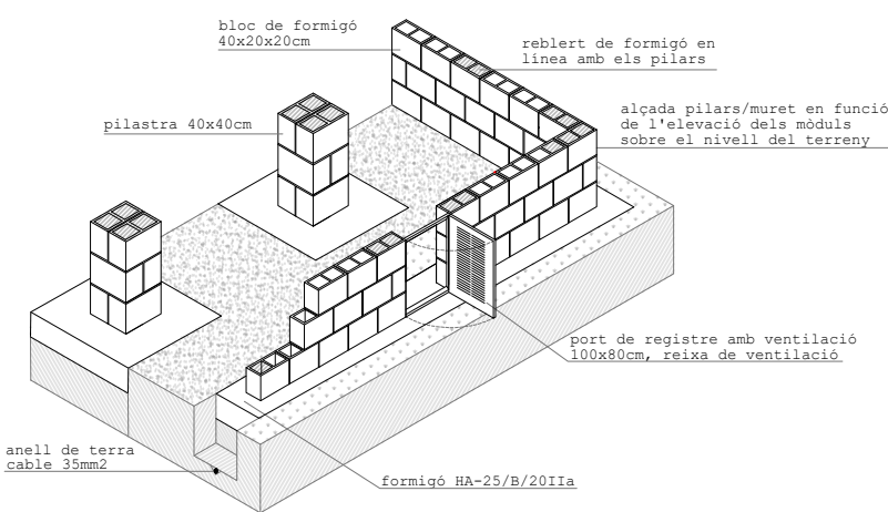
D2_detall registre d'accés a forjat sanitari e:1/100
