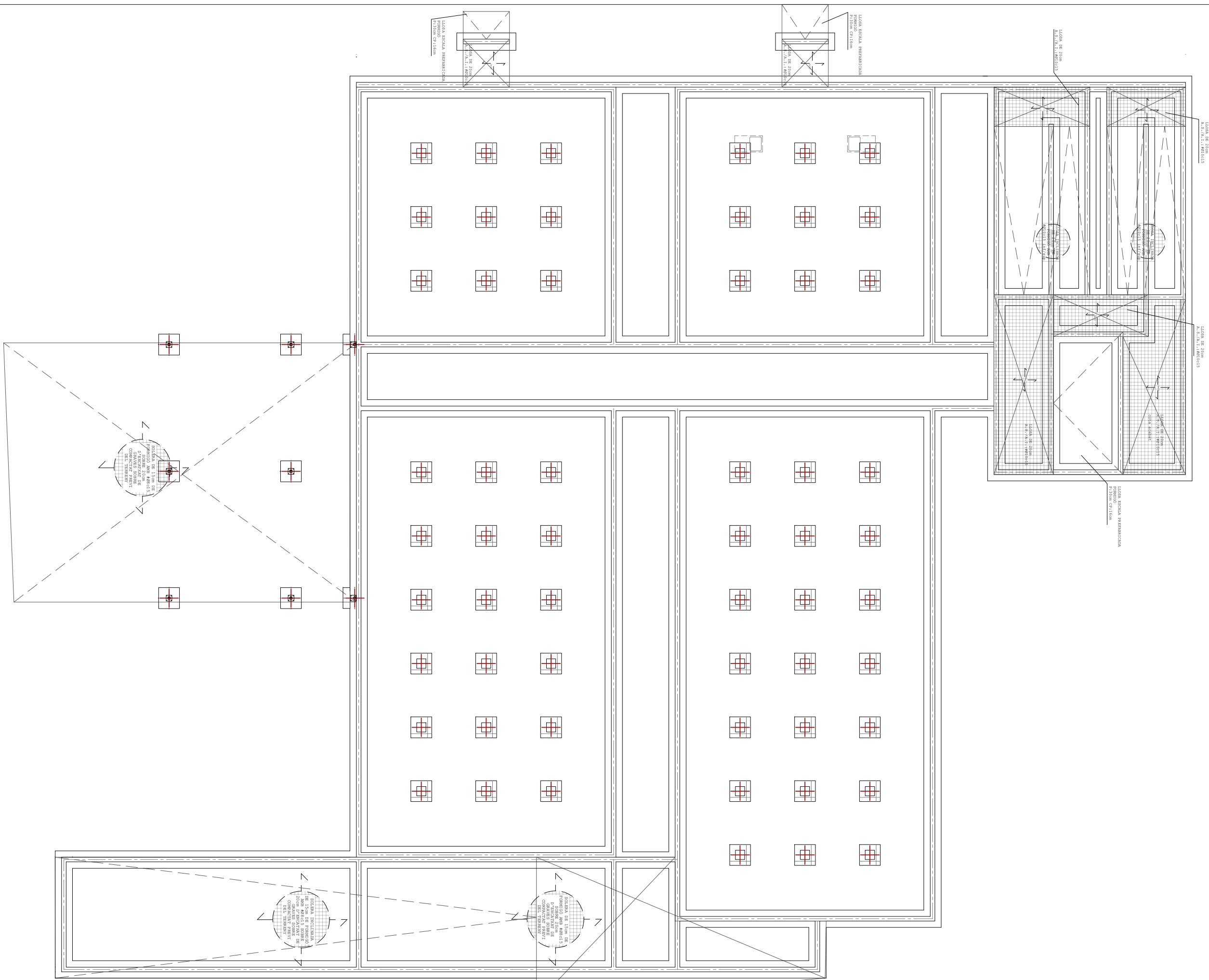
PLANTA ESTRUCTURA DE RAMPES, SOLERES I LLOSES
