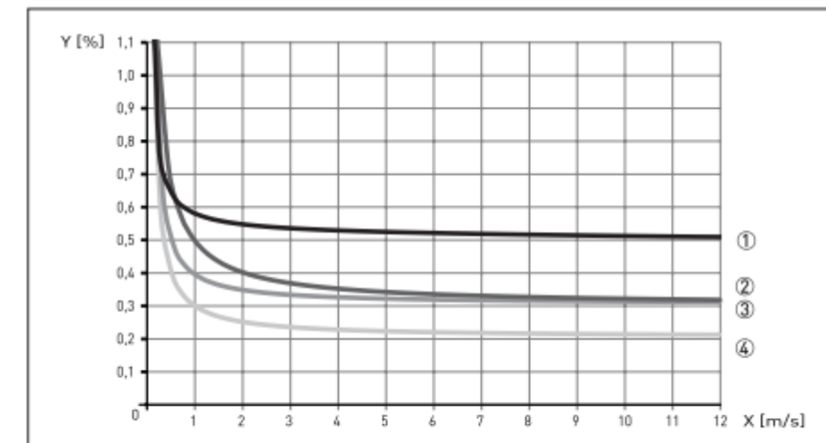
Figura 2-3: Velocidad de caudal frente a precisión
