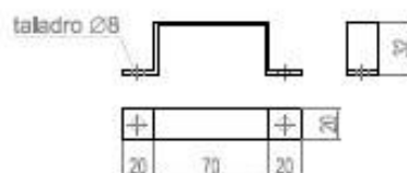
PIEZA 6 ( 1 UNIDAD) ESPESOR DE LA CHAPA: 2 mm.
