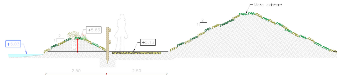
Figura 7. Secció tipus mota perimetral tipus A. Costat Sud.
