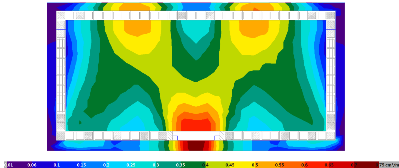
Figura 11. Quantia mínima necessària en X superior
