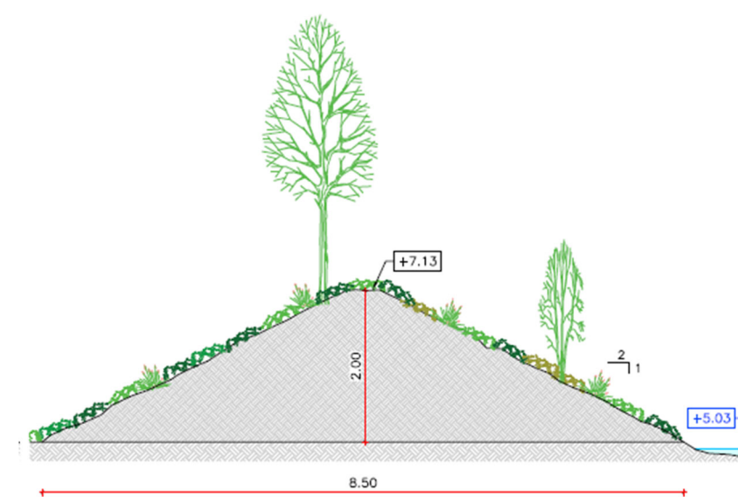
Figura 12. Secció perimetral, mota tipus E
