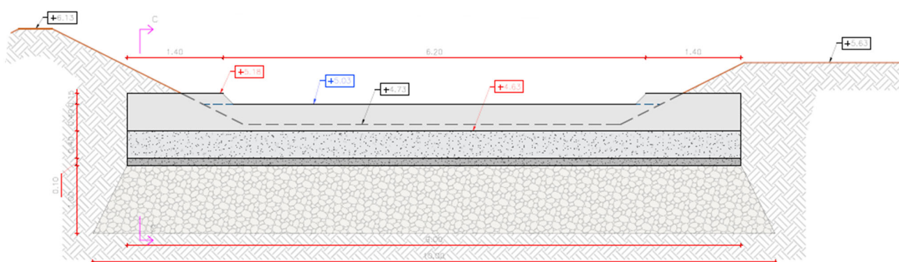
Figura 16. Mur de desguàs. Secció longitudinal.
