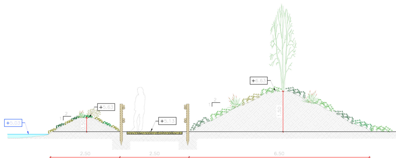
Figura 10. Secció perimetral, mota tipus B. Costat Est.
