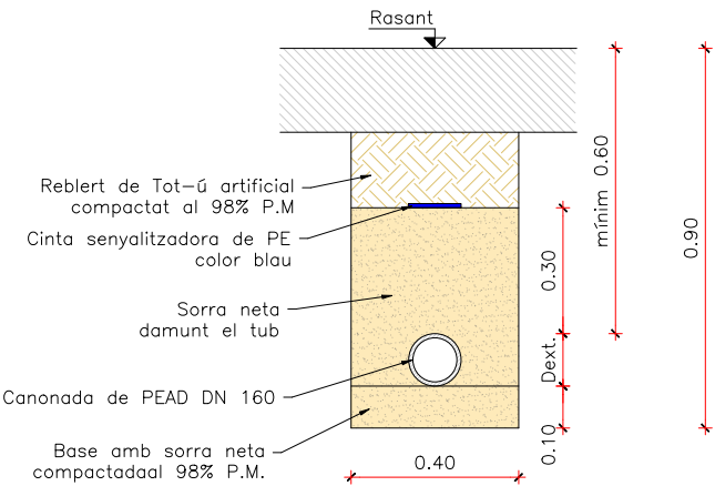
Detall rasa canonada PEAD Esc 1/20
