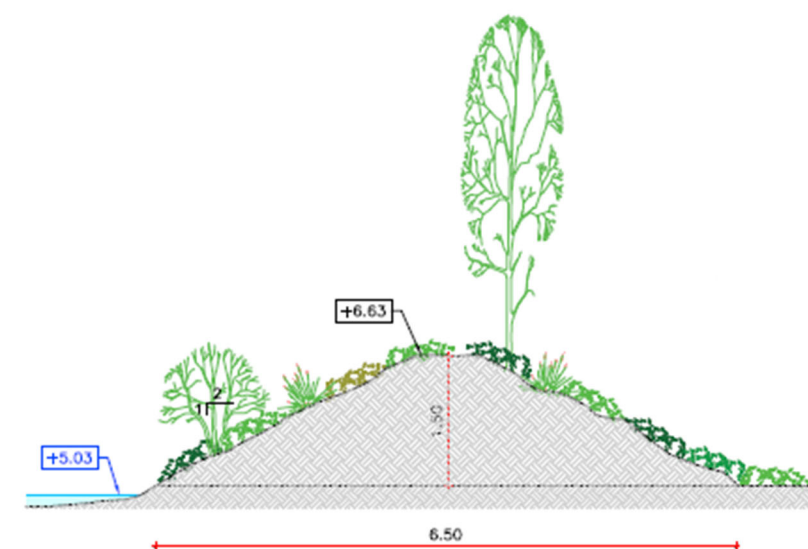
Figura 11. Secció perimetral, mota tipus C
