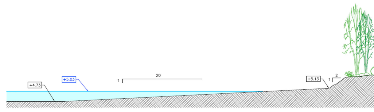
Figura 8. Detall secció tipus illa interior
