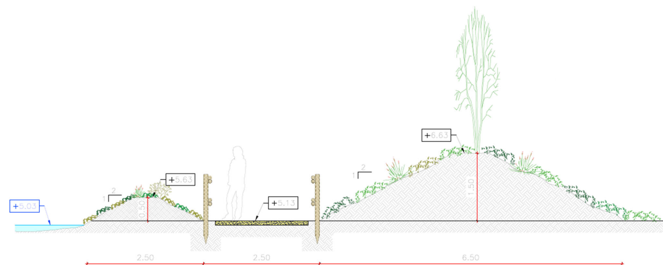
Figura 8. Secció perimetral, mota tipus B. Costat Est.
