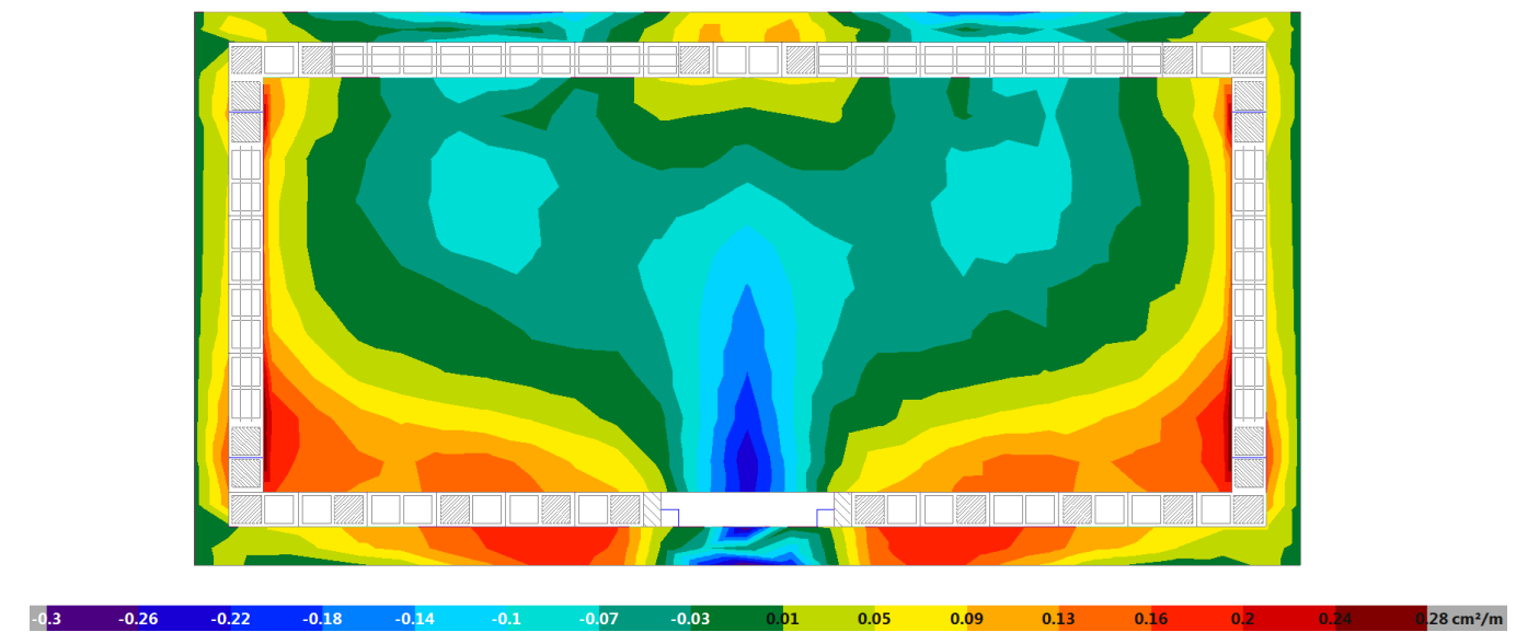
Figura 9. Quantia mínima necessària en X inferior
