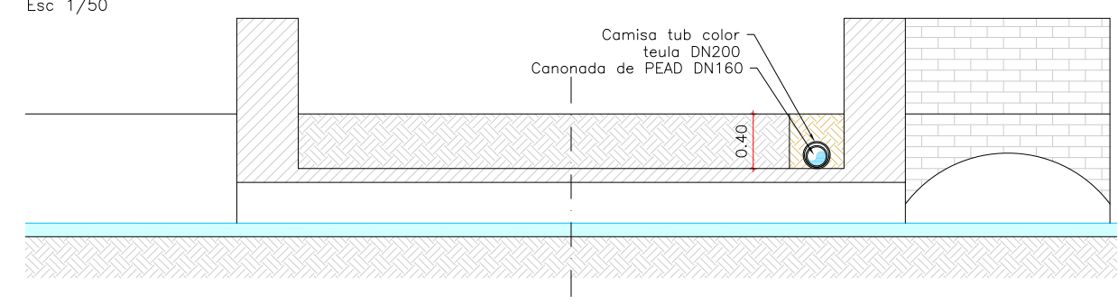
DETALL CREUAMENT PONT SANT FRANCESC SECCIÓ C-C Esc 1/50
