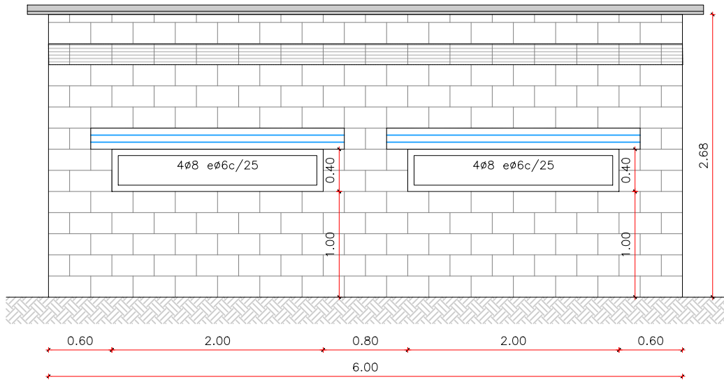
Mur 3
