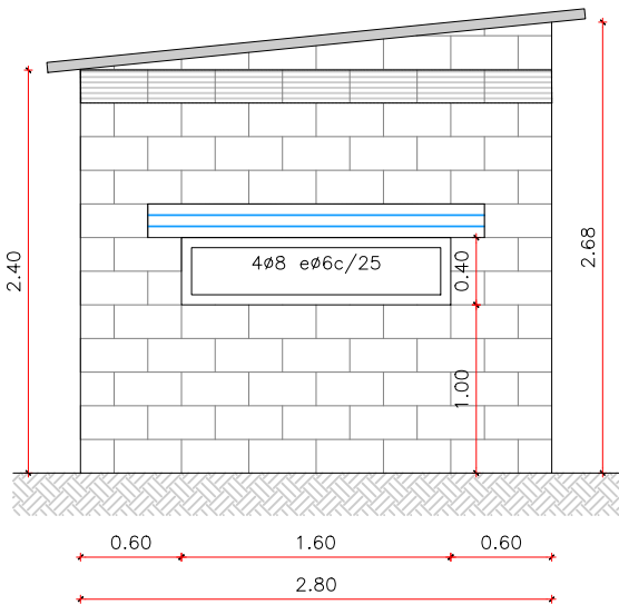
Mur 4
