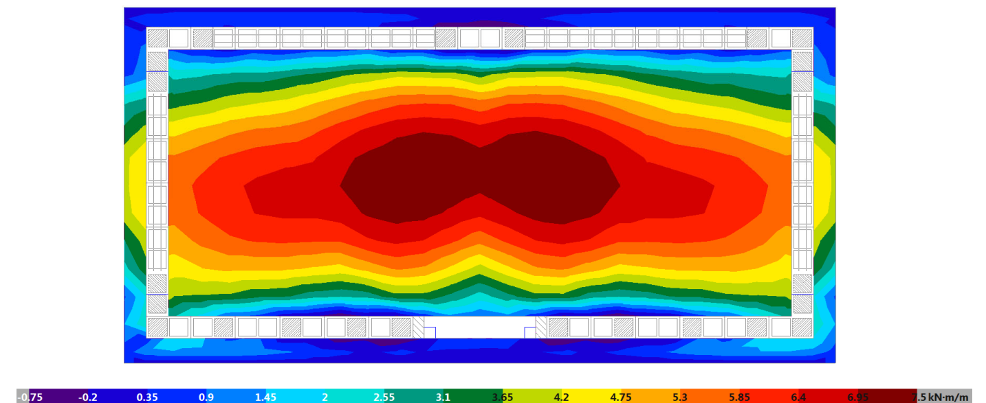
Figura 6. Moment Y, quantia superior
