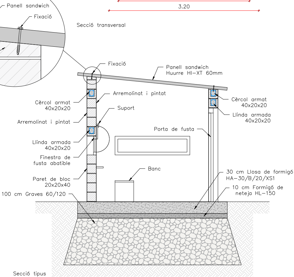
Secció tipus
