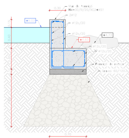
Figura 17. Mur de desguàs. Secció Transversal.
