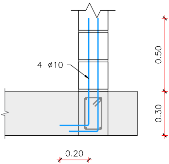
DETALL ESPERES MUR Esc 1/25
