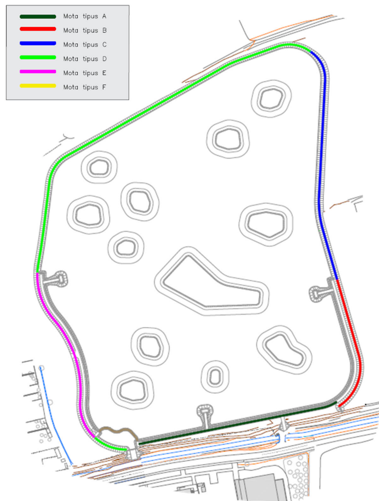
Figura 13. Tipologia de seccions de motes perimetrals
