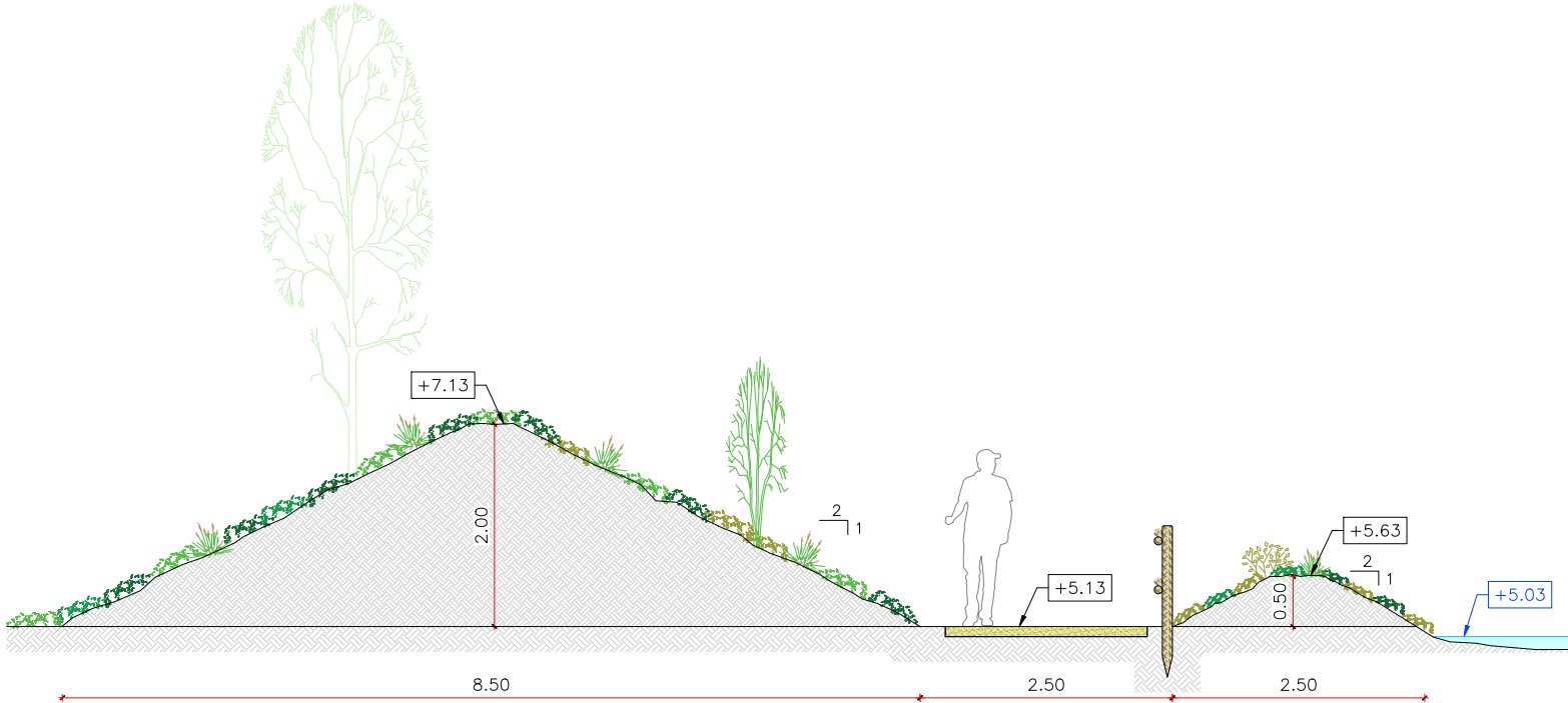
SECCIÓ TIPUS MOTA PERIMETRAL TIPUS F Esc 1/75
