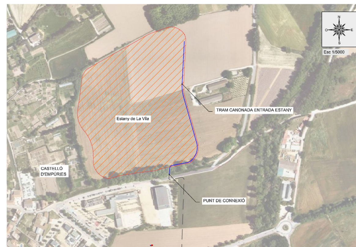
Figura 2. Àmbit de l'actuació i nou tram de canonada d'entrada a l'Estany des del punt de connexió
