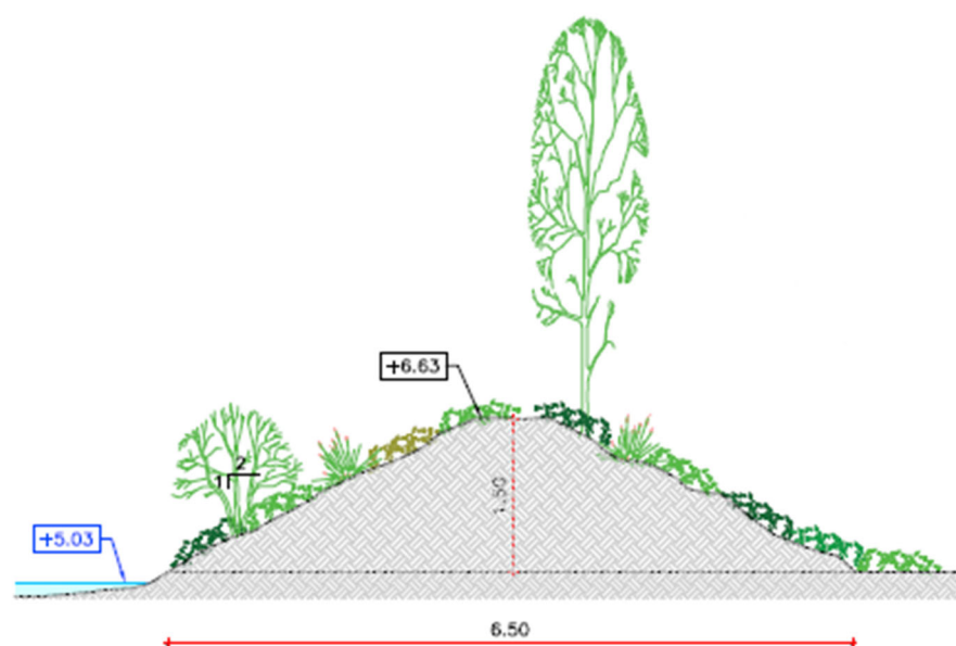
Figura 9. Secció perimetral, mota tipus C
