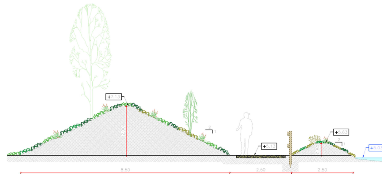
Figura 11. Secció perimetral, mota tipus F. Costat Oest.
