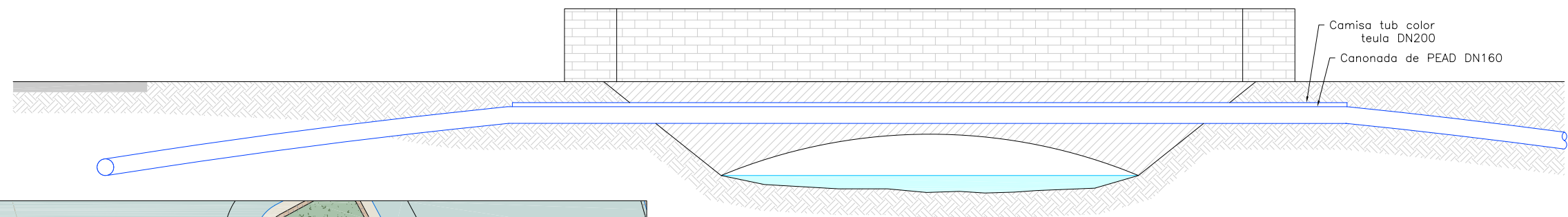
DETALL CREUAMENT PONT DE SANT FRANCESC SECCIÓ B-B Esc 1/50
