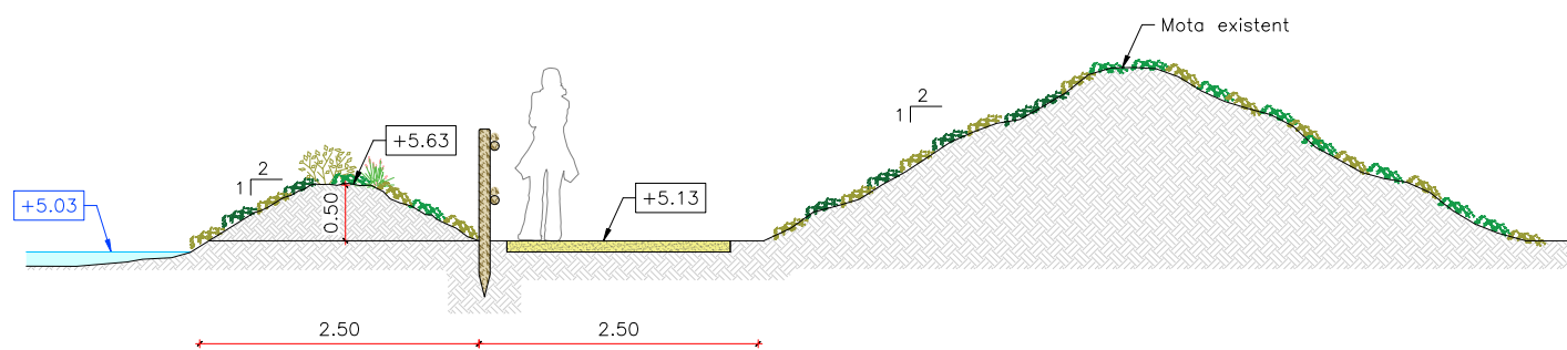
SECCIÓ TIPUS MOTA PERIMETRAL TIPUS A Esc 1/75
