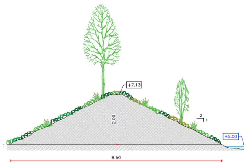
Figura 10. Secció perimetral, mota tipus E
