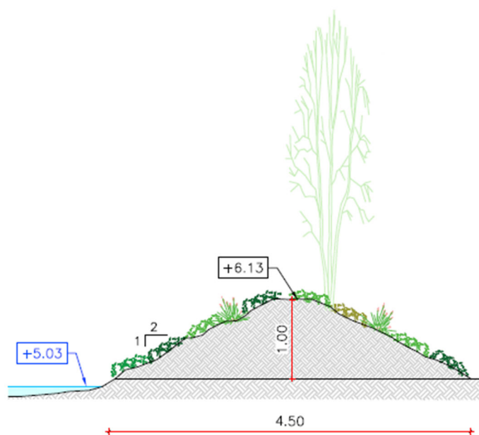
Figura 14. Secció perimetral, mota tipus D. Costat Nord.
