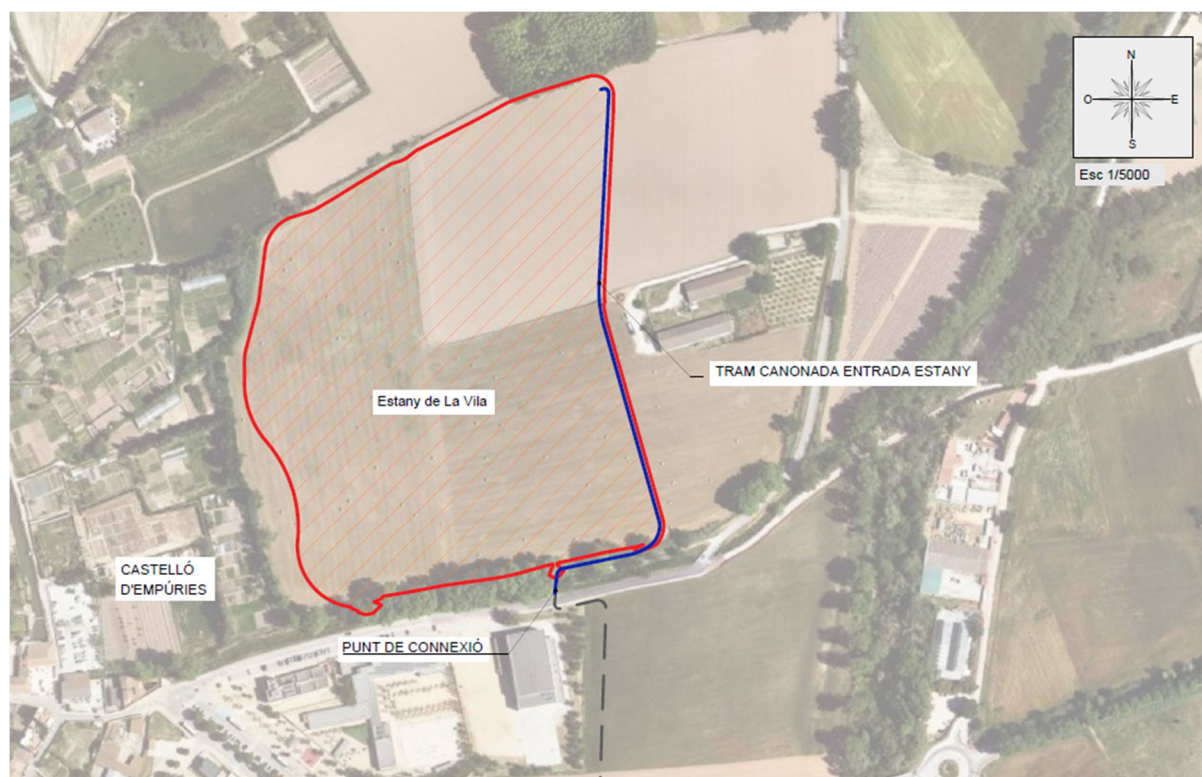
Figura 7. Àmbit de l'actuació i nou tram de canonada d'entrada a l'Estany des del punt de connexió
