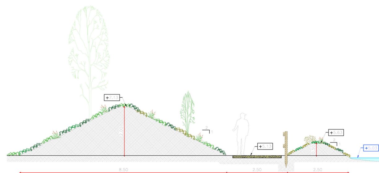
Figura 5. Secció tipus del perímetre de l'Estany en la seva part visitable
