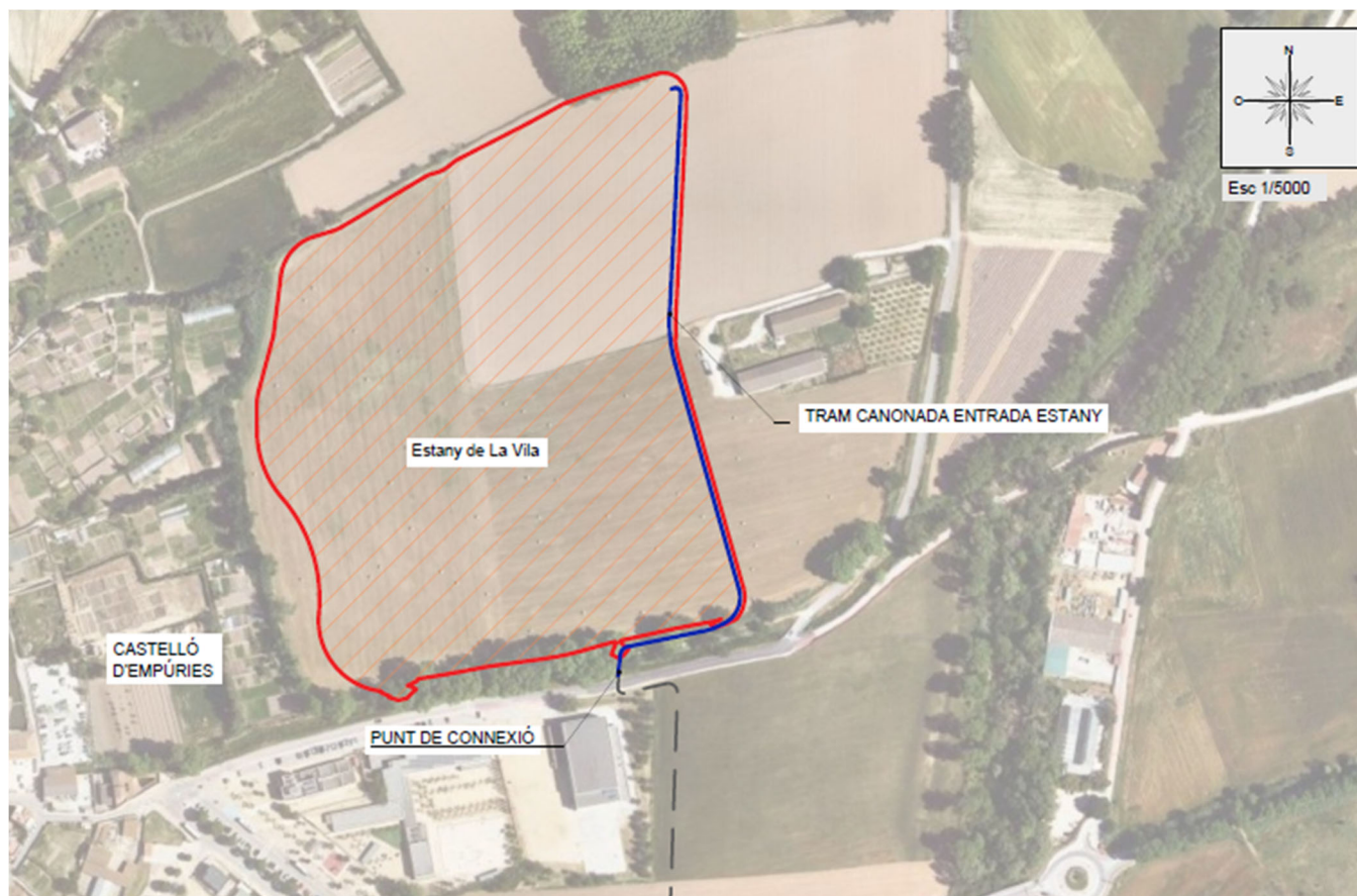
Figura 3. Àmbit de l'actuació i nou tram de canonada d'entrada a l'Estany des del punt de connexió
