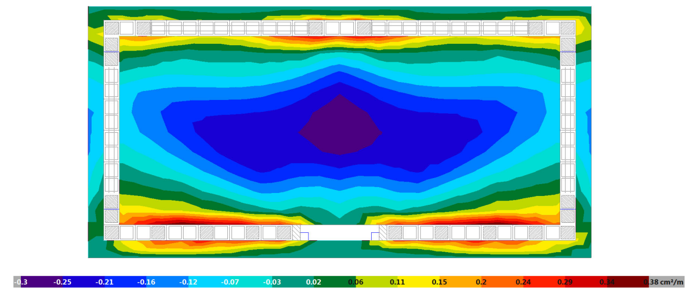
Figura 10. Quantia mínima necessària en Y inferior
