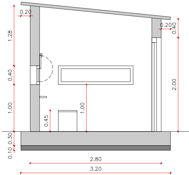
Secció transversal
