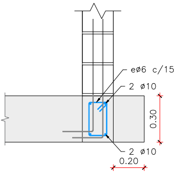
DETALL BIGA PERIMETRAL Esc 1/25
