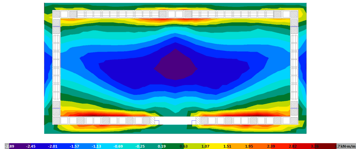
Figura 4. Moment Y inferior
