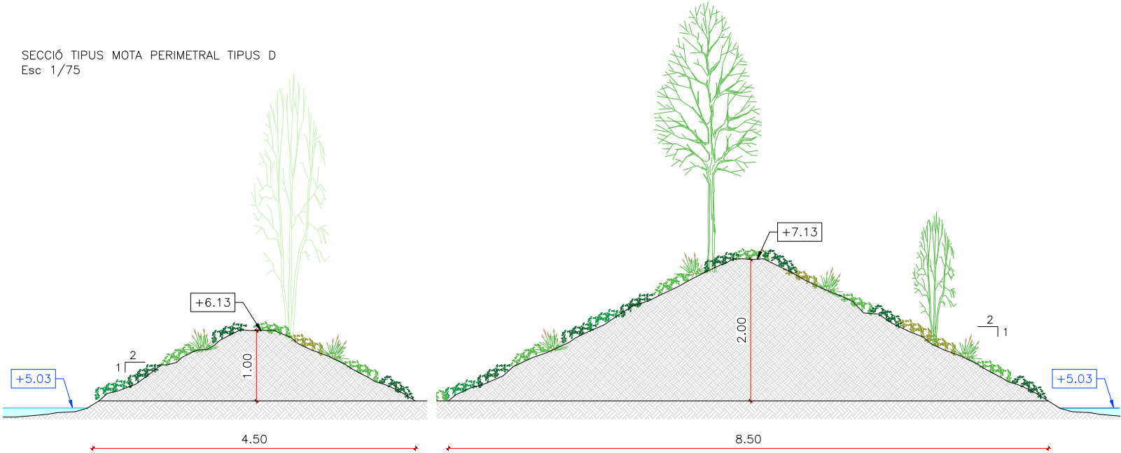
SECCIÓ TIPUS MOTA PERIMETRAL TIPUS E Esc 1/75
