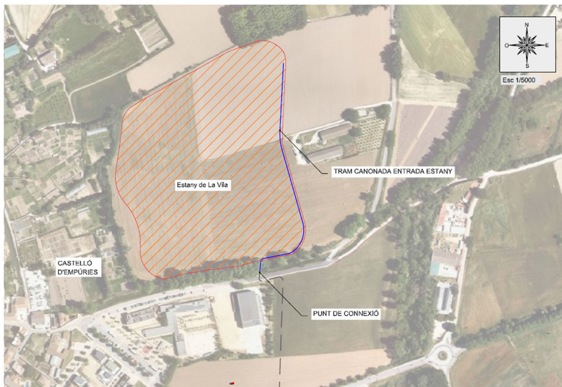
Figura 1. Àmbit de l'actuació i nou tram de canonada d'entrada a l'Estany de la Vila des del punt de connexió
