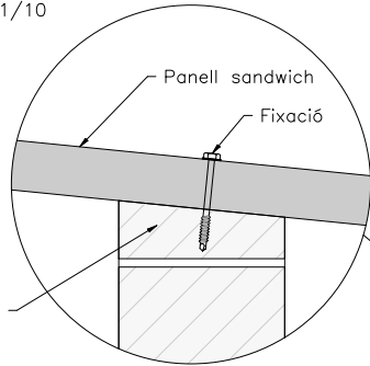
DETALL FIXACIÓ Esc 1/10
