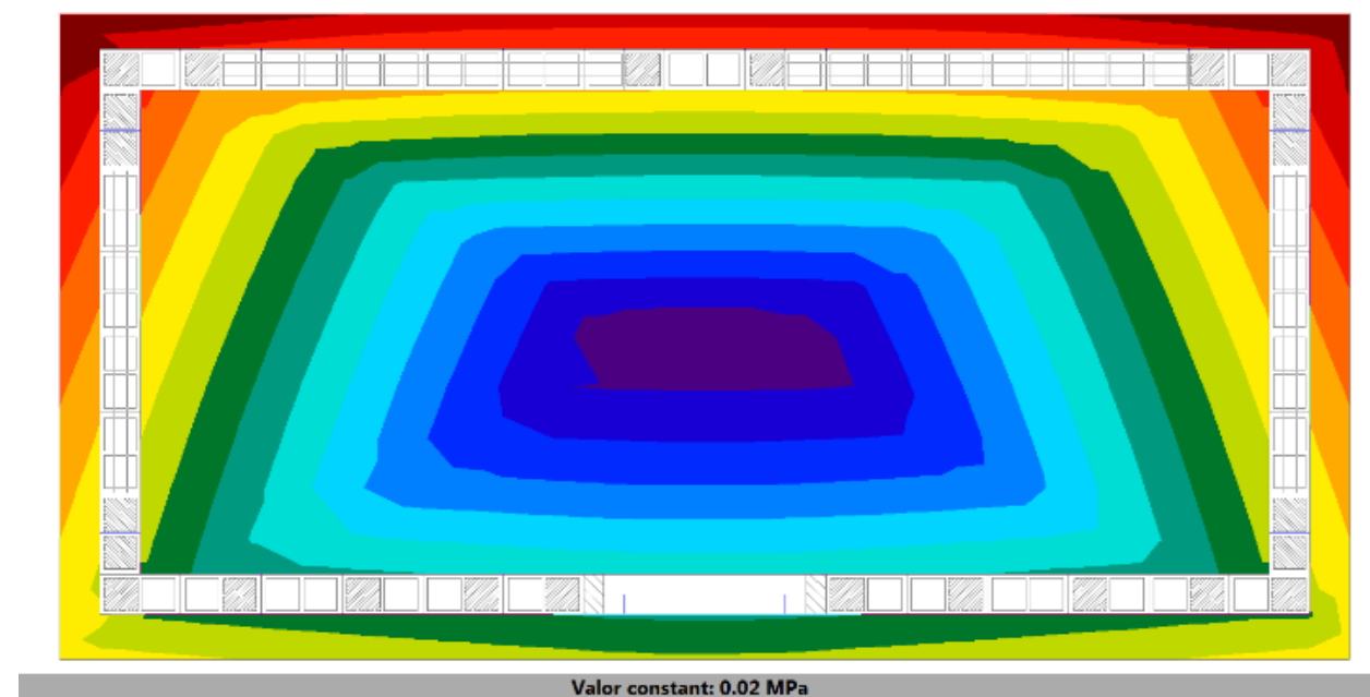
Figura 2. Tensions màximes sobre el terreny
