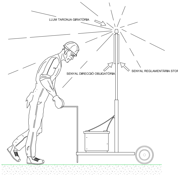
VISTA LATERAL
