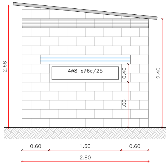
Mur 2
