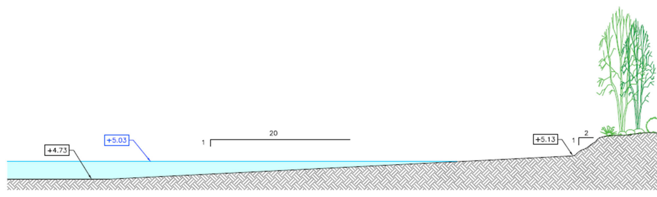
Figura 6. Detall secció tipus illa interior
