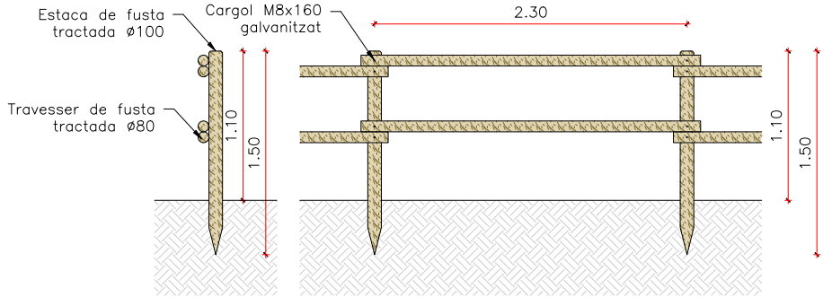
DETALL TANCA DE FUSTA TEXANA Esc 1/50
