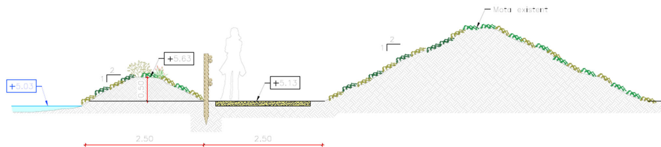
Figura 9. Secció tipus mota perimetral tipus A. Costat Sud.
