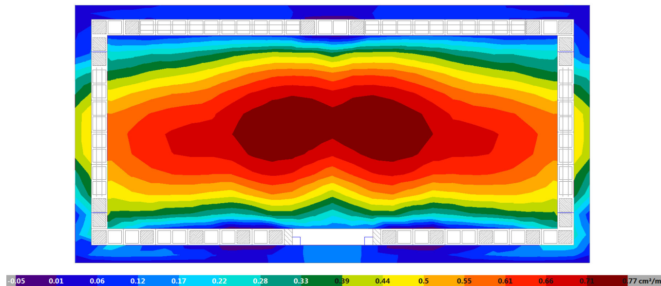
Figura 12. Quantia mínima necessària en Y superior
