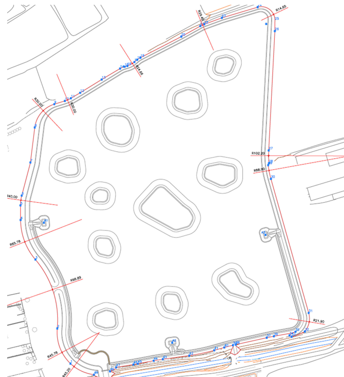
Figura 2. Eix de replanteig Estany de la Vila
