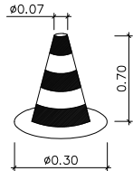
CON DE BALISAMENT DETALL 010105
