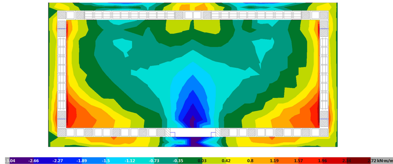
Figura 3. Moment X inferior
