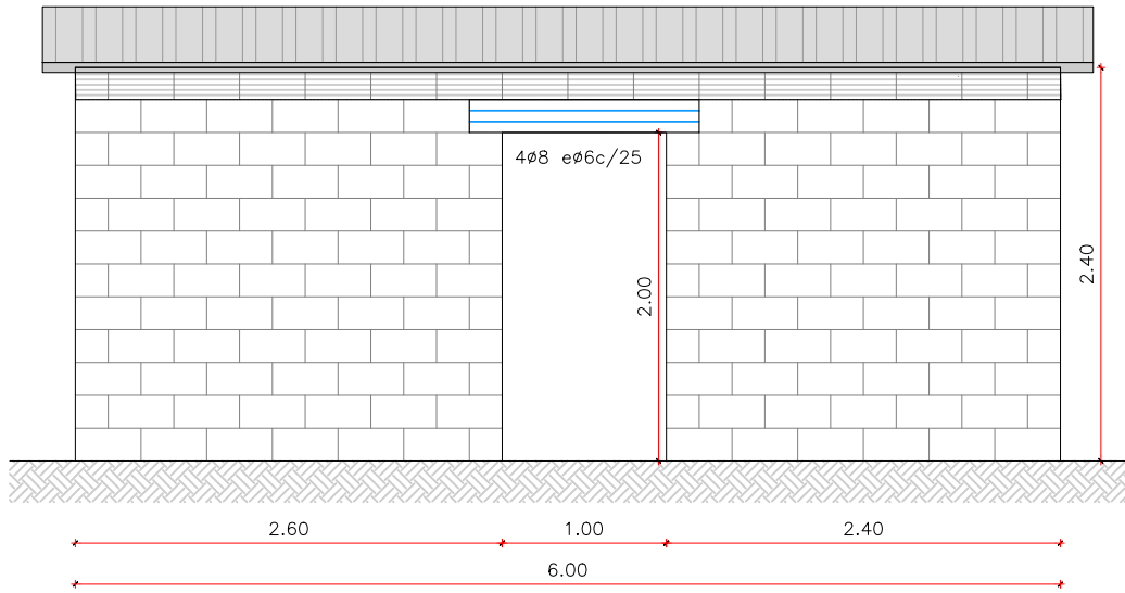
Mur 1
