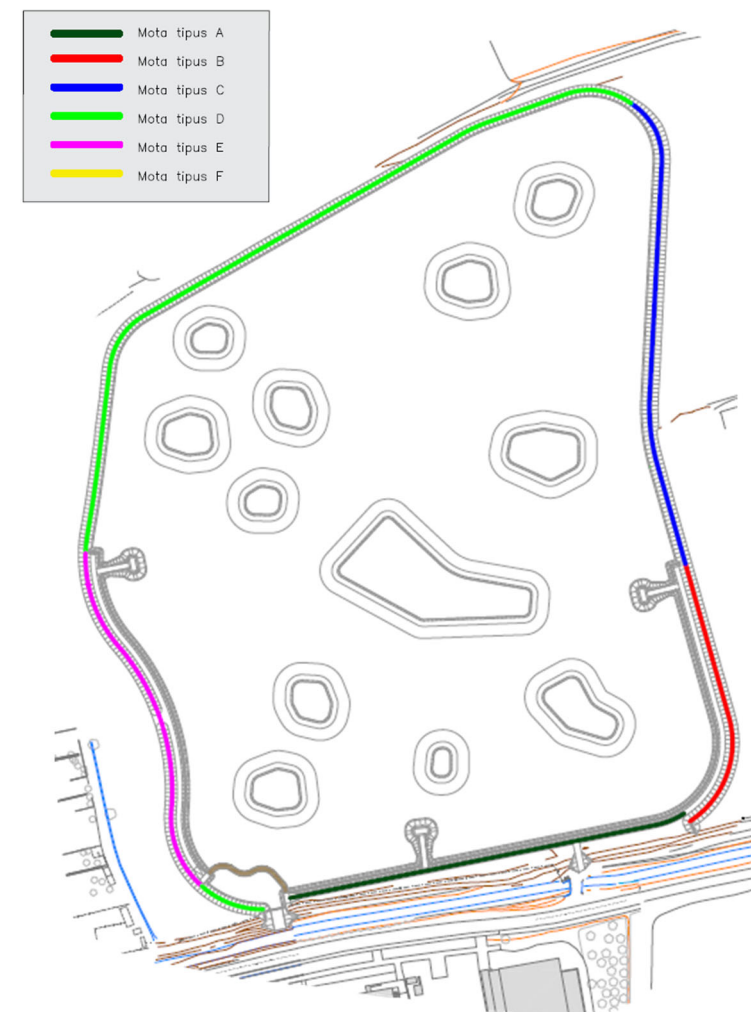
Figura 15. Tipologia de seccions de motes perimetrals
