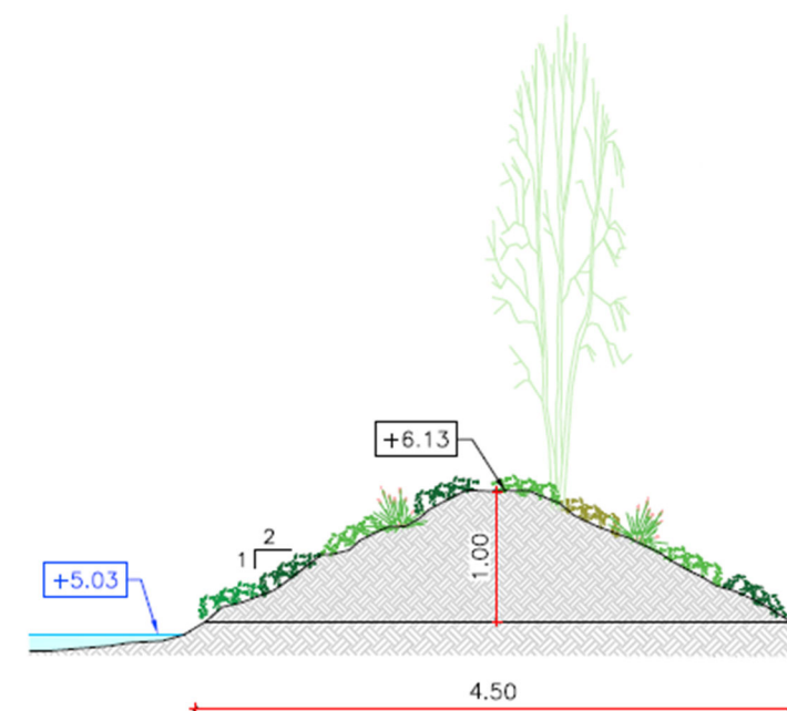
Figura 12. Secció perimetral, mota tipus D. Costat Nord.
