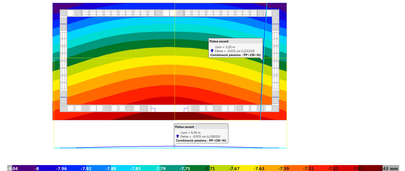
Figura 13. Desplaçaments llosa fonamentació
