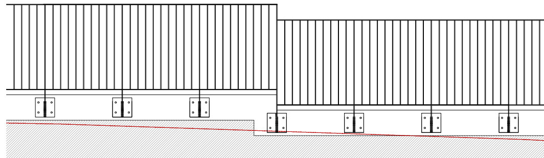
Alçat de barana en punts singulars de canvis de nivell: 1/50
