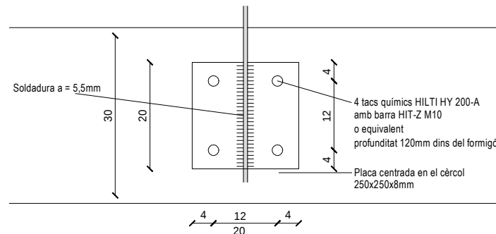
Detall ancoratge barana al cèrcol de formigó: 1/10
