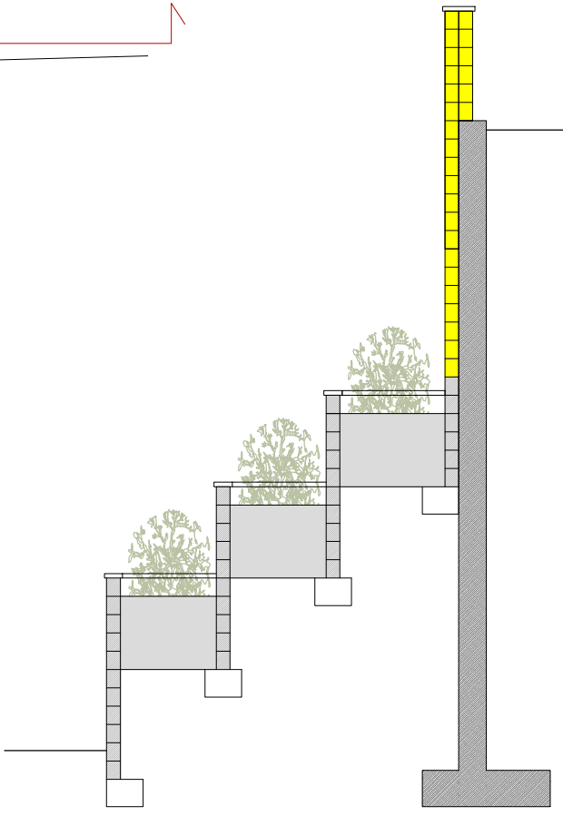
Secció C-C' enderroc: 1/75
