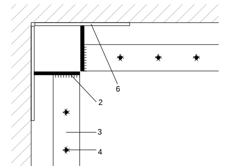
Detall en planta de la barana en cantonada: 1/10
