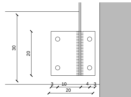
Detall ancoratge a l'extrem del mur: 1/10
