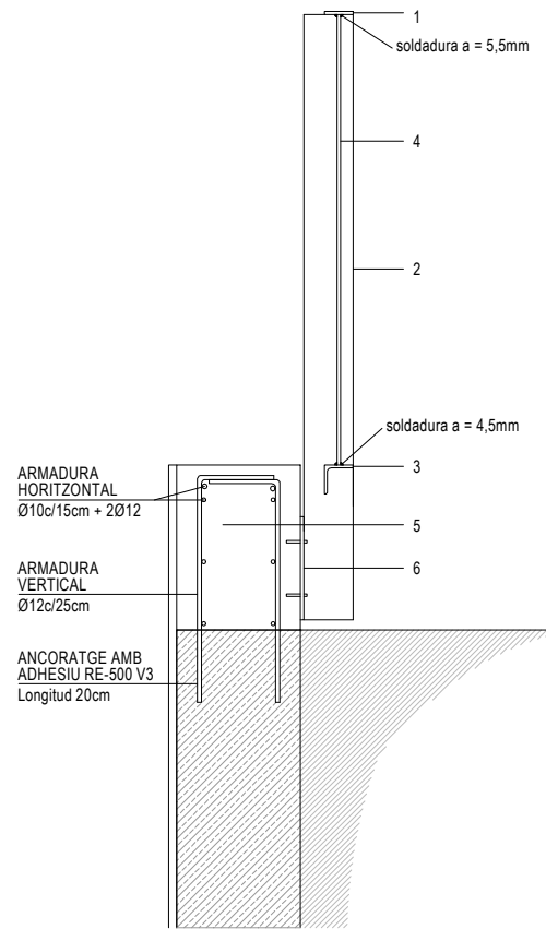
Secció: 1/20
