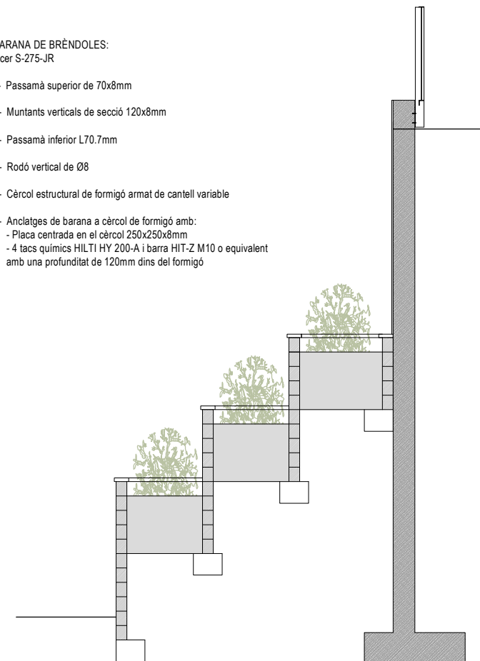
Secció A-A' proposa: 1/75
