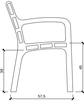
nota: els tractaments anti-graffiti i anti-envelliment de les fustes s'aplicaran a taller BANC FUSTA AMB RESPALLERS I RECOLZA-BRAÇOS DE 150cm Esc.: 1/10 (cotes en cm)
