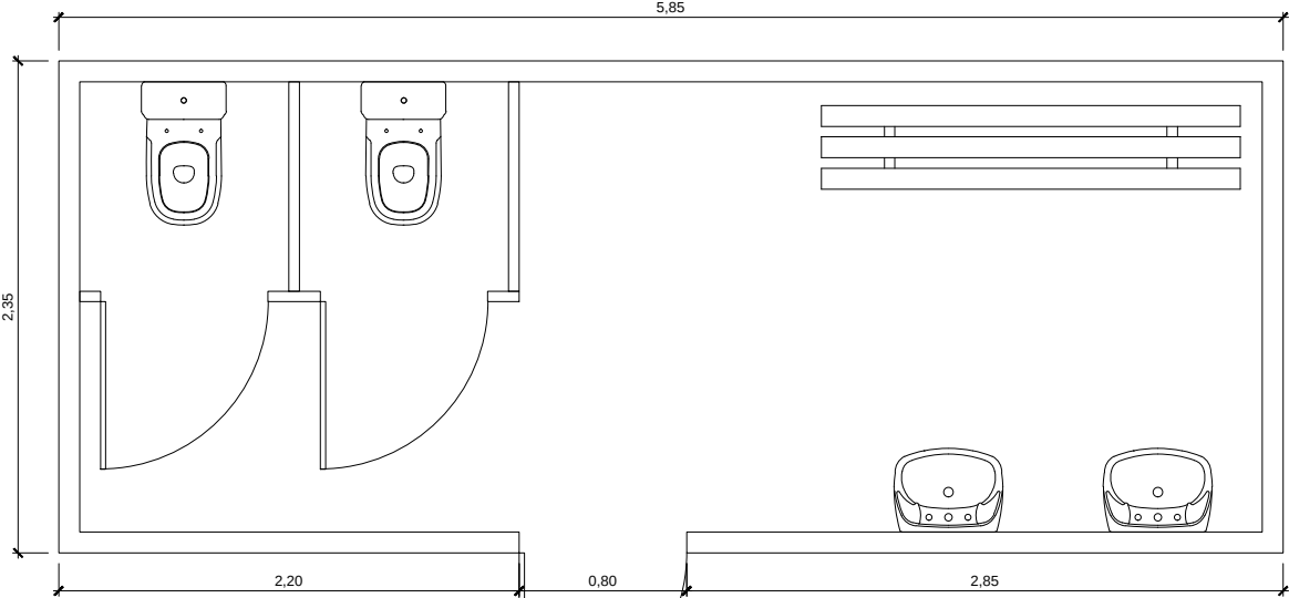
MÒDUL VESTUARI DE 585x235cm Esc.: 1/10 (cotes en cm)
