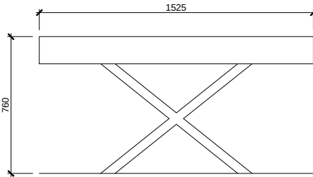
ALÇAT FRONTAL
