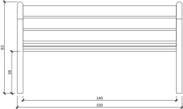
nota: els tractaments anti-graffiti i anti-envelliment de les fustes s'aplicaran a taller BANC FUSTA AMB RESPALLERS I RECOLZA-BRAÇOS DE 150cm Esc.: 1/10 (cotes en cm)
