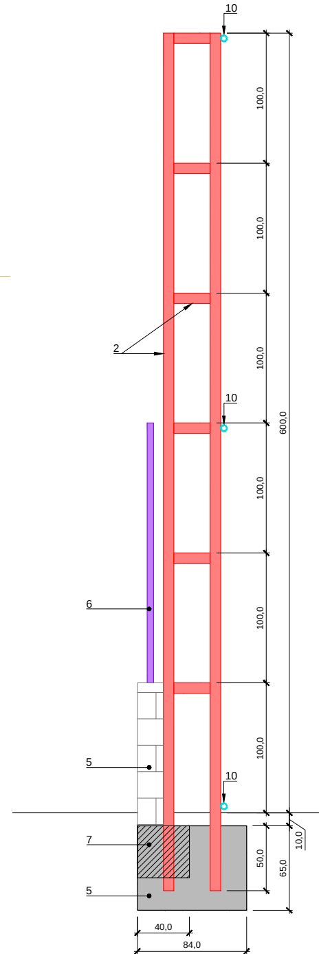
SECCIÓ TIPUS ESTRUCTURA esc.: 1/20 (cotes en cm)
