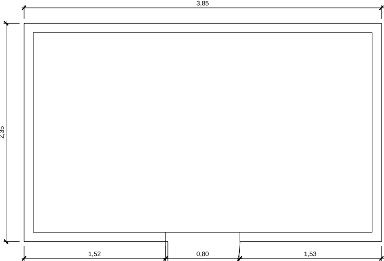
MÒDUL MAGATZEM MITJA DE 385x235cm Esc.: 1/10 (cotes en cm)
