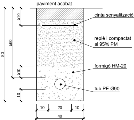
DETALL RASA Esc.: 1/10 (cotes en mm)
