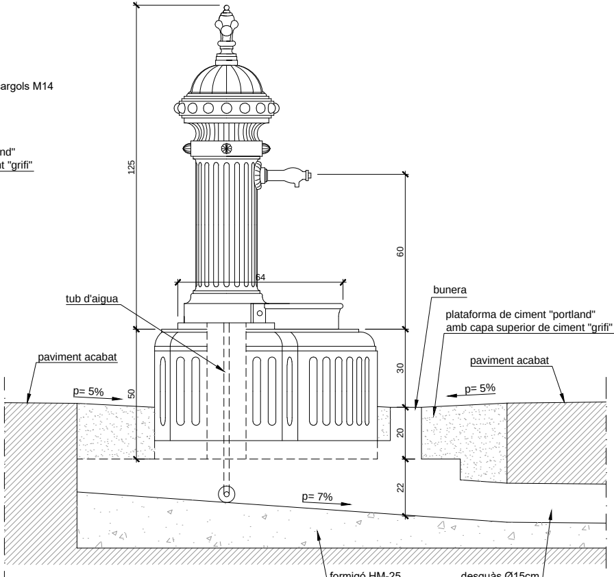
SECCIÓ
