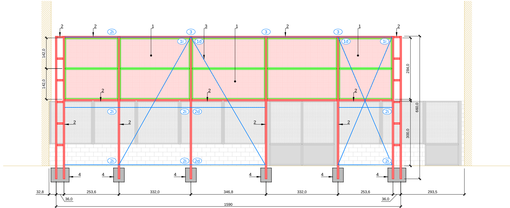
ALÇAT A esc.: 1/50 (cotes en cm)
