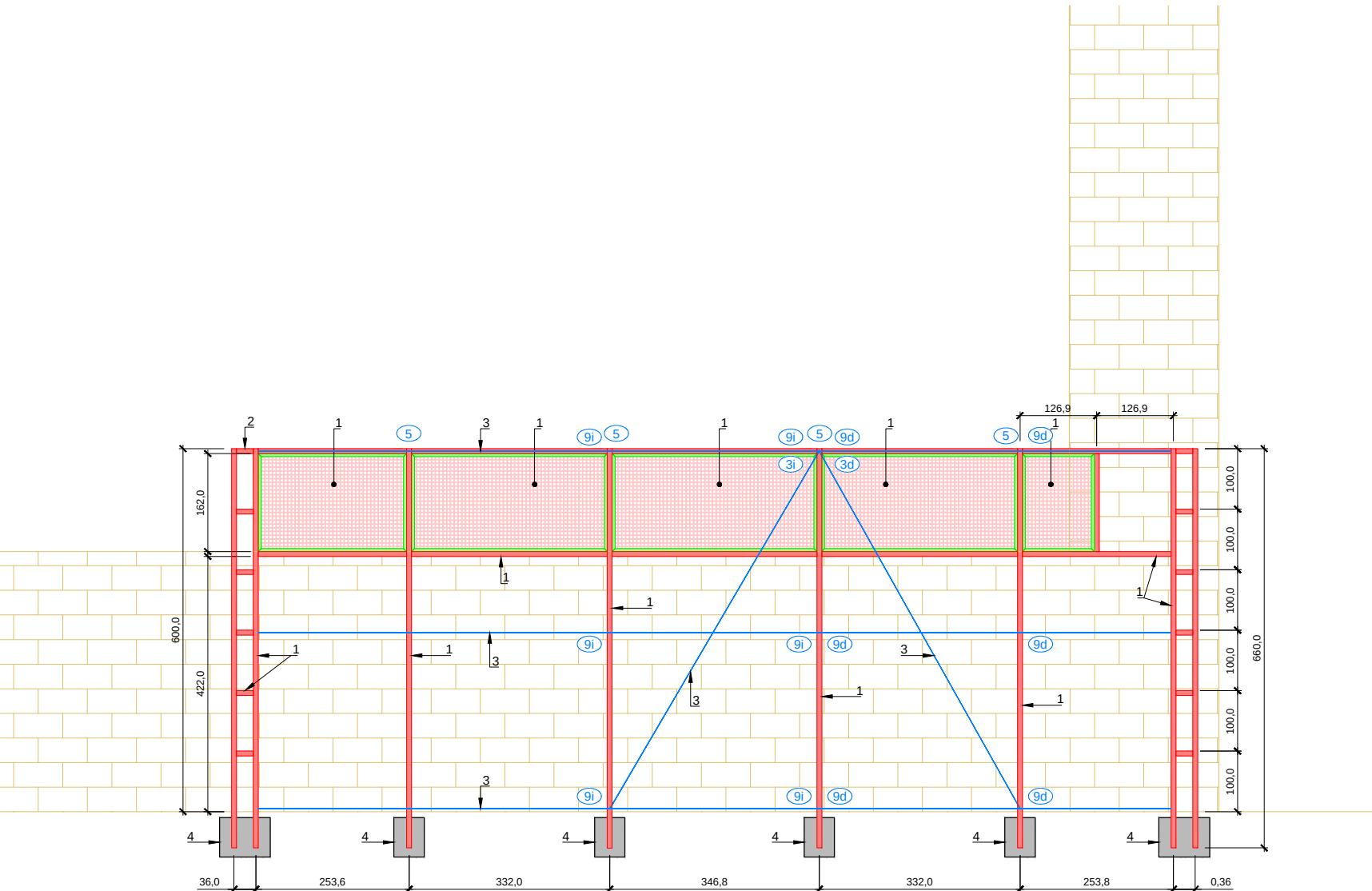
ALÇAT B esc.: 1/50 (cotes en cm)
