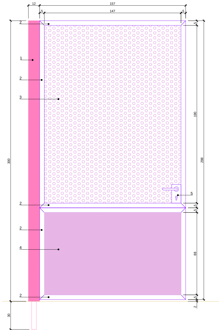
ALÇAT
