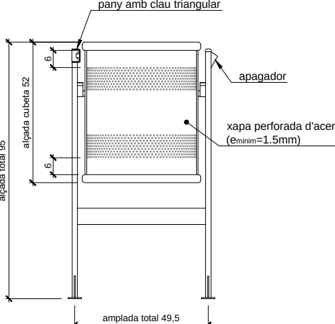
ALÇAT
