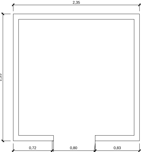
MÒDUL MAGATZEM PETIT DE 235x235cm Esc.: 1/10 (cotes en cm)
