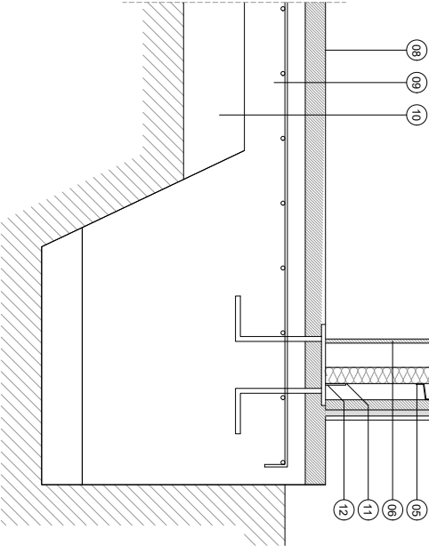
SECCIO VERTICAL, TIPUS E:1/10
