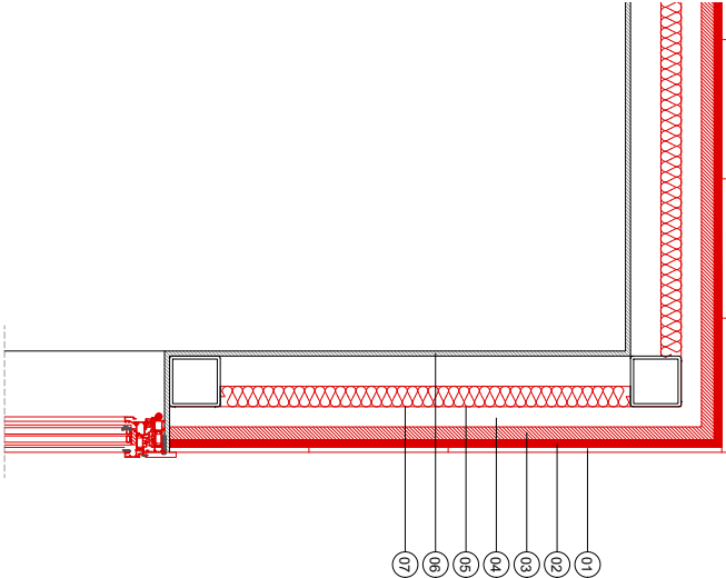
SECCIO HORIZONTAL, TIPUS E:1/10
