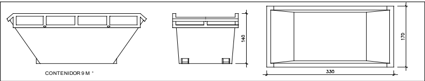
CONTENIDOR 9 M 3
