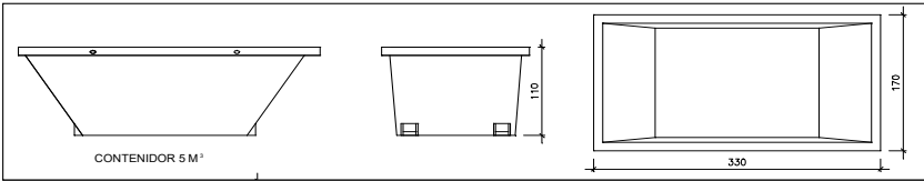
CONTENIDOR 5 M 3
