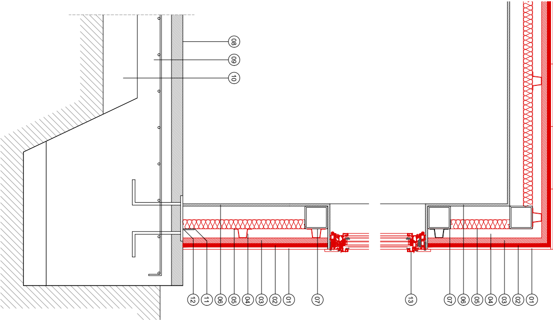
SECCIO VERTICAL, TIPUS E:1/10
