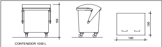
CONTENIDOR 1000 L
