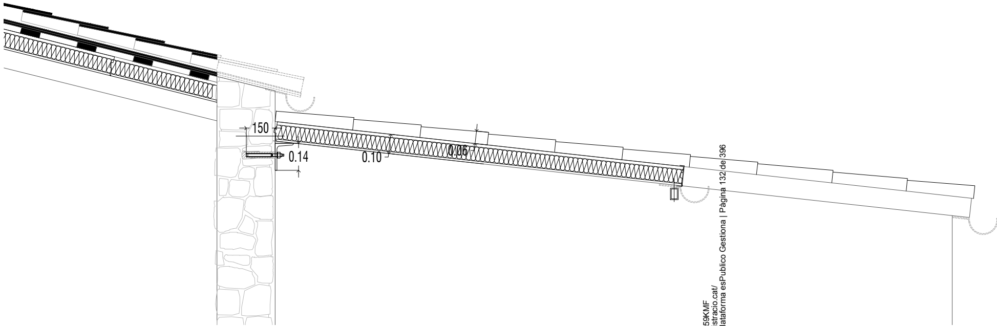
SECCIÓ CONSTRUCTIVA- NOVA COBERTA ZONA RENTADOR I AÏLLAMENT A COBERTA PRINCIPAL
