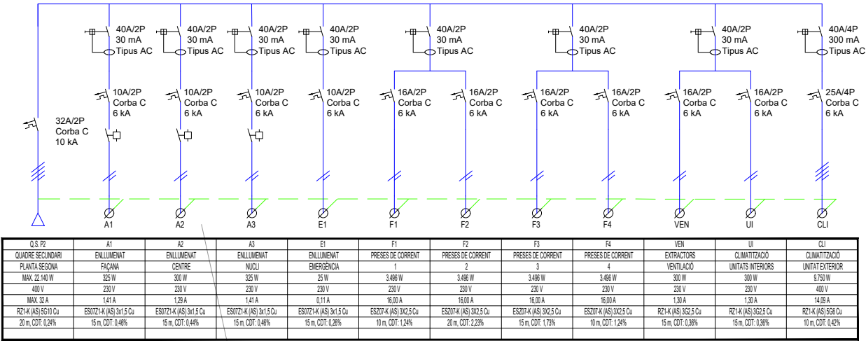
QUADRE SECUNDARI DE PLANTA 2 (Q.S. P2)
