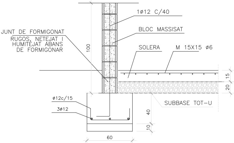
DETALL PARET DE CARGA
