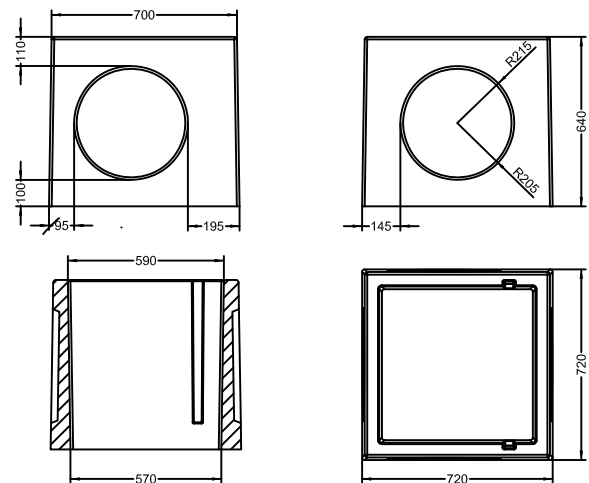
ARQUETA 60X60CM
