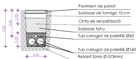
DETALL RASA 2Ø160 + 1Ø63 - AMB ACABAT AMB PANOT
