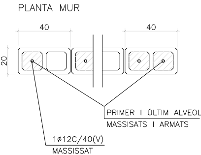
DETALL PARET DE CARGA
