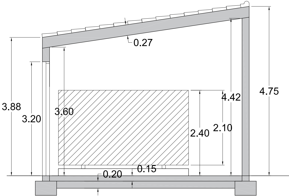
SECCIÓ
