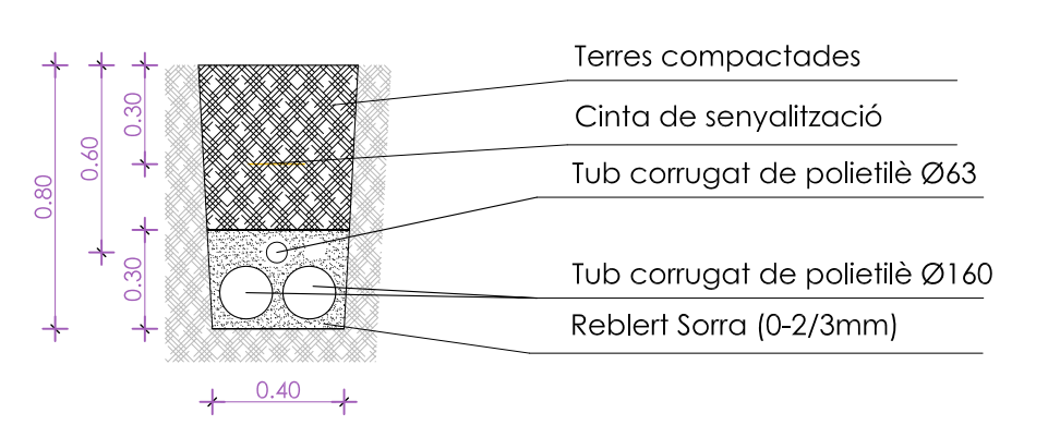
DETALL RASA 2Ø160 + 1Ø63 - AMB ACABAT DE TERRES
