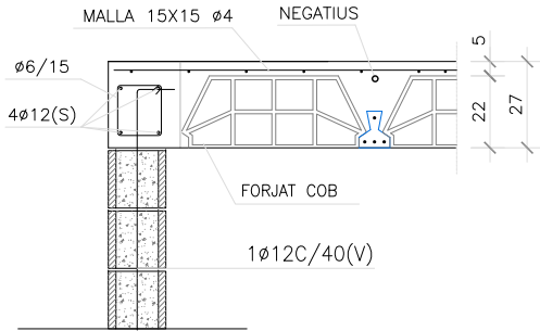
DETALL FORJAT UNIDIRECCIONAL
