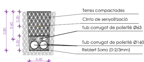
DETALL RASA 2Ø160 + 1Ø63 - AMB ACABAT DE TERRES
