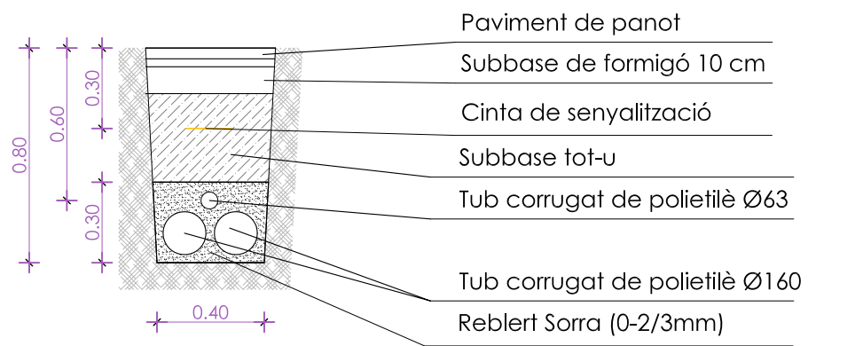
DETALL RASA 2Ø160 + 1Ø63 - AMB ACABAT AMB PANOT
