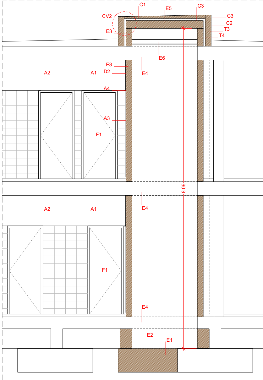
SECCIÓ T2
