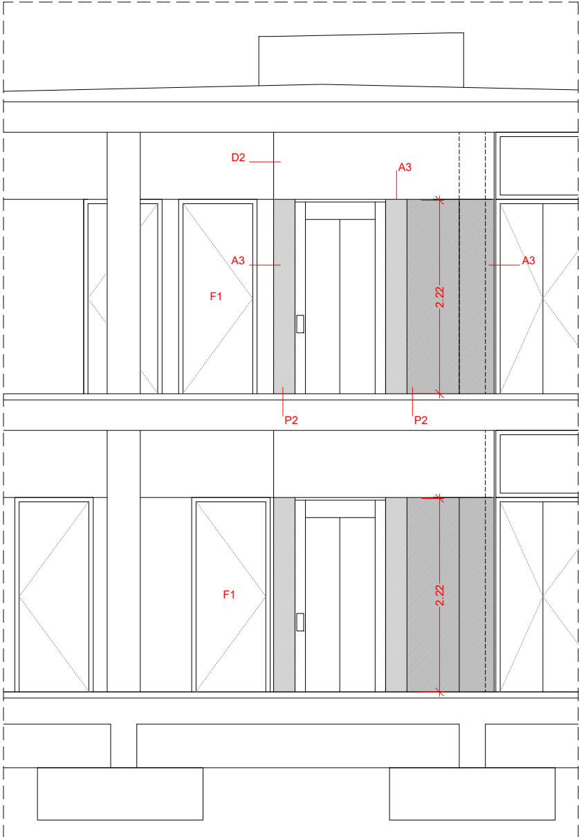
SECCIÓ T1
