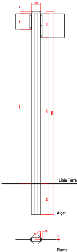
Banderola ref: D 26Q Escala= 1/5 - Imprès a Din A3
