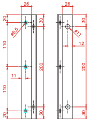
Detall dels angles de banderola per suports de fusta Ø100 mm.
