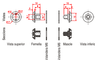
Detall cargols especial, Escala = 1/2 - Imprès a Din A3 Cargols de llautó mecanitzats M6
