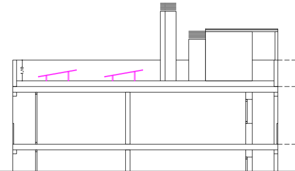
DETALL SECCIÓ TRANSVERSAL COBERTA PLANTA SISENA
