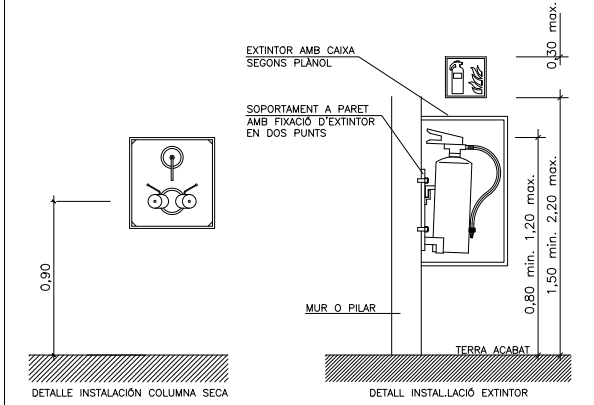
DETALL UBICACIÓ EXTINTORS I COLUMNA SECA EN PARET
