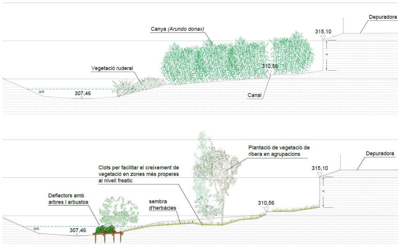
Figura 8 Comparació de secció tipus de l'estat actual (superior) i futur (inferior)
