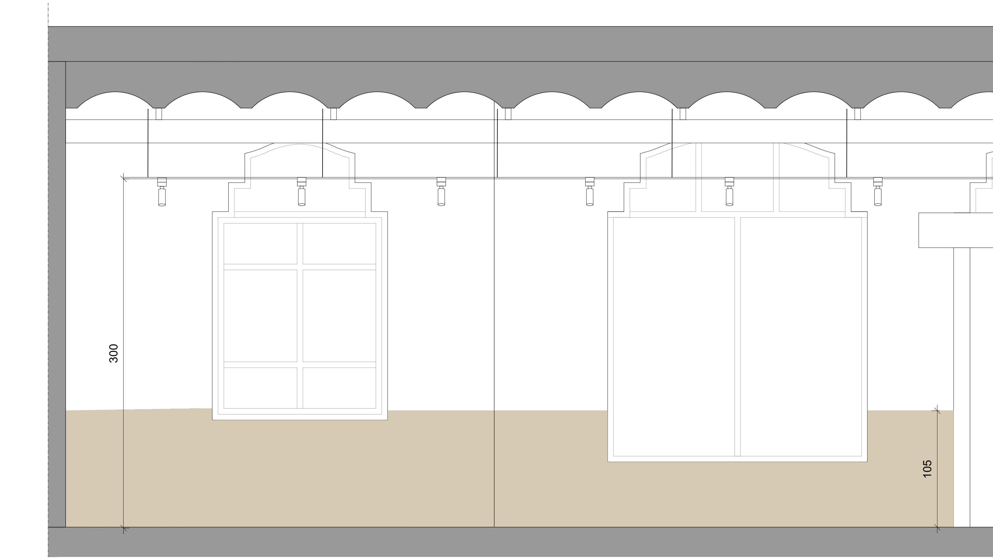
ALÇAT CC' R2 e 1/20. L=14,75 ml
