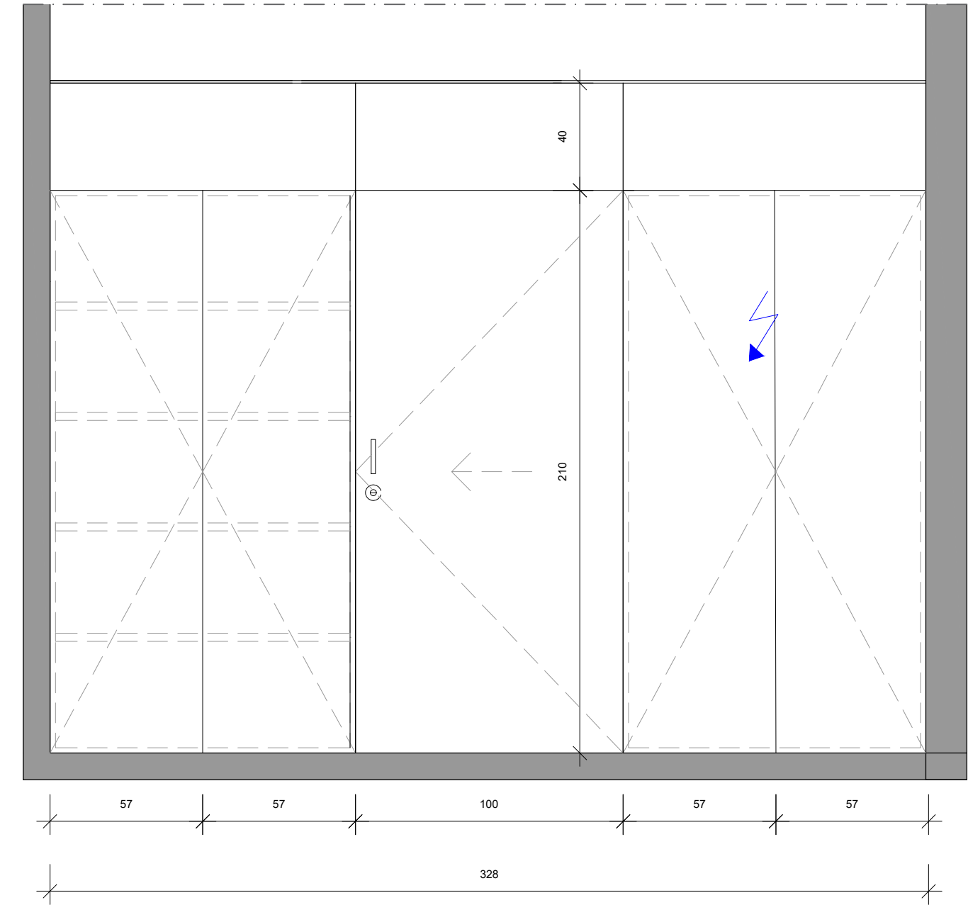
A-A' SECCIÓ GENERAL E 1:20
