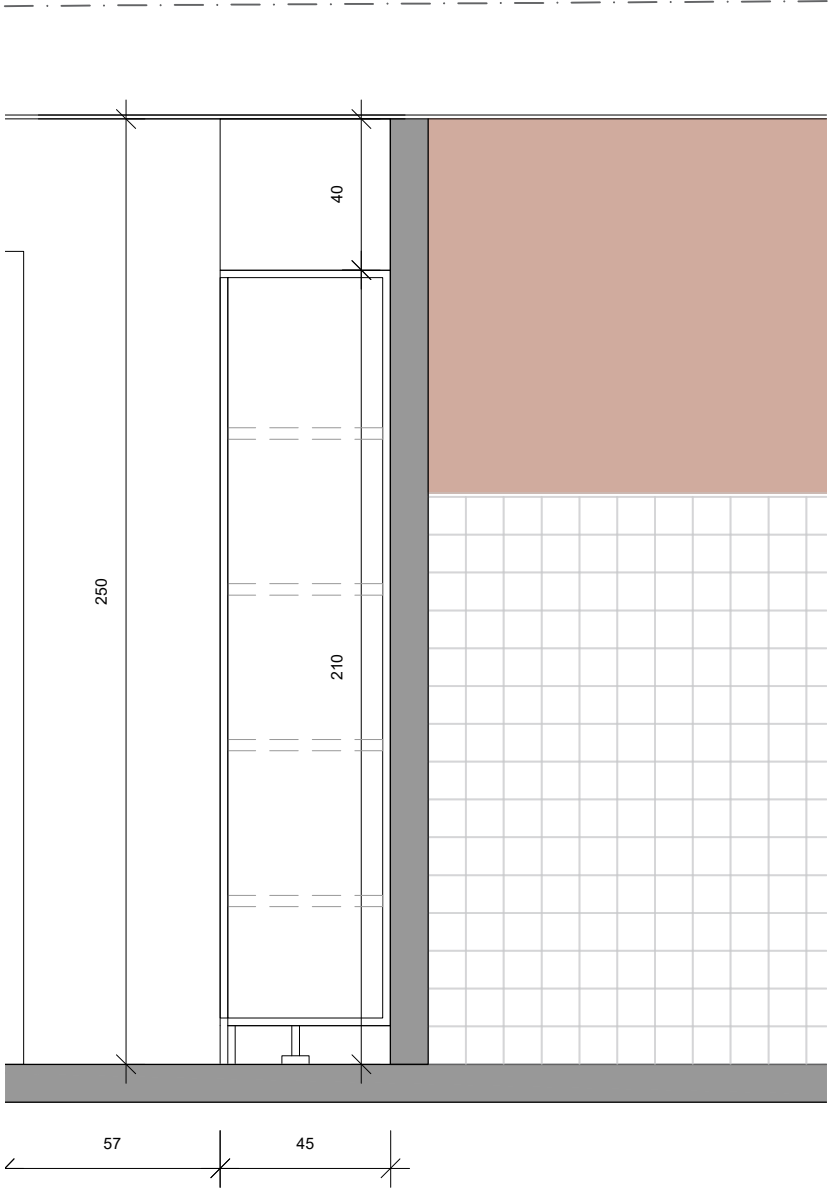
B-B' SECCIÓ GENERAL E 1:20
