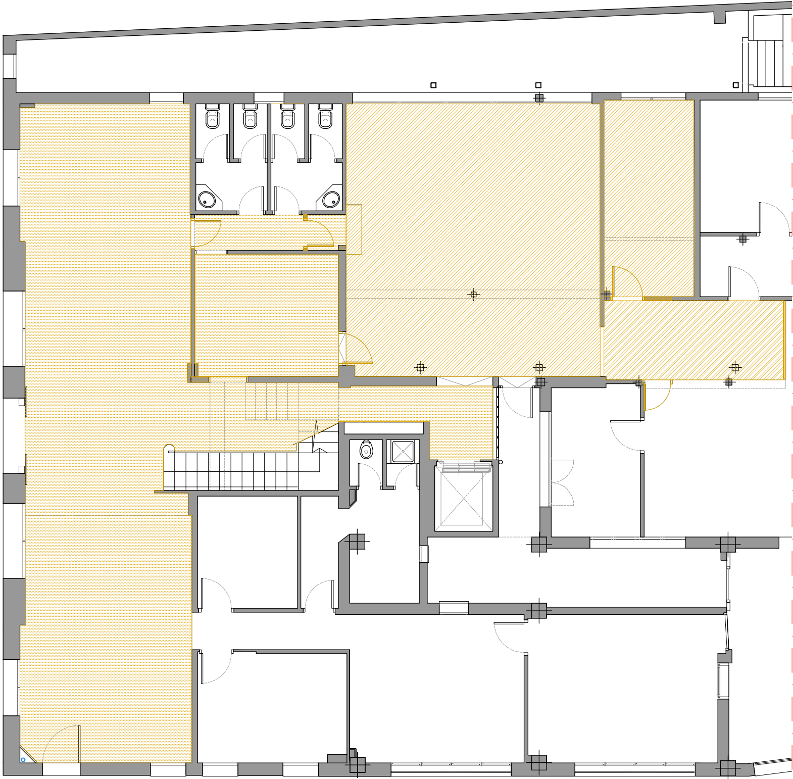
PLANTA ENDERROCS
