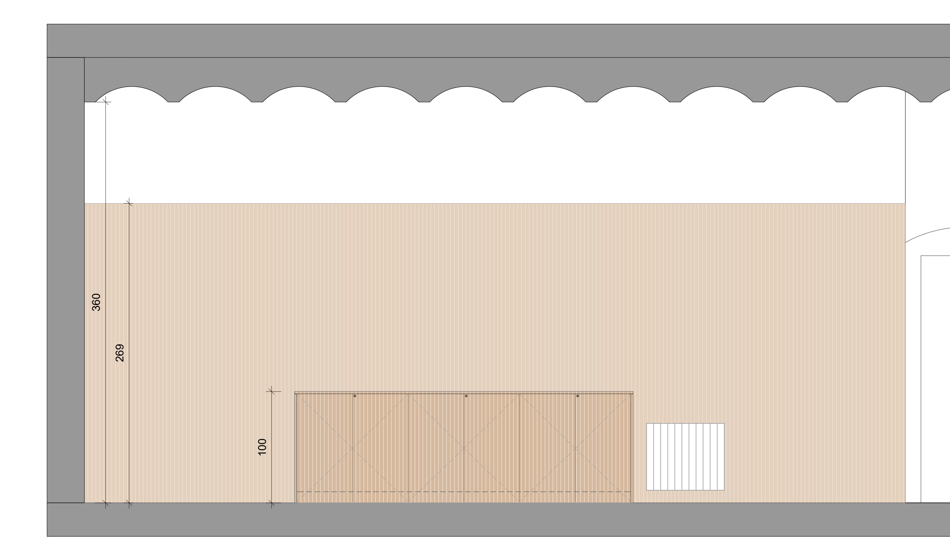
ALÇAT AA' R1 e 1/20. L=10 ml
