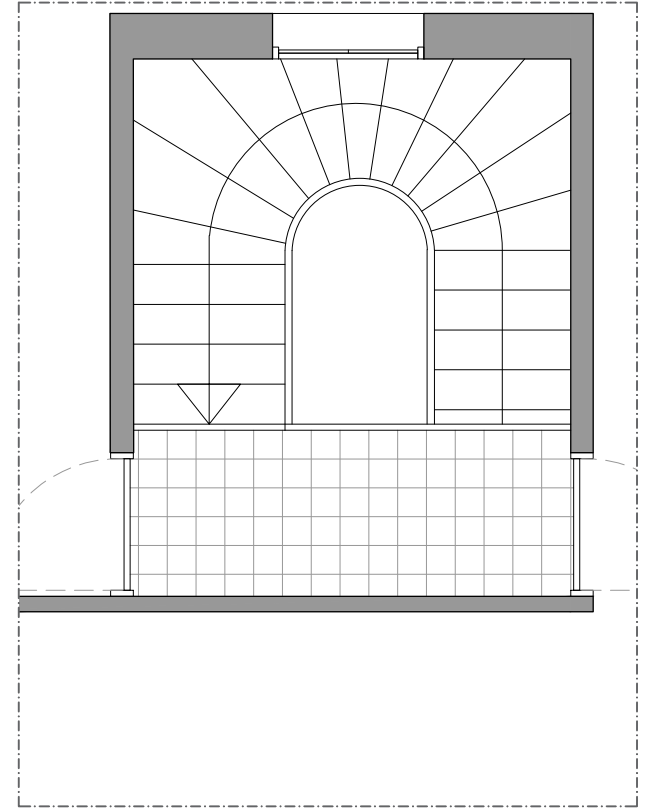
P2 PLANTA
