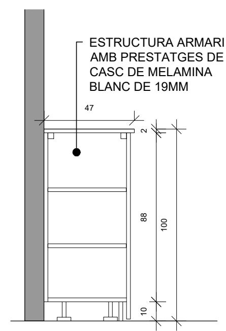
SECCIÓ
