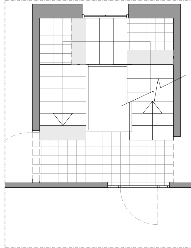
P1 PLANTA
