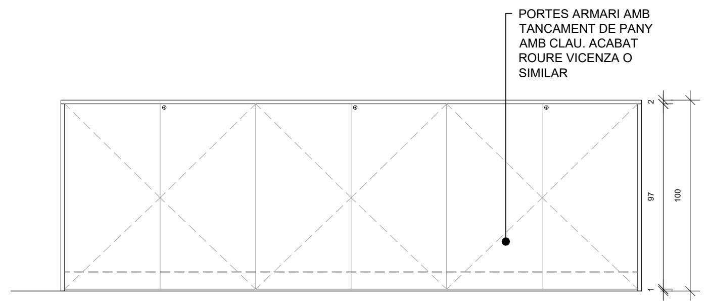
ALÇAT
