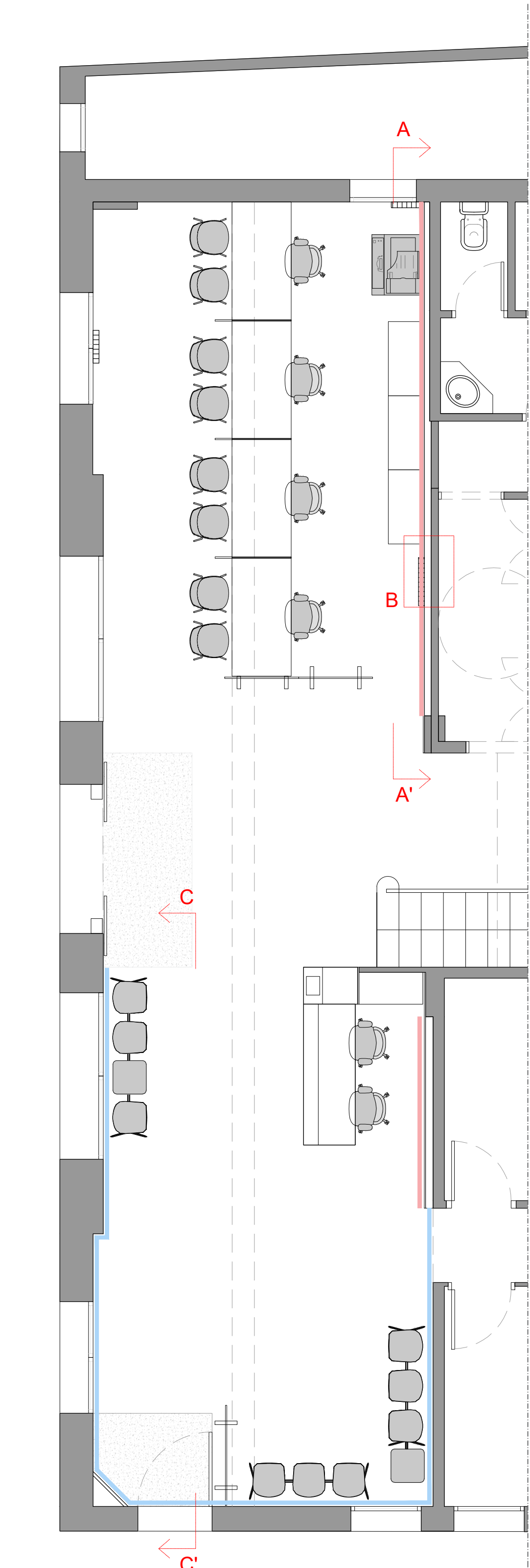
PLANTA 1/50
