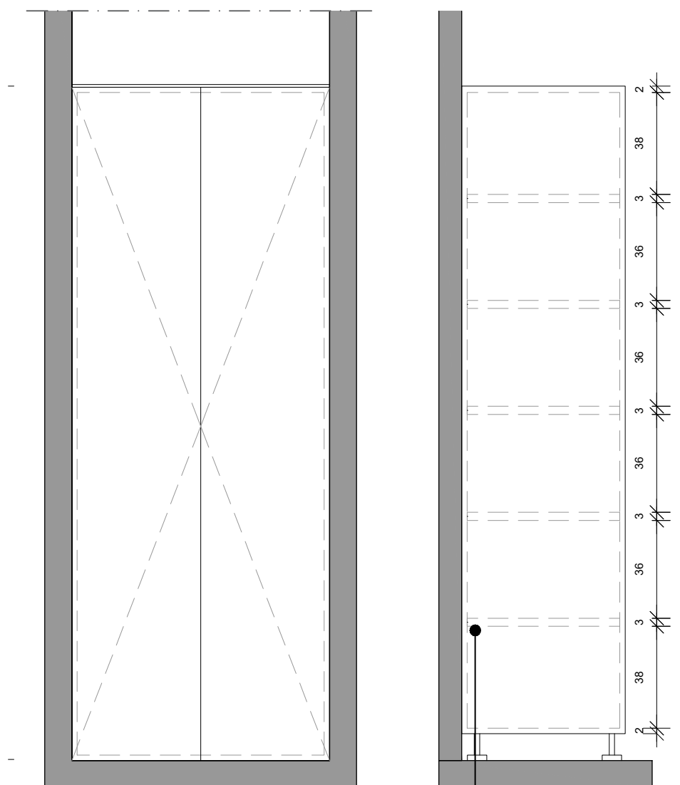
ALÇAT
