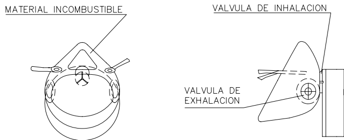
SECCION A-A
