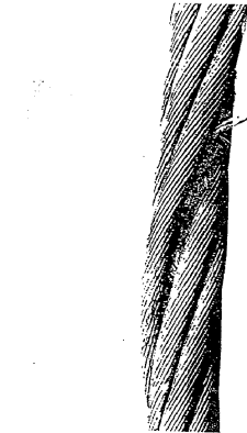
Cliché 14 - Aumento local del diámetro del cable debido a la humedad del alma textil que aparece desgranada entre los cordones. El cable debe ser retirado.
