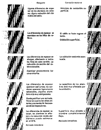
Cliché 4 - Ejemplos de la progresión del desgaste y la corrosión externa de un cable cruzado.
