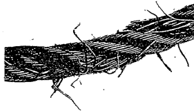
Cliché 21 - Ejemplo de un cable salido de una garganta de pólea y atascado. Esto ha producido una deformación y rotura de alfileres así como la rotura parcial de cordones. El cable debe ser retirado inmediatamente.
