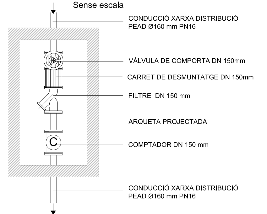
DETALL MUNTATGE COMPTADOR A LA SORTIDA DEL DIPÒSIT EN CONDUCCIÓ DE DISTRIBUCIÓ PEAD Ø160 mm PN16 PROJECTADA Sense escala
