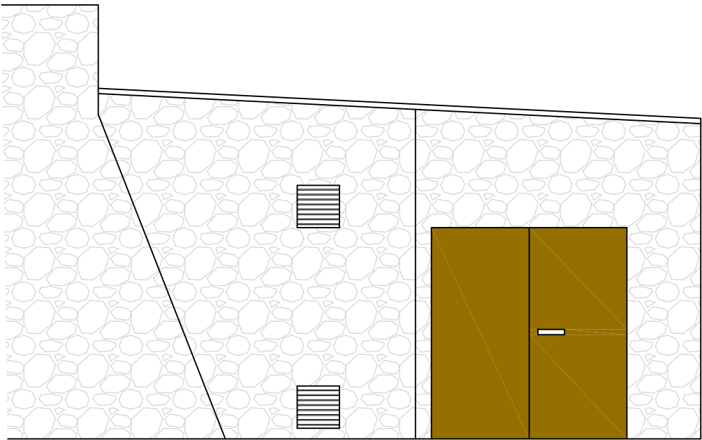
ALÇAT SUD-OEST
