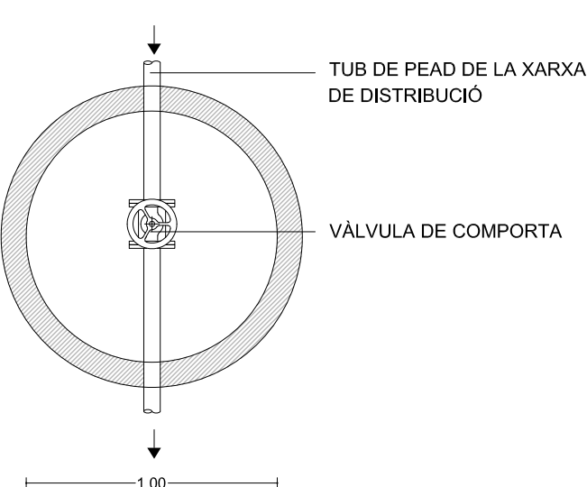
DETALL DE PLANTA DE PERICÓ DE VÀLVULA DE COMPORTA DE SECCIONAMENT PER A TUB PEAD Sense escala
