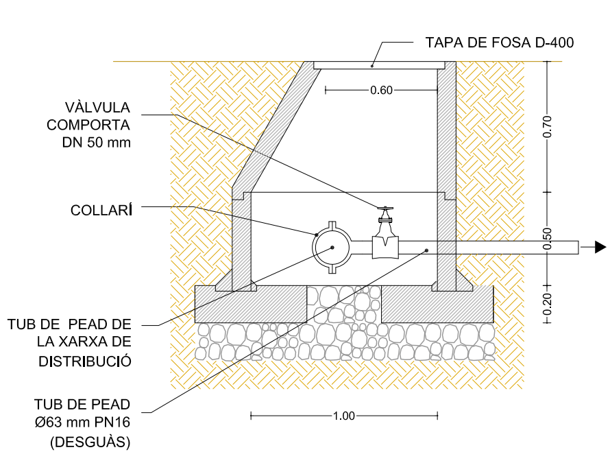
DETALL DE SECCIÓ DE PERICÓ DE DESGUÀS DE CONDUCCIÓ DE REG Sense escala
