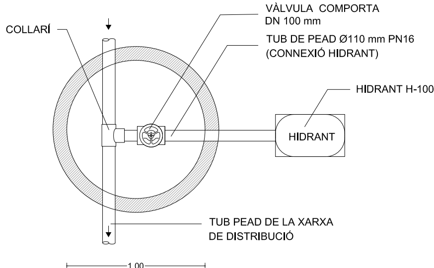
DETALL DE PLANTA DE PERICÓ DE VÀLVULA DE SECCIONAMENT D'HIDRANT Sense escala
