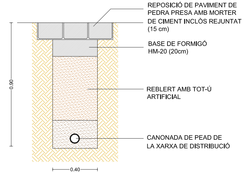
RASA TIPUS PAS CONDUCCIÓ PER TRAMS DE VIAL AMB PAVIMENT DE PEDRA Sense escala
