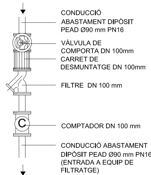
DETALL MUNTATGE COMPTADOR EN CONDUCCIÓ D'ABASTAMENT A L'ENTRADA DEL DIPÒSIT Sense escala
