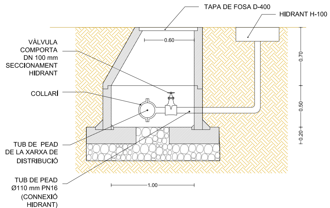
DETALL DE SECCIÓ DE PERICÓ DE VÀLVULA DE SECCIONAMENT D'HIDRANT Sense escala
