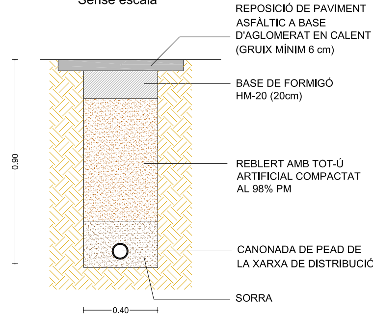
RASA TIPUS PER TRAMS DE DE VIAL AMB PAVIMENT ASFÀLTIC Sense escala
