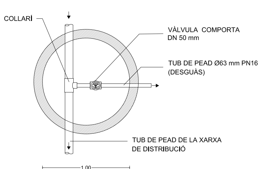
DETALL DE PLANTA DE PERICÓ DE DESGUÀS DE CONDUCCIÓ DE XARXA DE DISTRIBUCIÓ Sense escala
