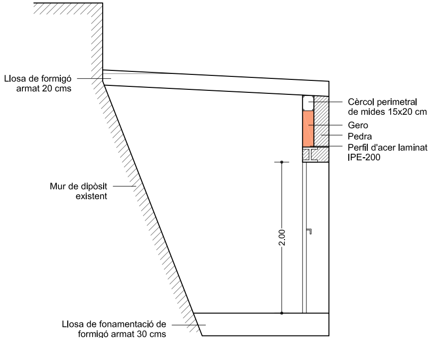
SECCIÓ A-A'
