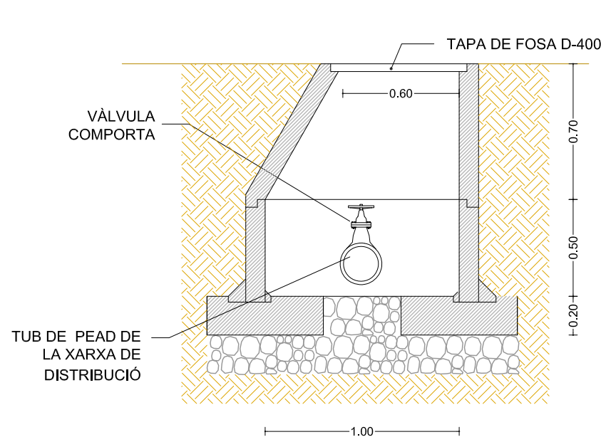
DETALL DE SECCIÓ DE PERICÓ DE VÀLVULA DE COMPORTA DE SECCIONAMENT PER A TUB DE PEAD Sense escala
