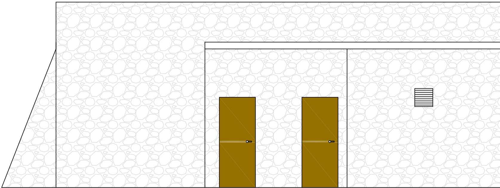
ALÇAT SUD-EST
