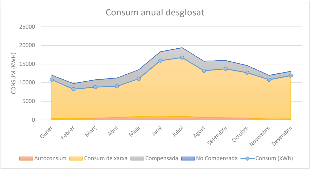
Figura 13 Distribució de l'energia per mesos
