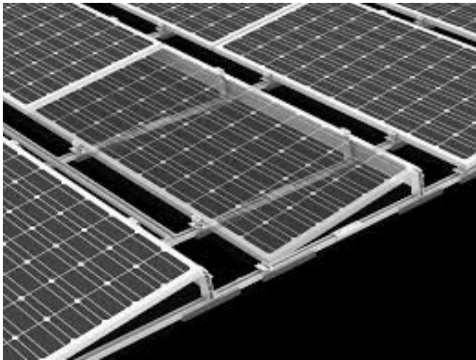
Figura 2.4 Detall de l'estructura de suport
