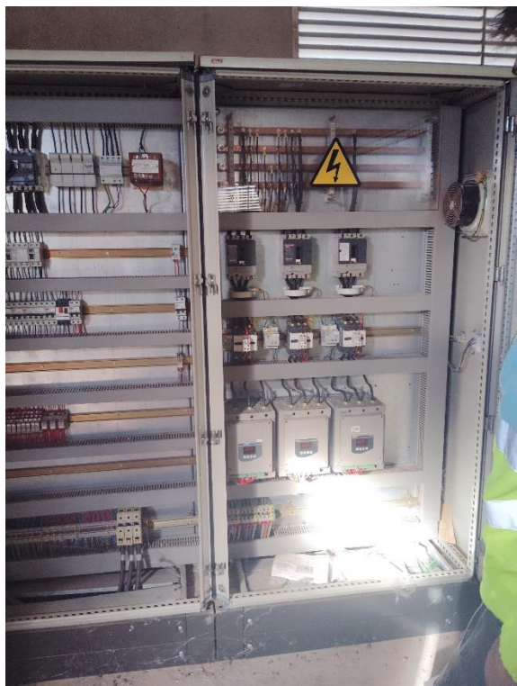
Figura 5. Interior del QGBT on s’instal·laran les proteccions de CA i es connectarà la instal·lació FV.
