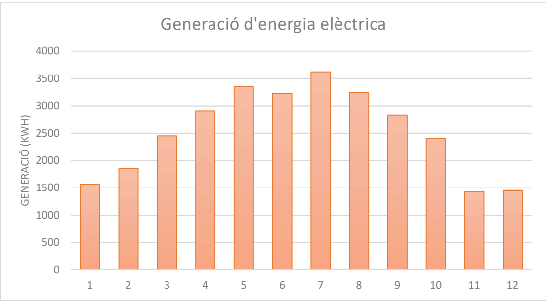
Figura 4.1 Generació mensual d'energia
