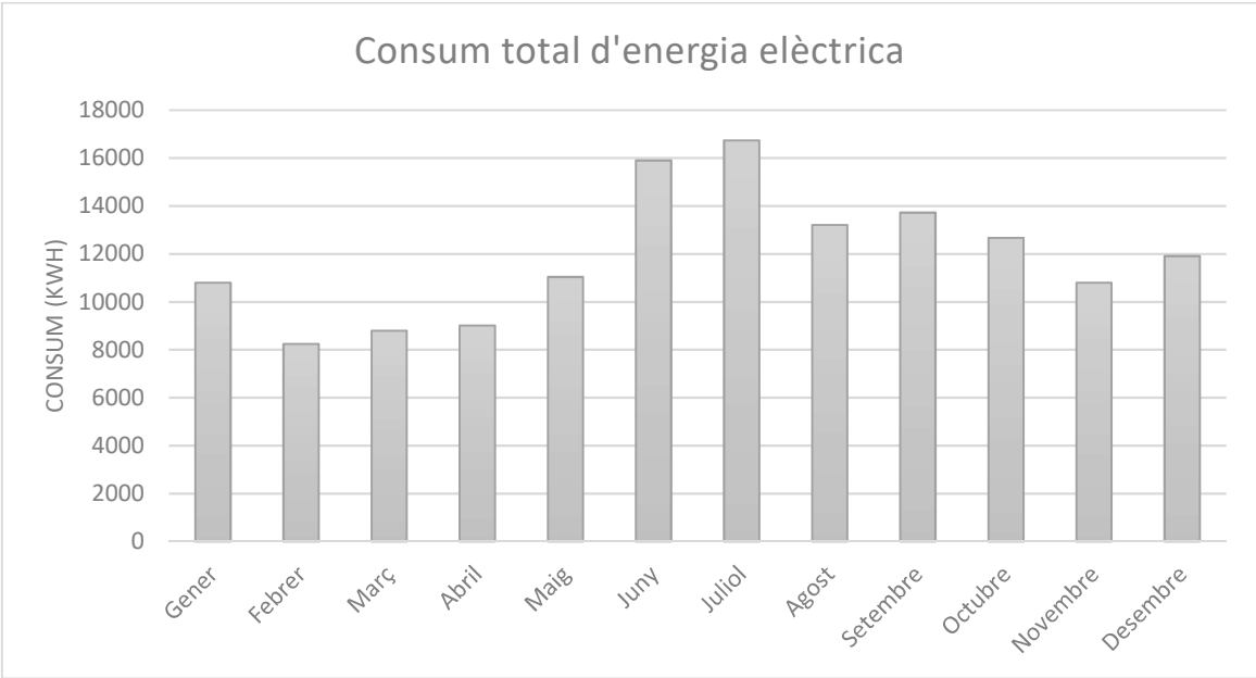
Figura 9 Consum mensual de l'EB Can Torres
