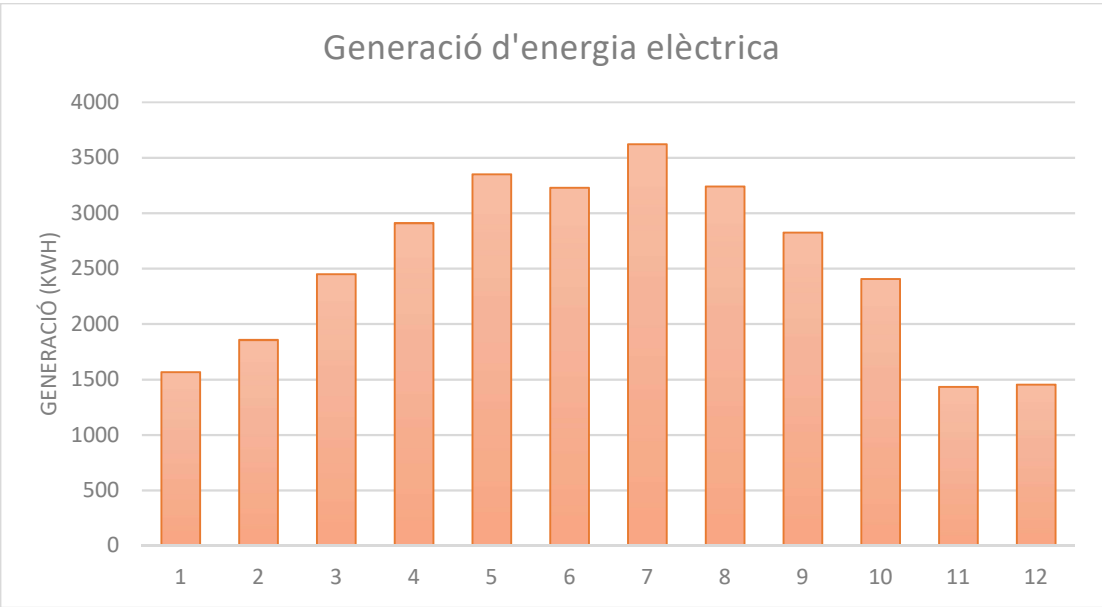
Figura 10 Generació mensual de la instal·lació FV
