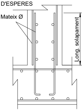
LONGITUD DE SOLAPAMENT SEGONS CODI ESTRUCTURAL
