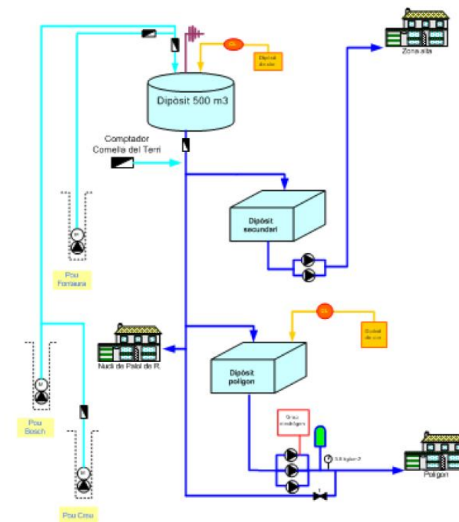
Figura 3. Esquema vertical de la xarxa actual de Palol de Revardit.
