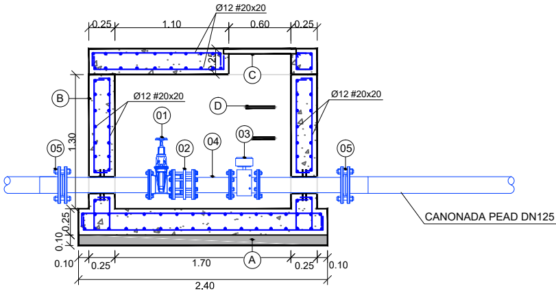
DETALL ARQUETA ESCALA:1/50
