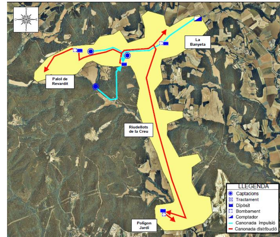
Figura 2. Esquema horitzontal de la xarxa actual de Palol de Revardit.
