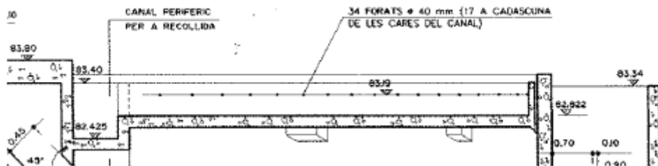
Imatge 4. Canal de sortida del decantador
