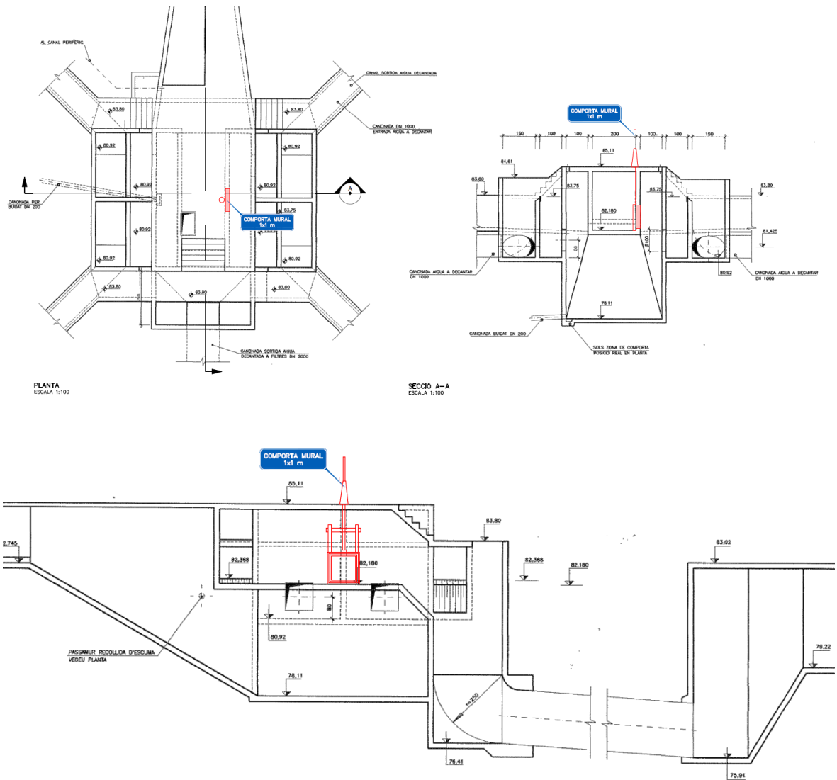
Imatge 5. Comportes proposades a mode de by-pass
