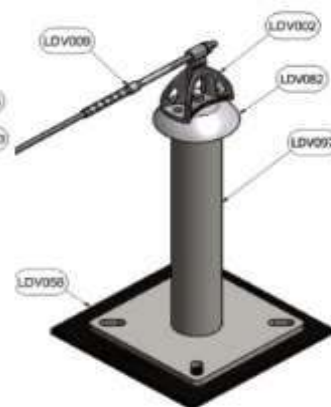
Fig. 4 Configuración de anclaje de extremo (ho con barra resaca)
