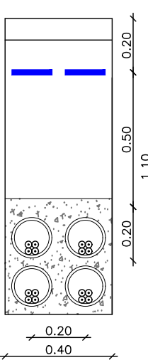
DETALL CONDUCTES ELÈCTRIQUES CREUAMENTS ESCALA 1:20
