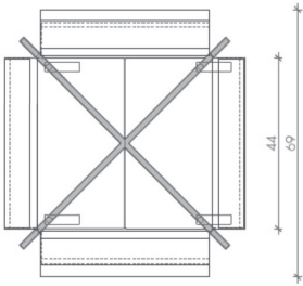
Planta
