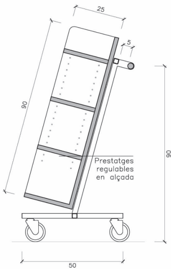
SECCIÓ
