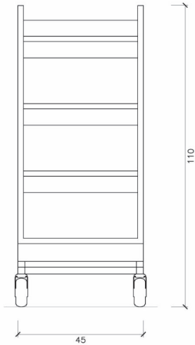
ALÇAT FRONTAL
