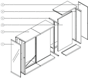
Secció tipus
