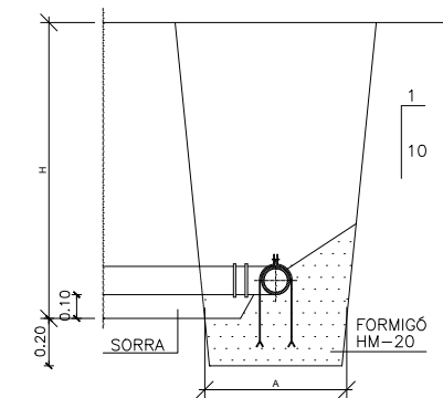
SECCIÓ A-A
