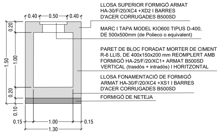
SECCIÓ S1
