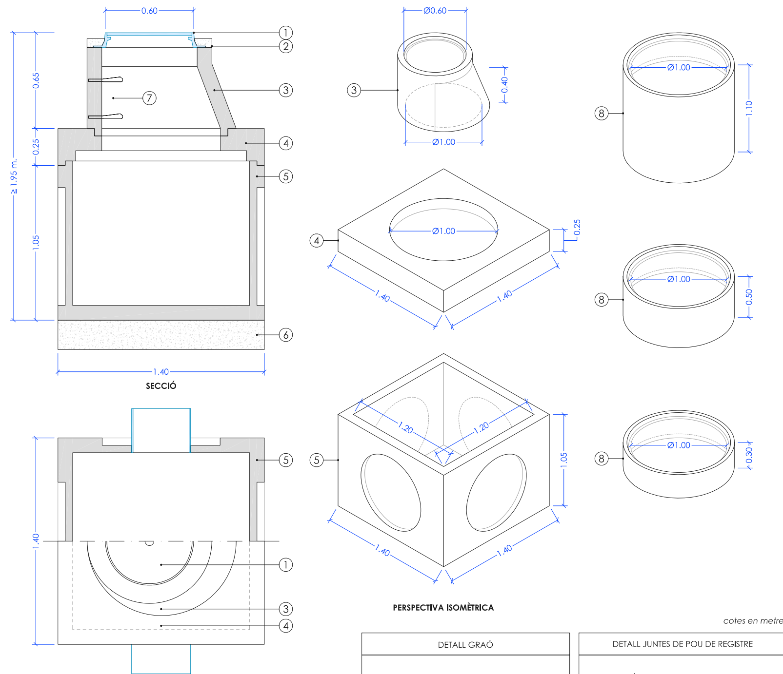
POU DE REGISTRE TIPUS II - ESCALA 1/25
