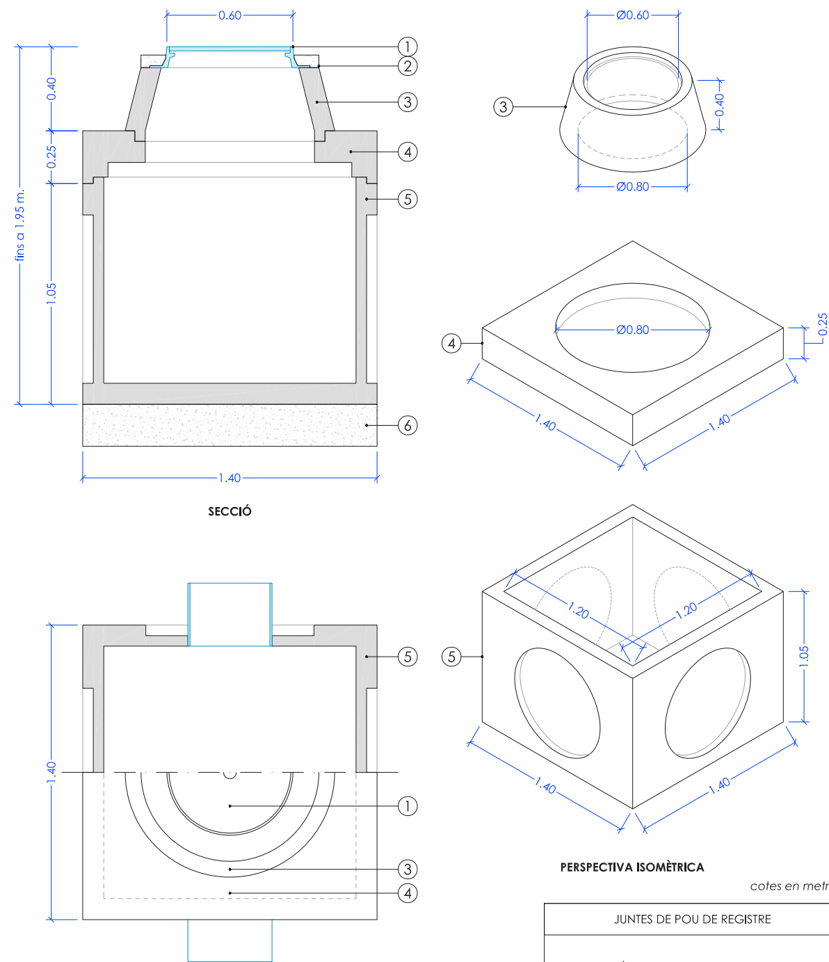
POU DE REGISTRE TIPUS I - ESCALA 1/25
