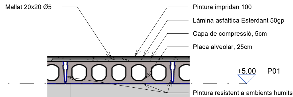
6 Detall 2 A.01/03 1 : 25
