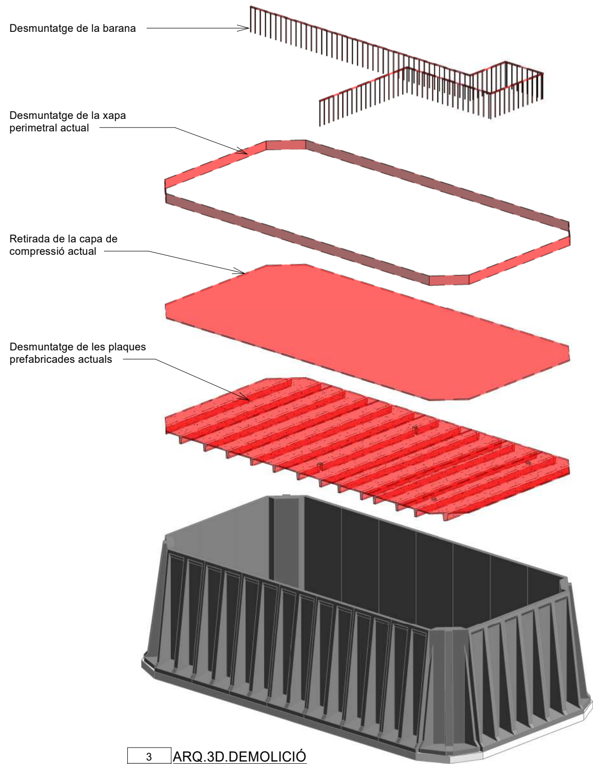
3 ARQ.3D.DEMOLICIÓ A.01/01
