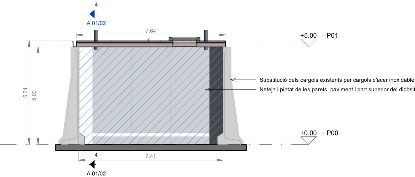
8 Secció 2 A.01/02 1 : 100
