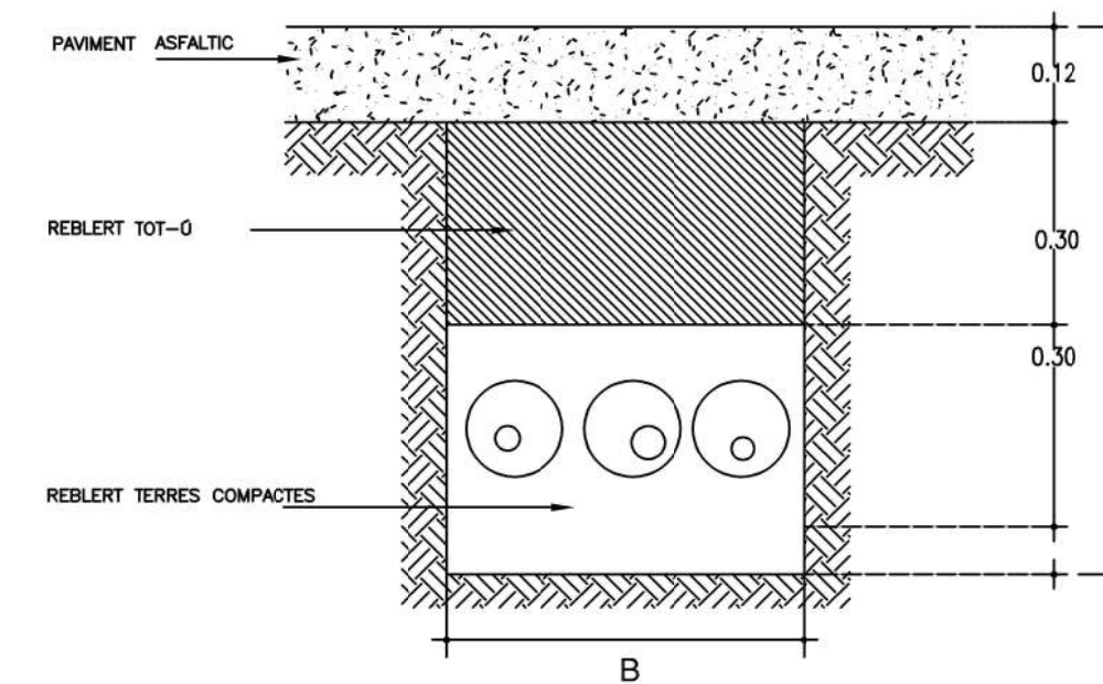
DETALL RASA EN PAVIMENT ASFALTIC
