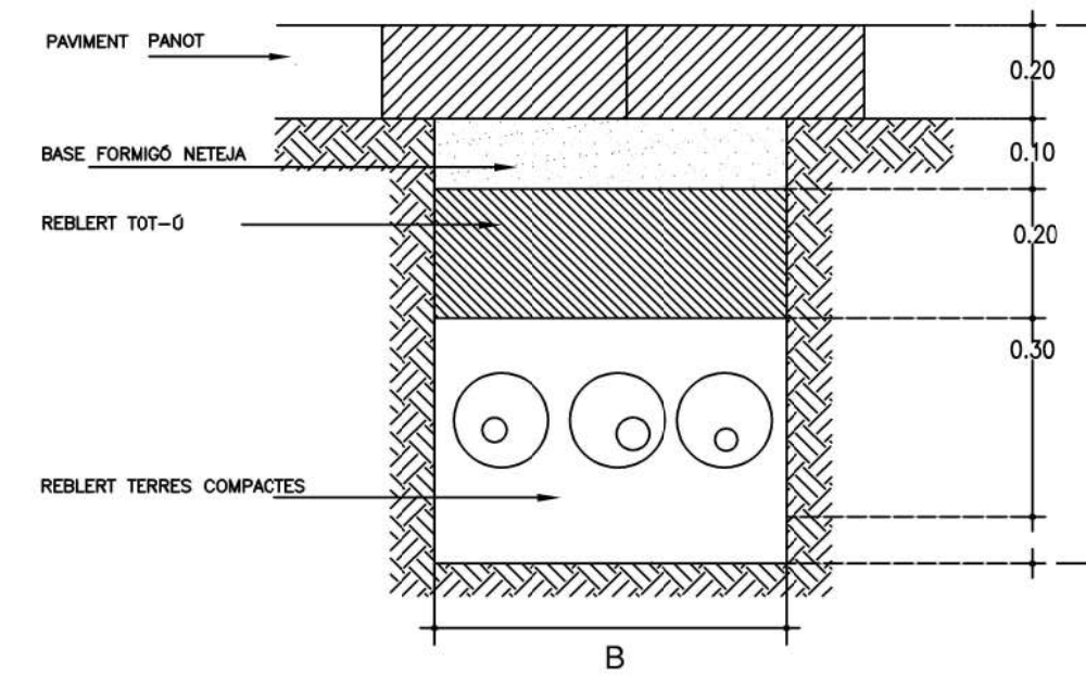
DETALL RASA EN VORERA DE PANOT
