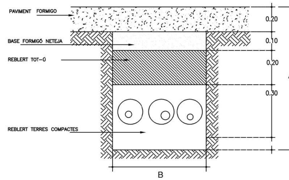
DETALL RASA EN VORERA DE FORMIGÓ
