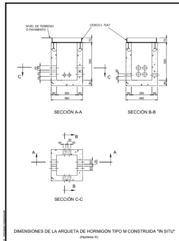
DIMENSIONES DE LA ARQUETA DE HORMIGÓN TIPO M CONSTRUIDA "IN SITU" (Figura 8)
