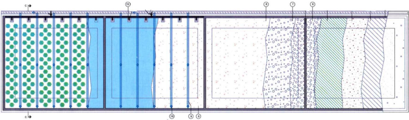
PLANTA ESTAT ACTUAL. E:1/100
