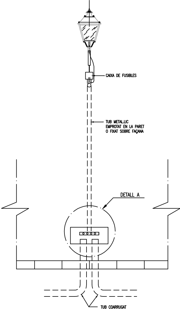
ALÇAT
