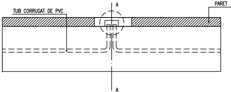
ALÇAT
