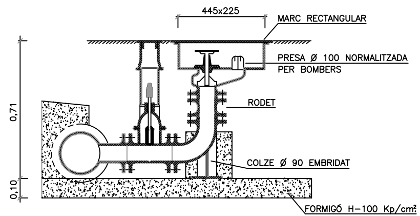
HIDRANT SOTERRAT AMB VÀLVULA
