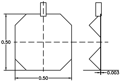
CONEXIO A TERRA DETALL 2
