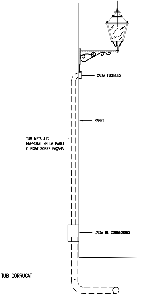
SECCIÓ A-A
