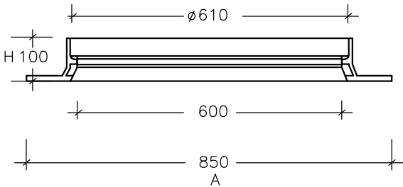
SECCIÓ BASTIMENT
