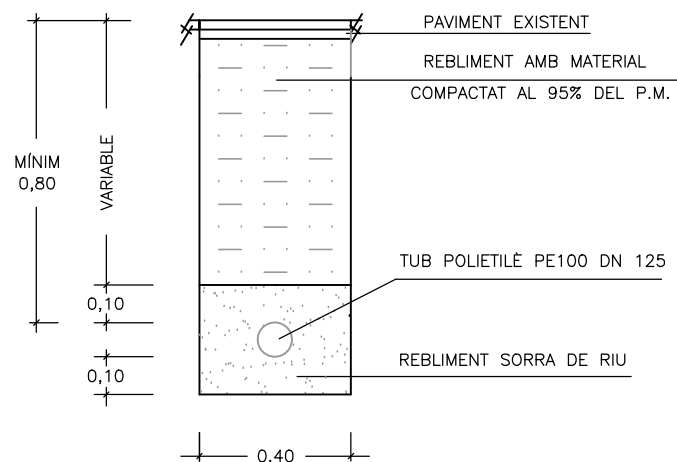
RASA TIPUS TUB D'AIGUA POTABLE ESCALA=1:20
