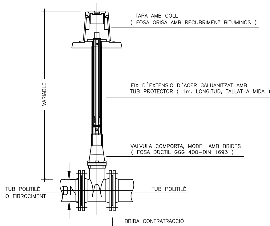
VÀLVULA COMPORTA DN 125 SENSE ESCALA
