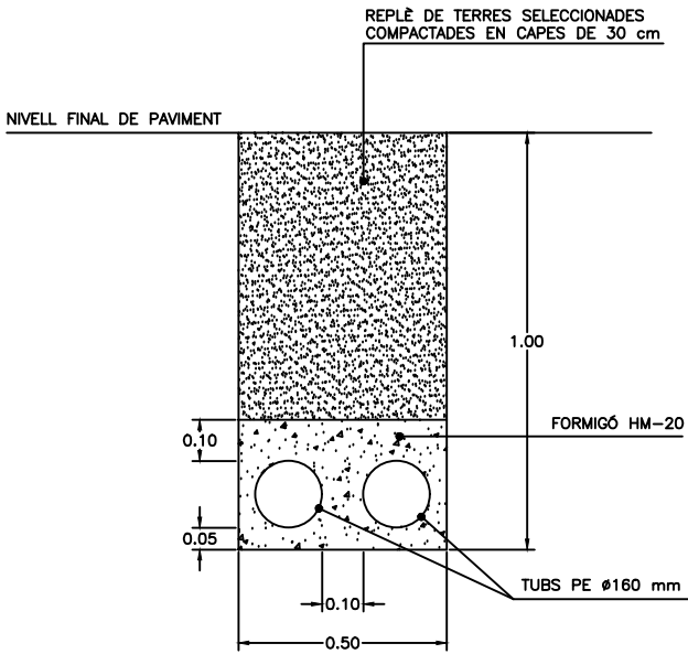
RASA BAIXA TENSIO ESCALA = 1/20
