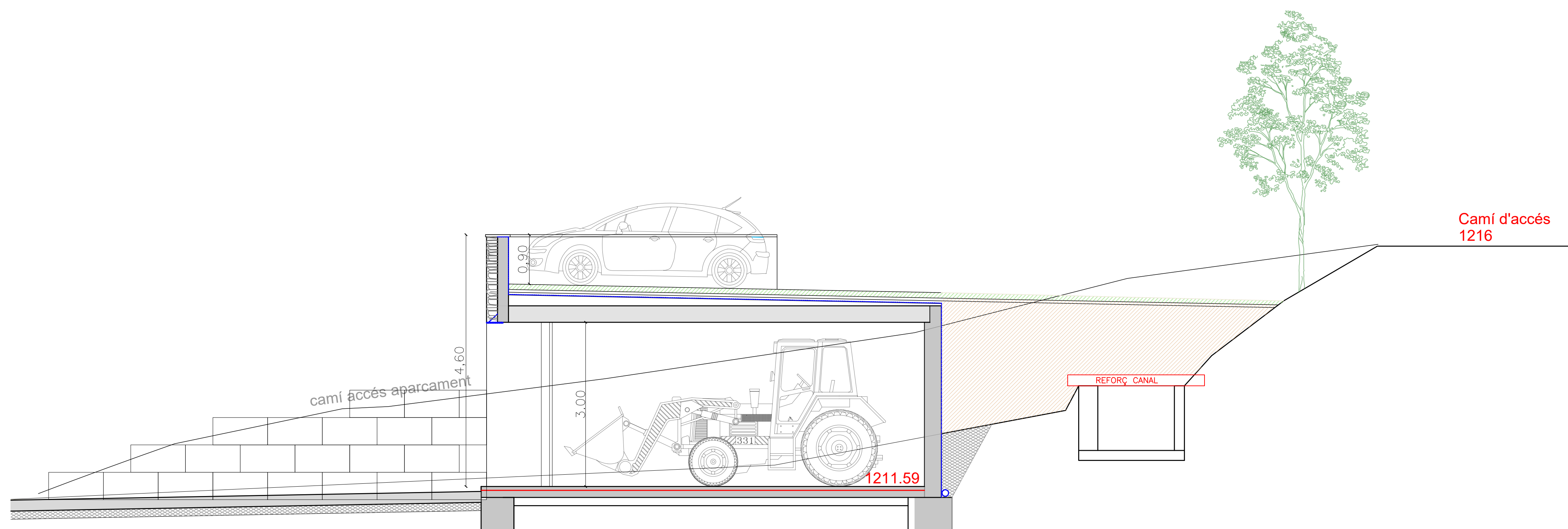
SECCIÓ TRANSVERSAL
