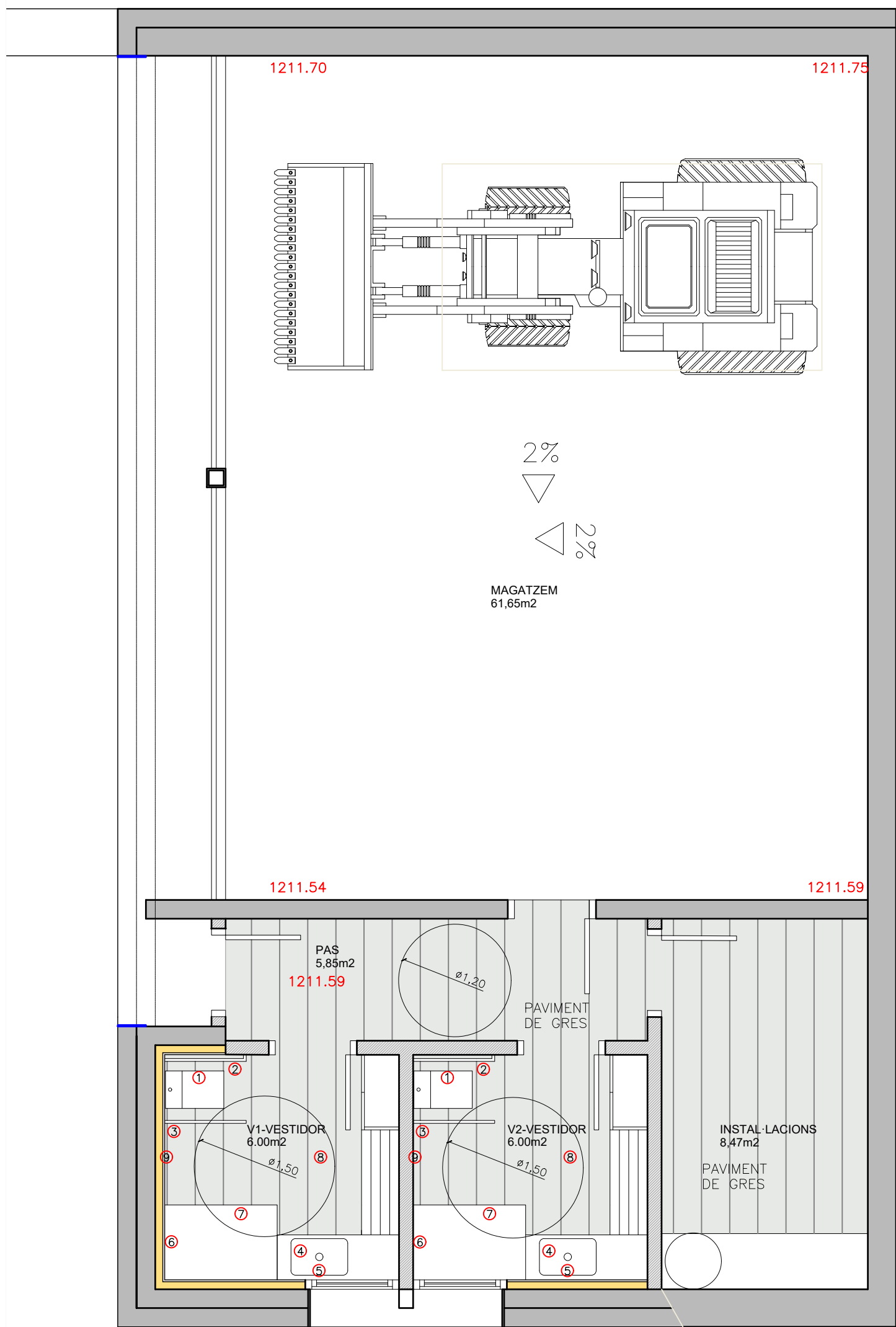
PLANTA MAGATZEM
