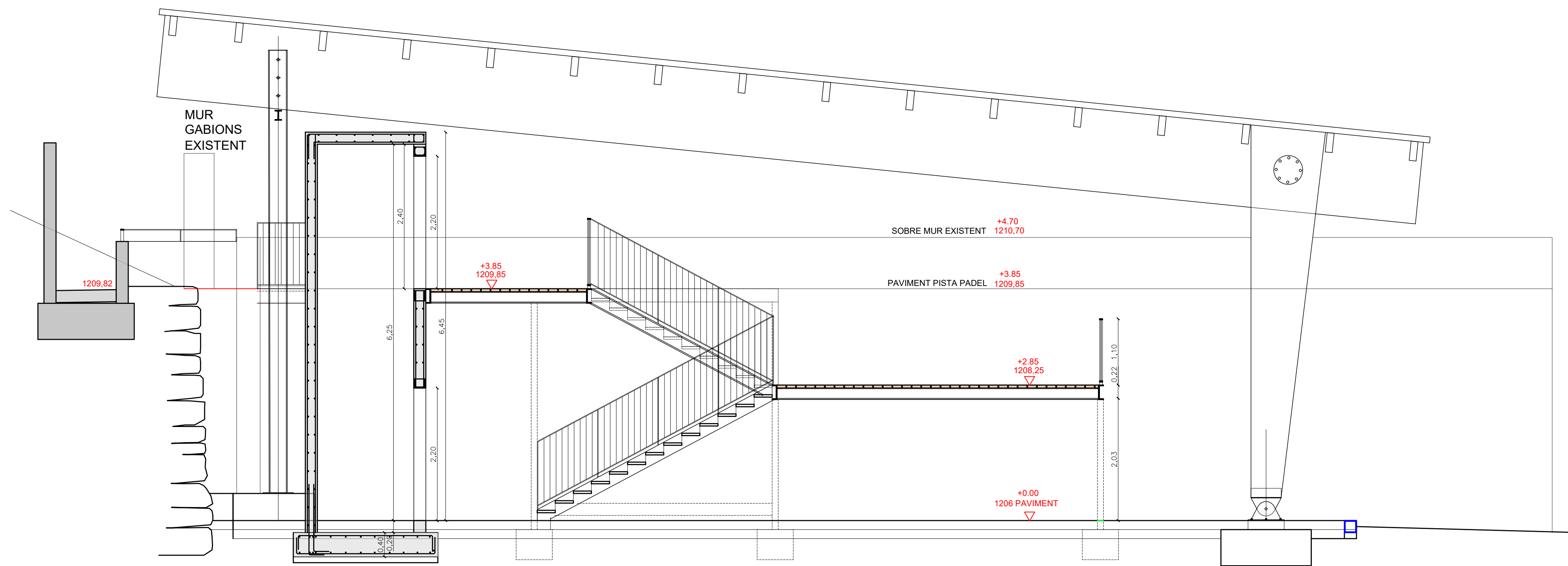
SECCIÓ ASCENSOR I ESCALA
