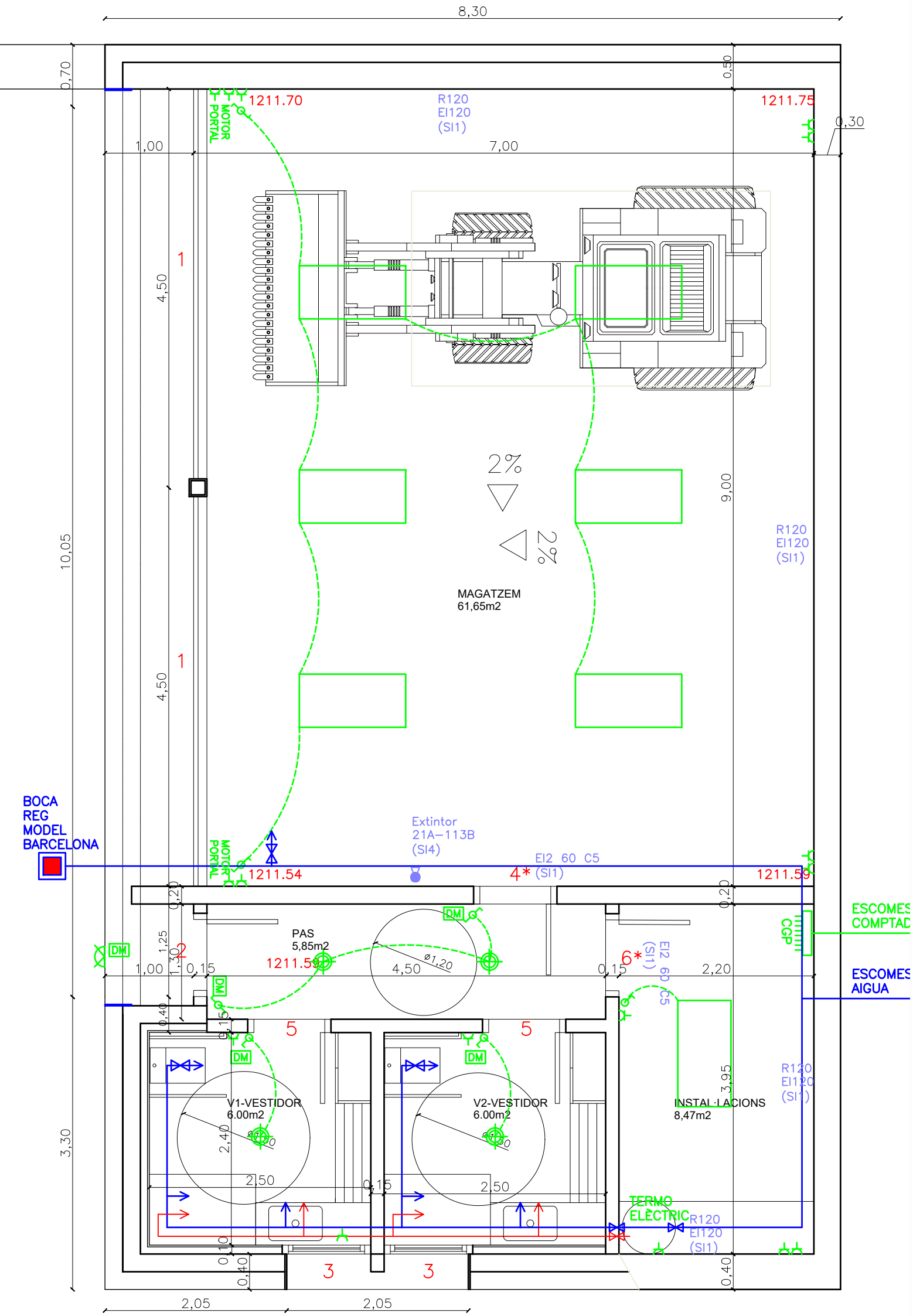
PLANTA MAGATZEM
