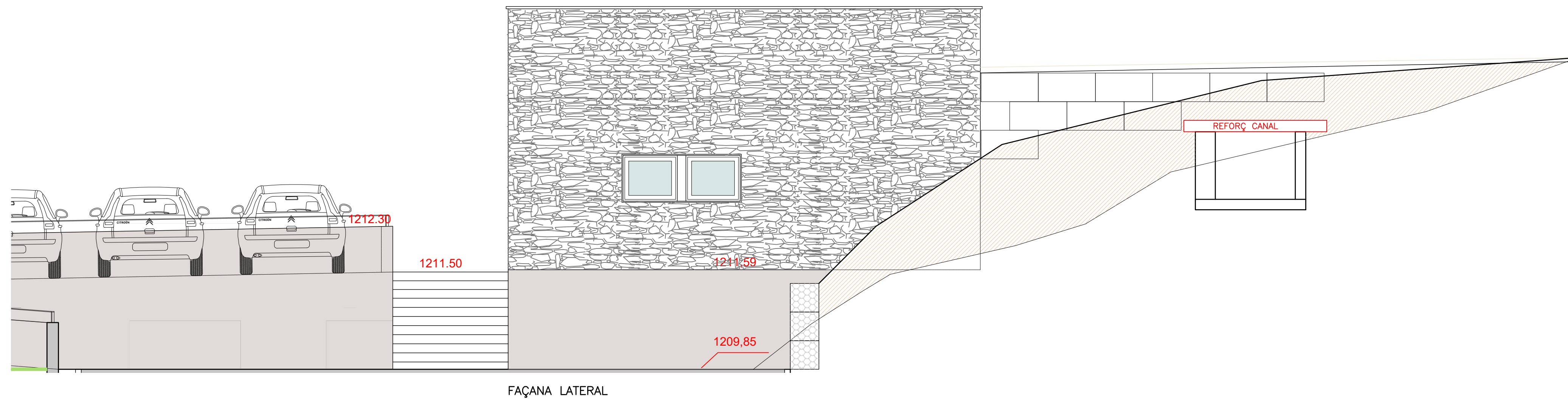
FAÇANA LATERAL
