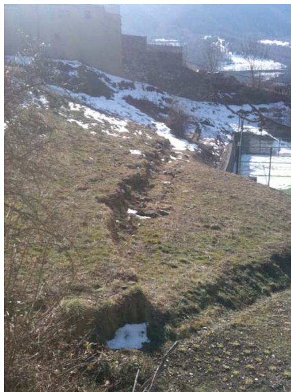
FOTOGRAFIA 2. Aflorament del dipòsit col·luvial quaternari (sorres i gravetes llimoses) en el vessant natural.
