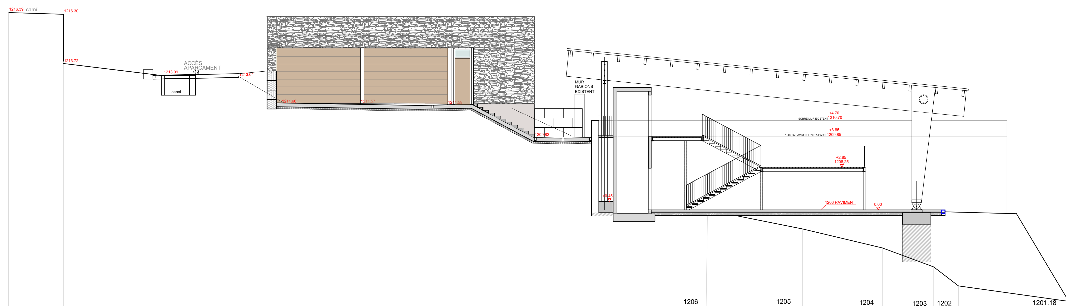
SECCIÓ B
