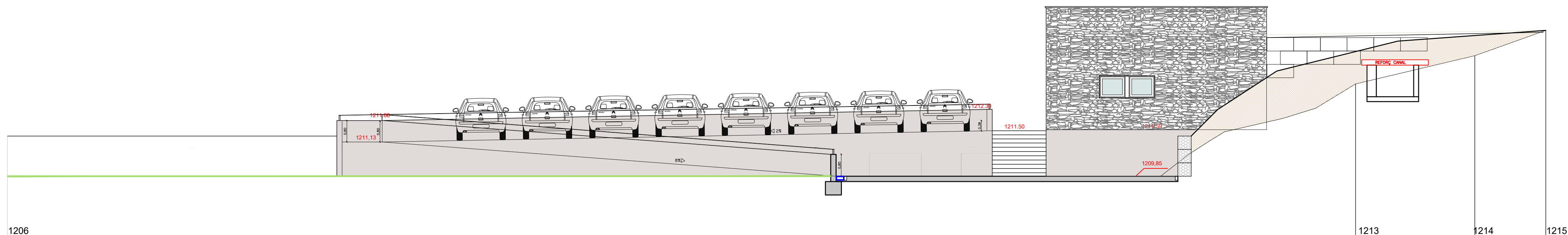
SECCIÓ E
