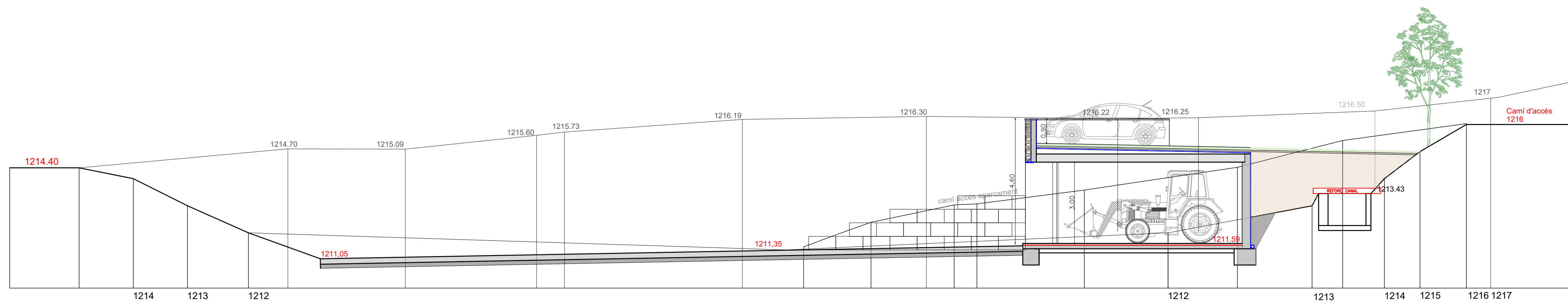
SECCIÓ D
