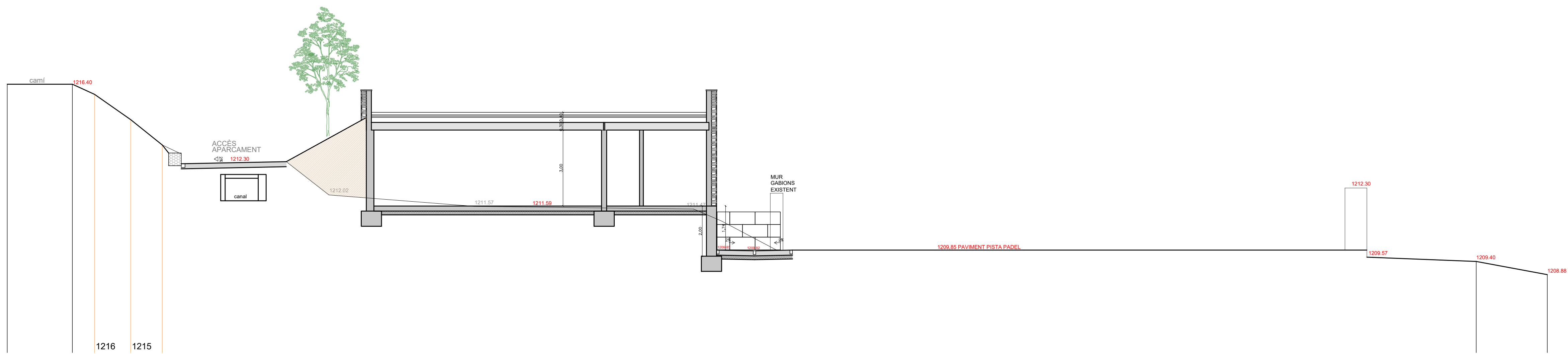
SECCIÓ A
