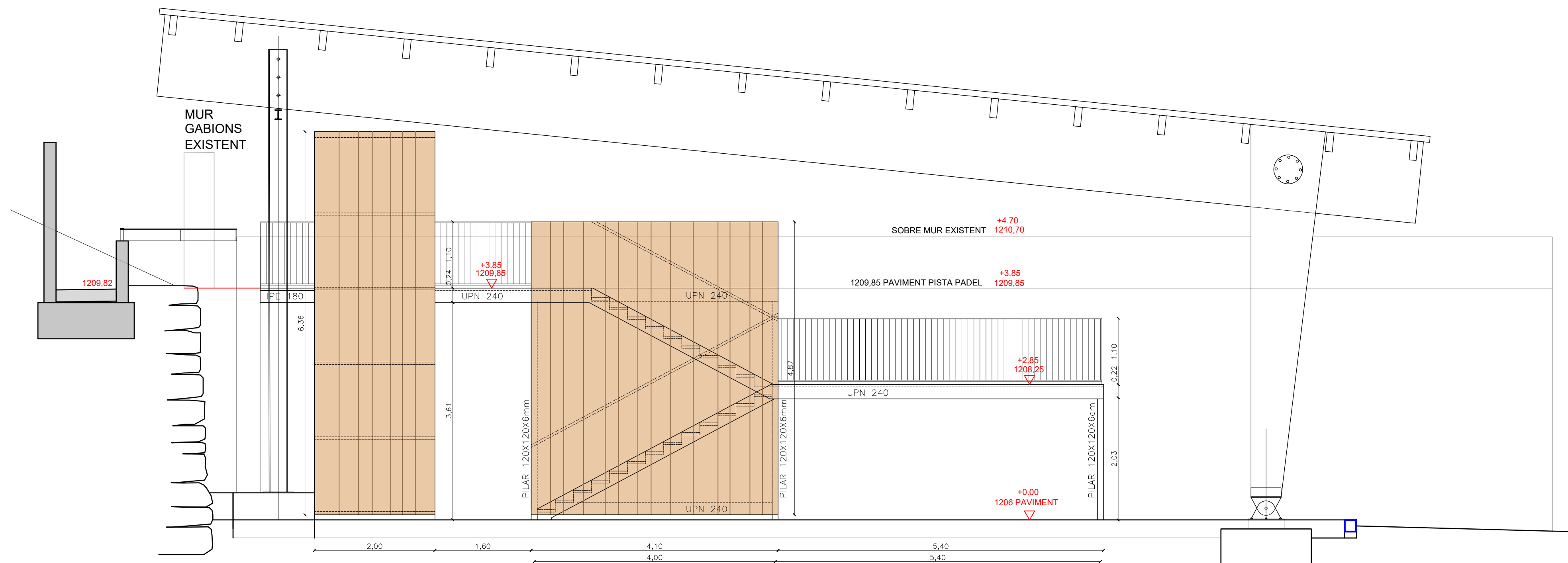
ALÇAT ASCENSOR I ESCALA
