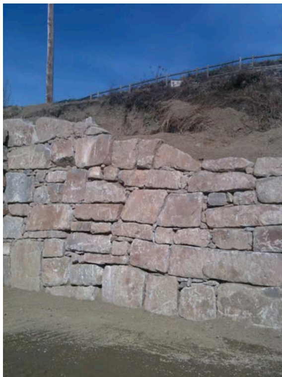
FOTOGRAFIA 3. Aflorament parcial del dipòsit col·luvial quaternari (sorres i gravetes llimoses) per sobre d'una escullera de nova construcció.
