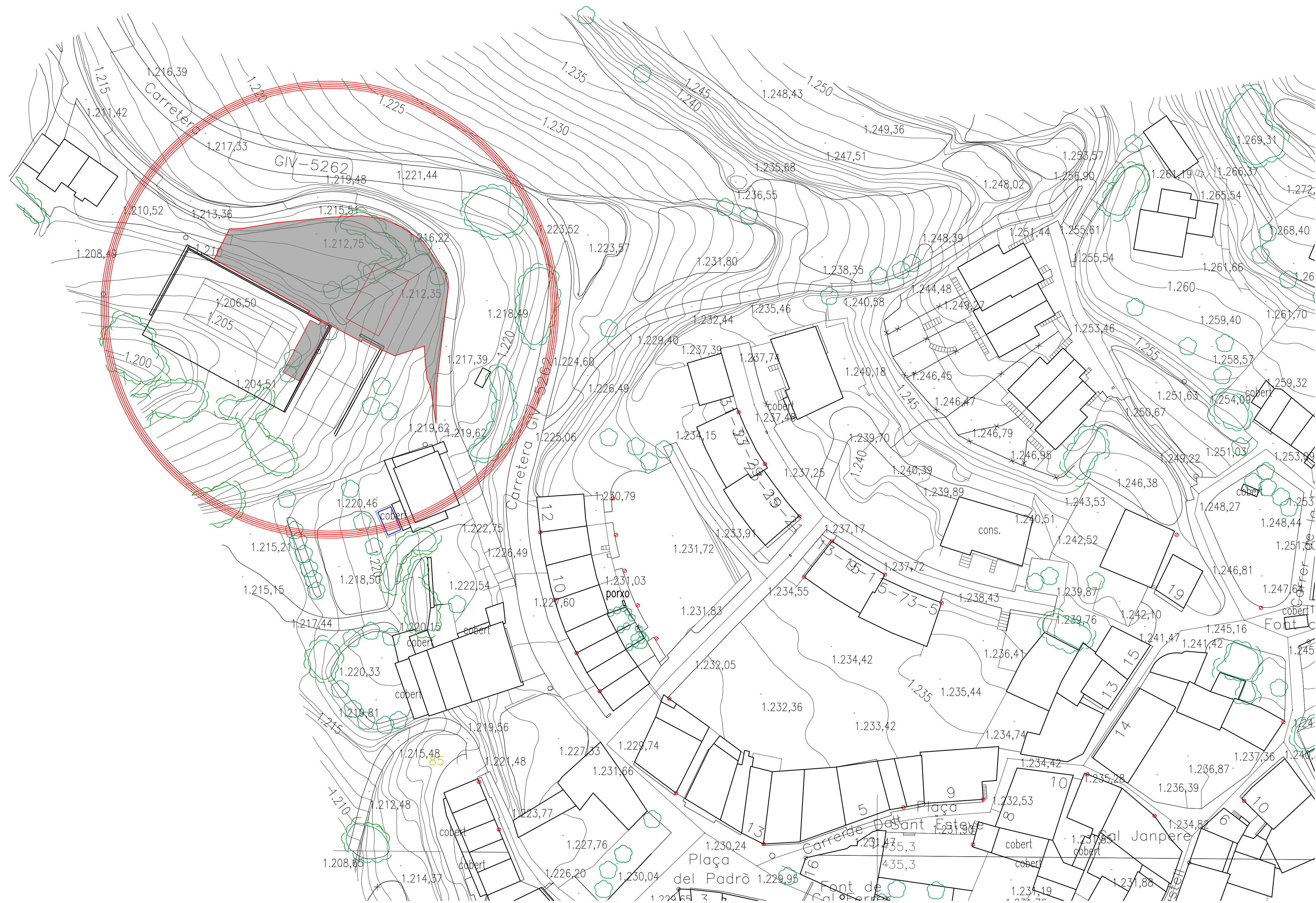
EMPLAÇAMENT 1:500
