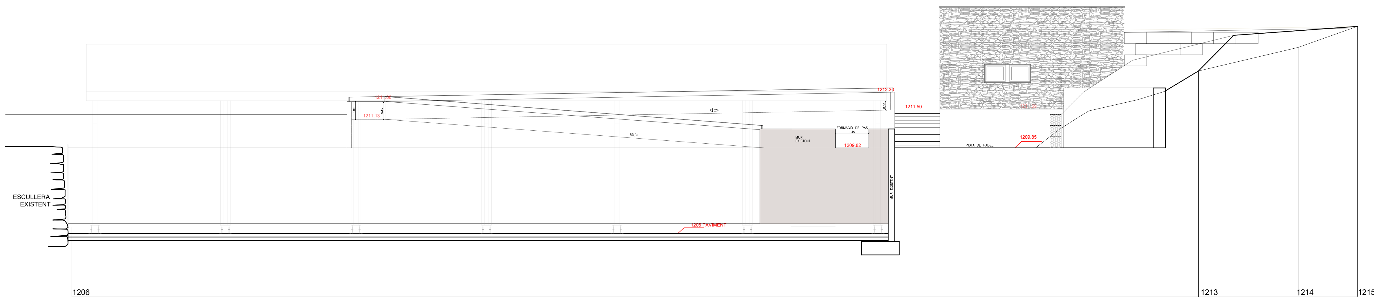
SECCIÓ F
