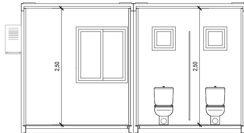
SECCIÓ A-A'
