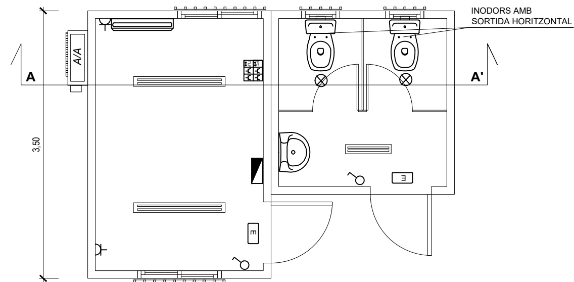
PLANTA
