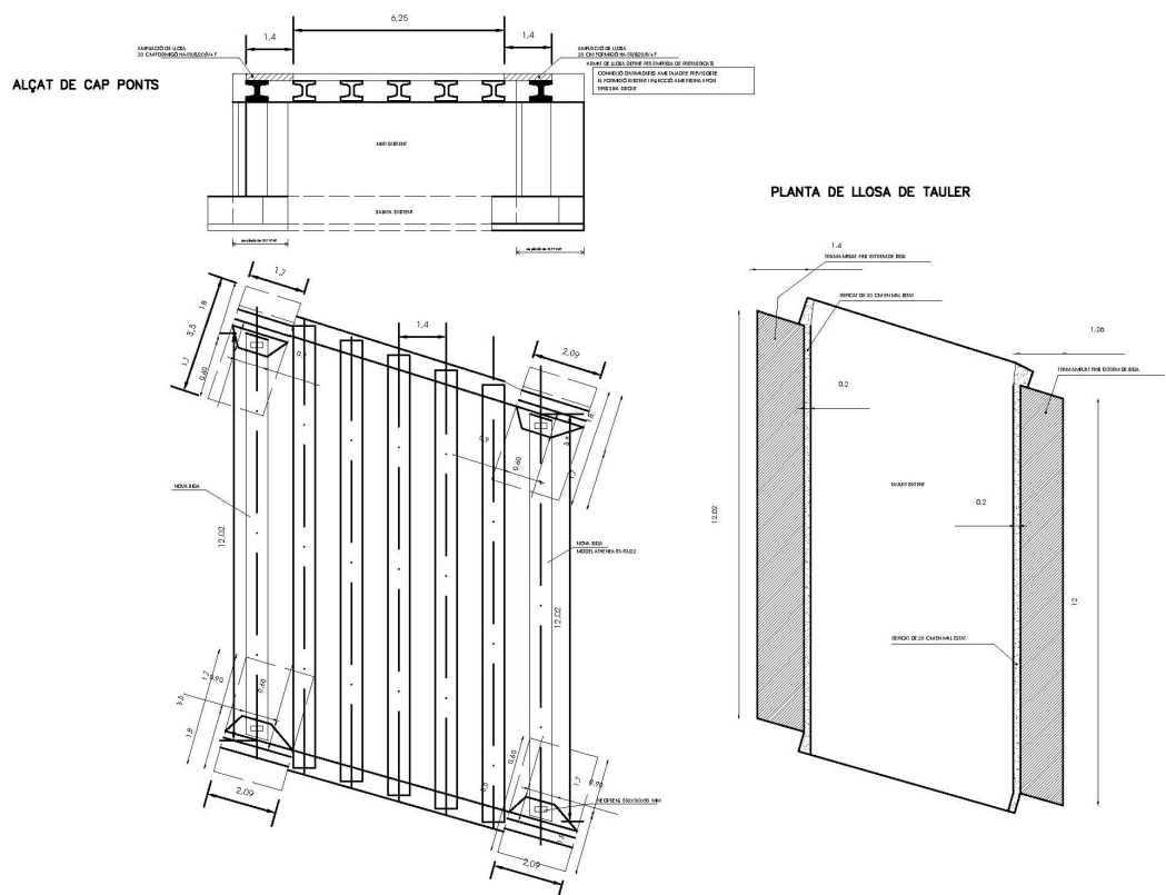
Projecte de reparació i eixample del pont desaparegut l'any 2007
