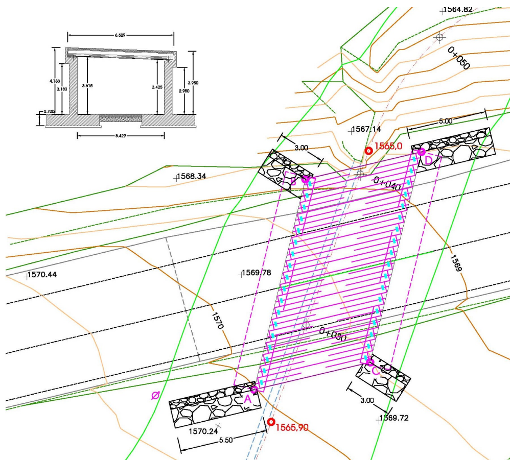
Alternativa núm. 3.- Bigues "TL" de formigó pretesat. Sección neta de 545x350 cm
