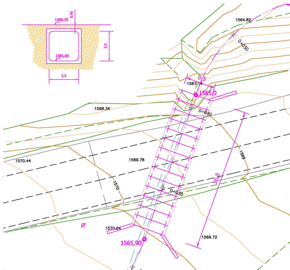
Alternativa núm. 2.- Marcs prefabricats de formigó armat de 350x350 cm
