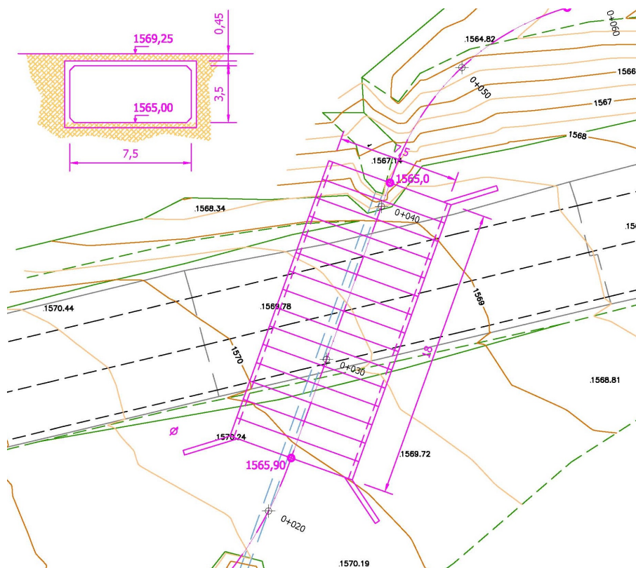
Alternativa núm. 1.- Marcs prefabricats de formigó armat de 750x350 cm
