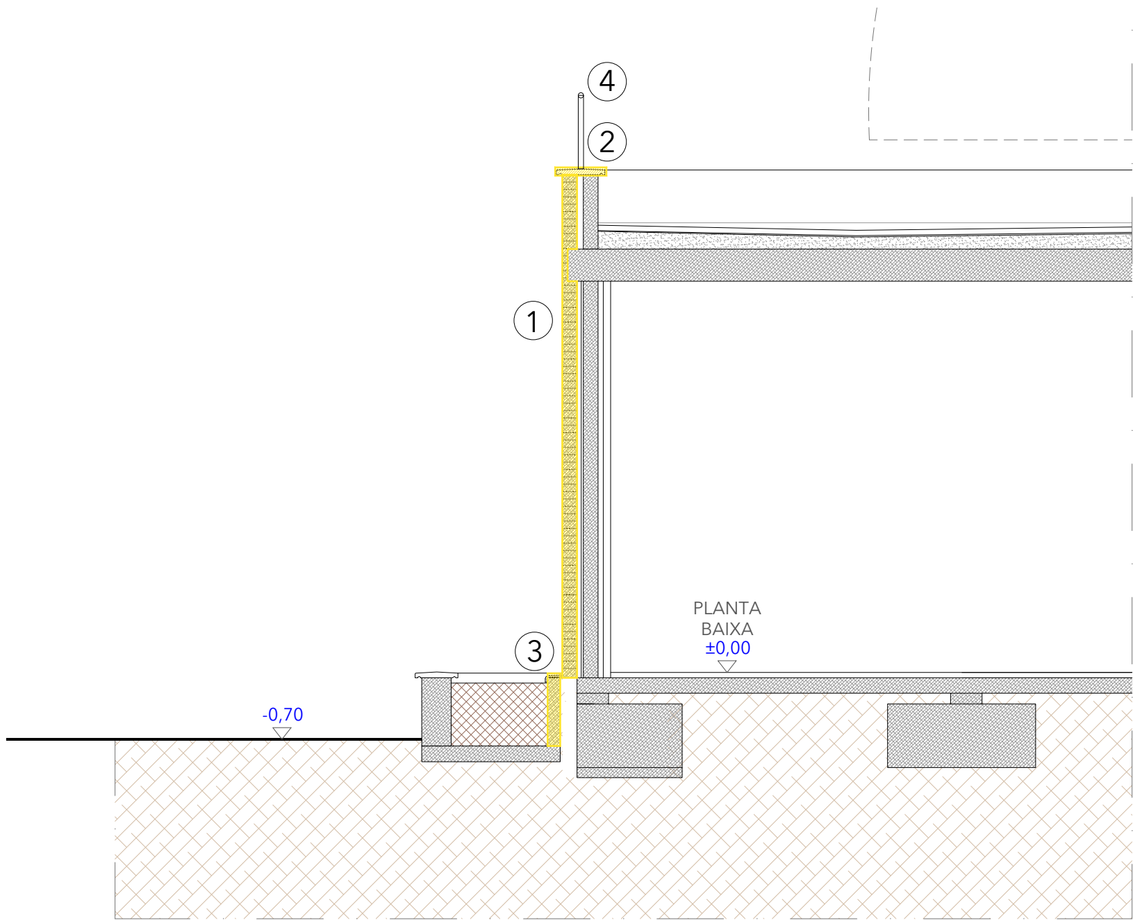
SECCIÓ e: 1/50
