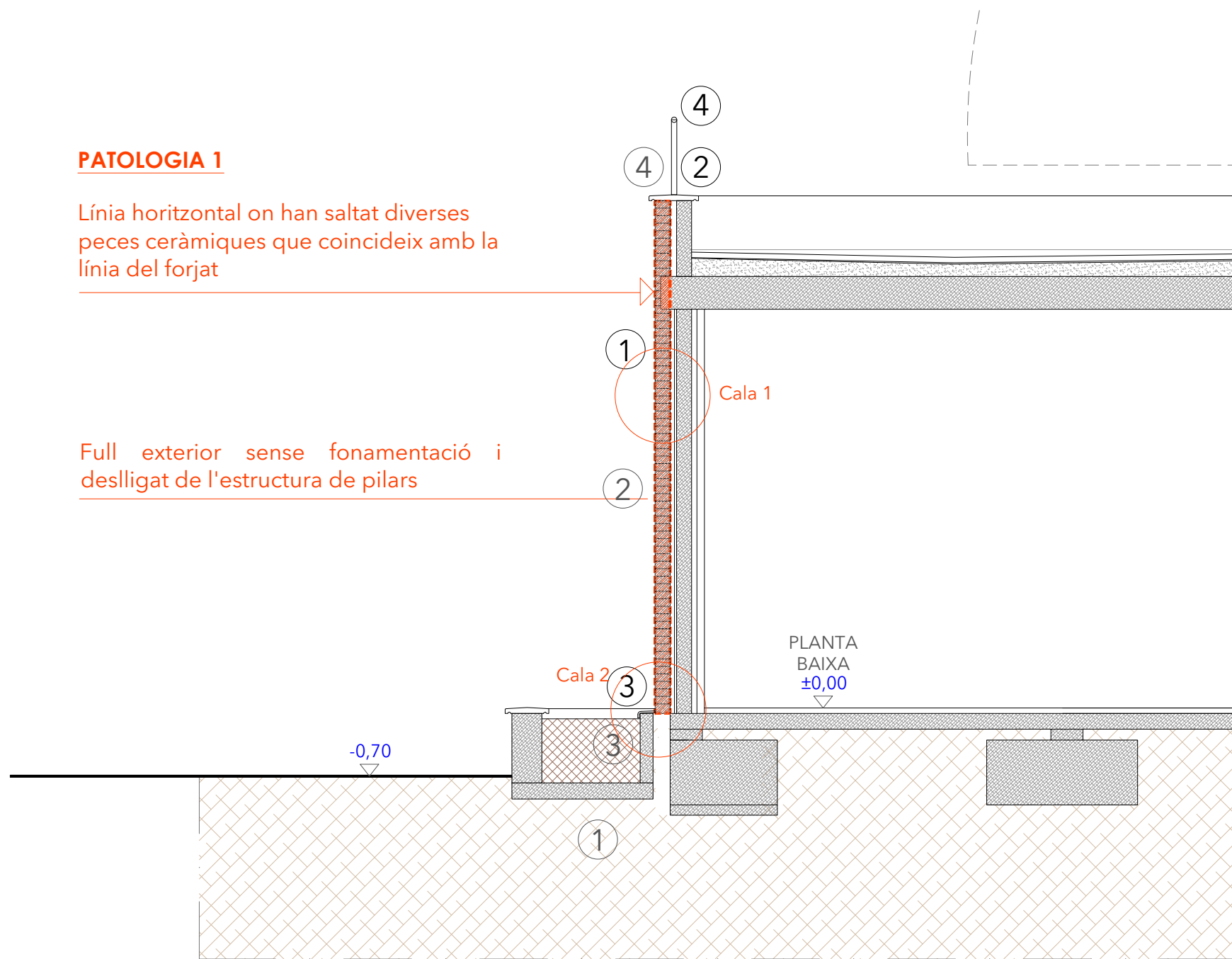
SECCIÓ e: 1/50
