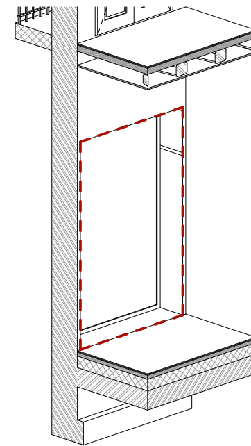
Intervenció 1:75
