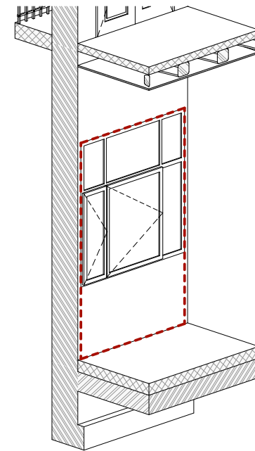
Estat actual 1:75
