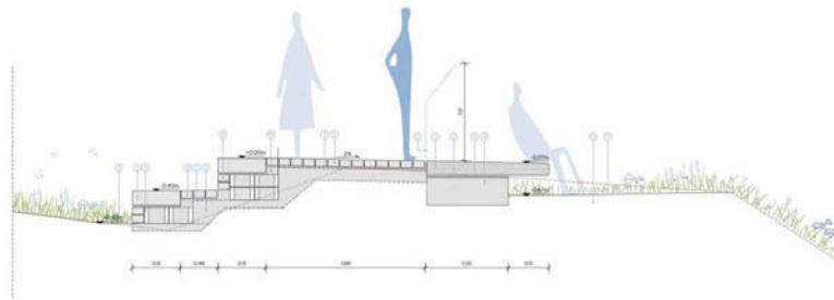
Secció tipus del projecte (graderies – Banc mirador)
