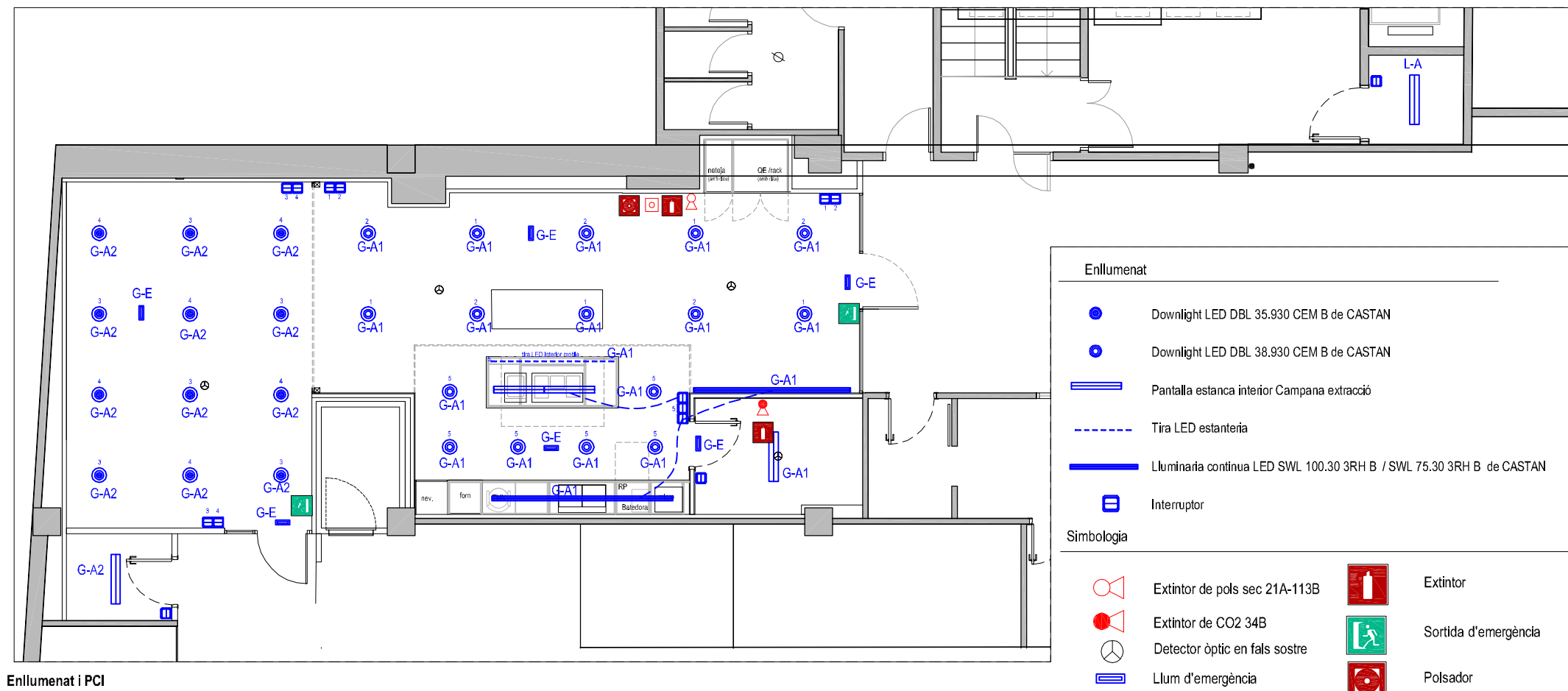
Enllumenat i PCI
