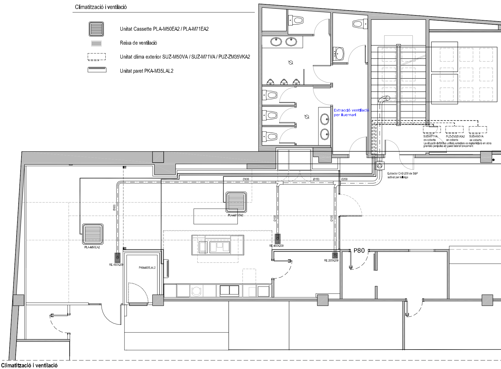
Climatització i ventilació
