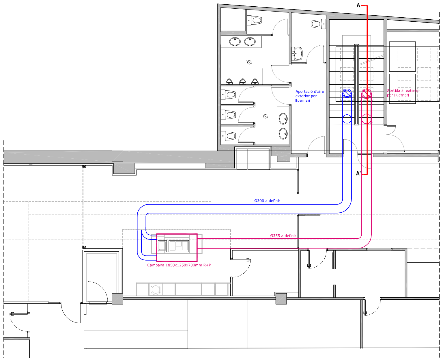
Planta baixa_Campana, extracció/aportació
