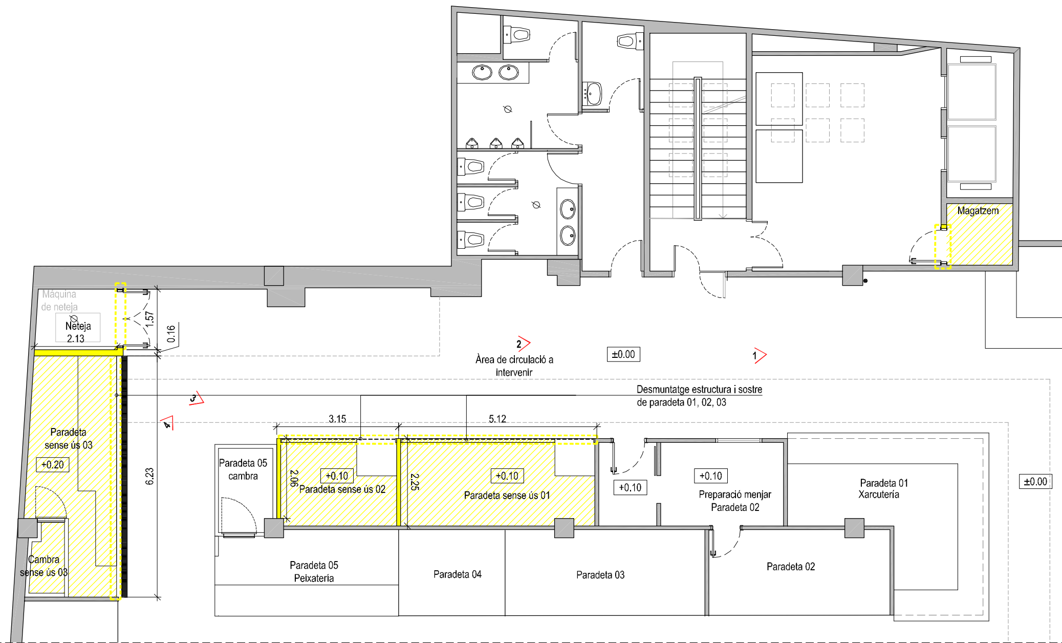
Planta enderroc
