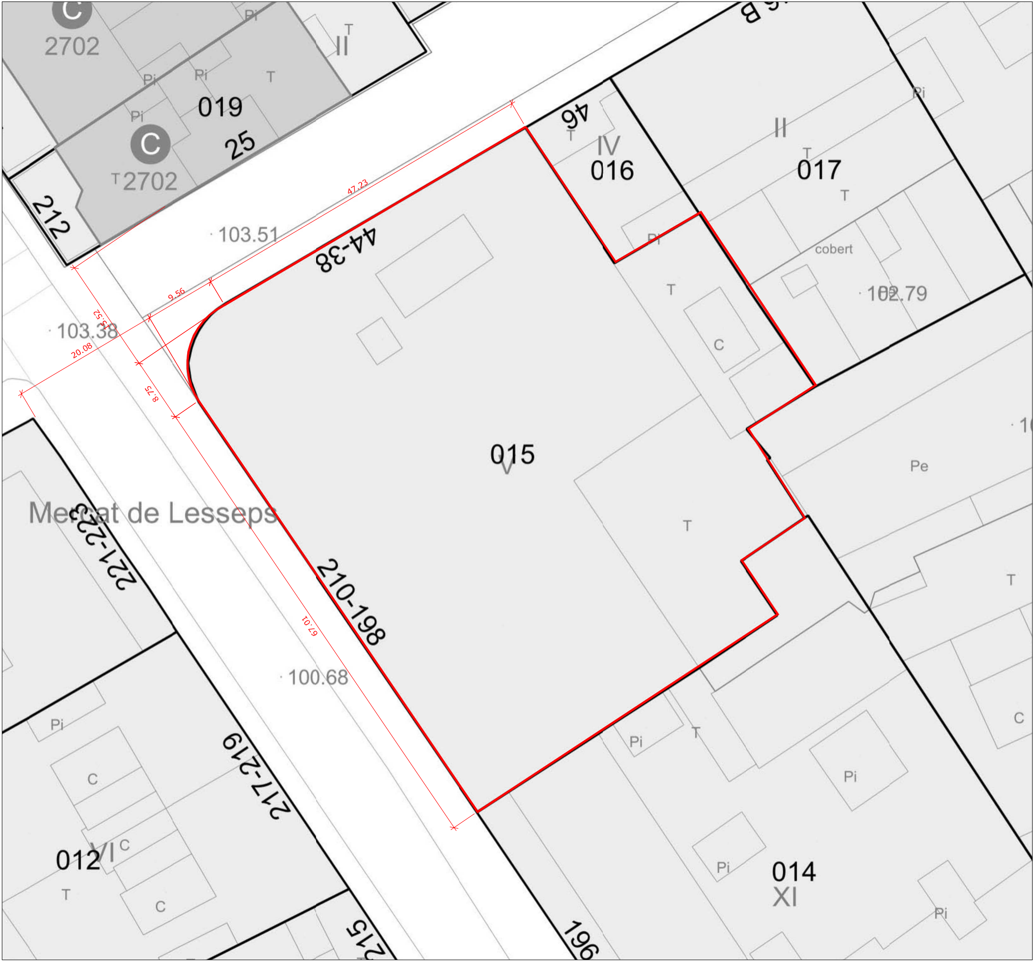
Emplaçament 1/500
