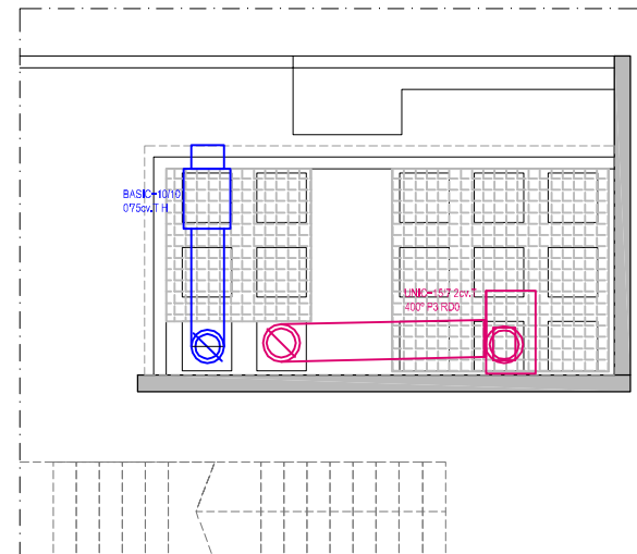
Coberta_Campana, extracció/aportació
