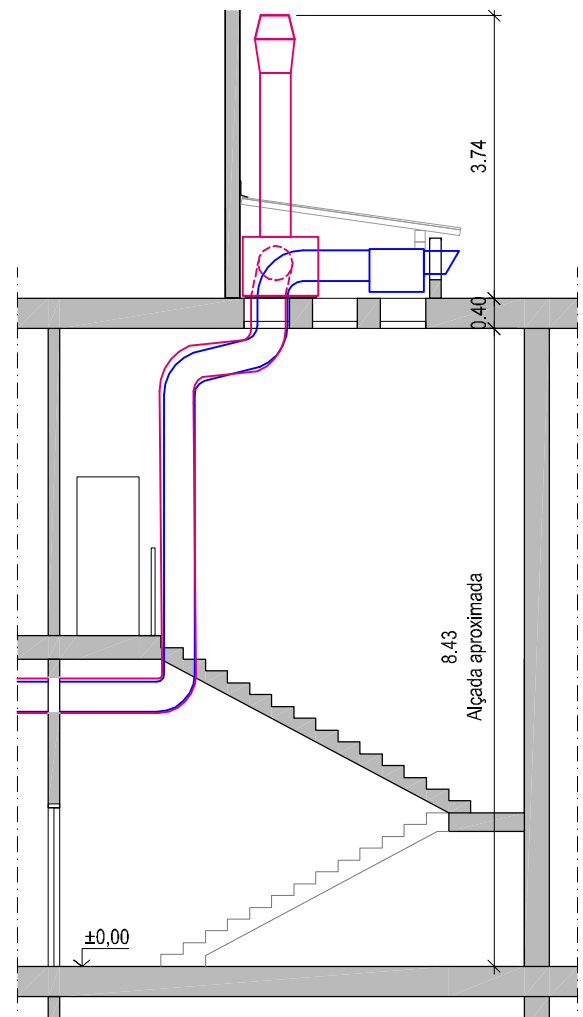
Secció A-A'_Campana, extracció/aportació
