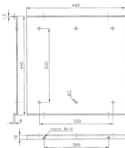
SUPORT
