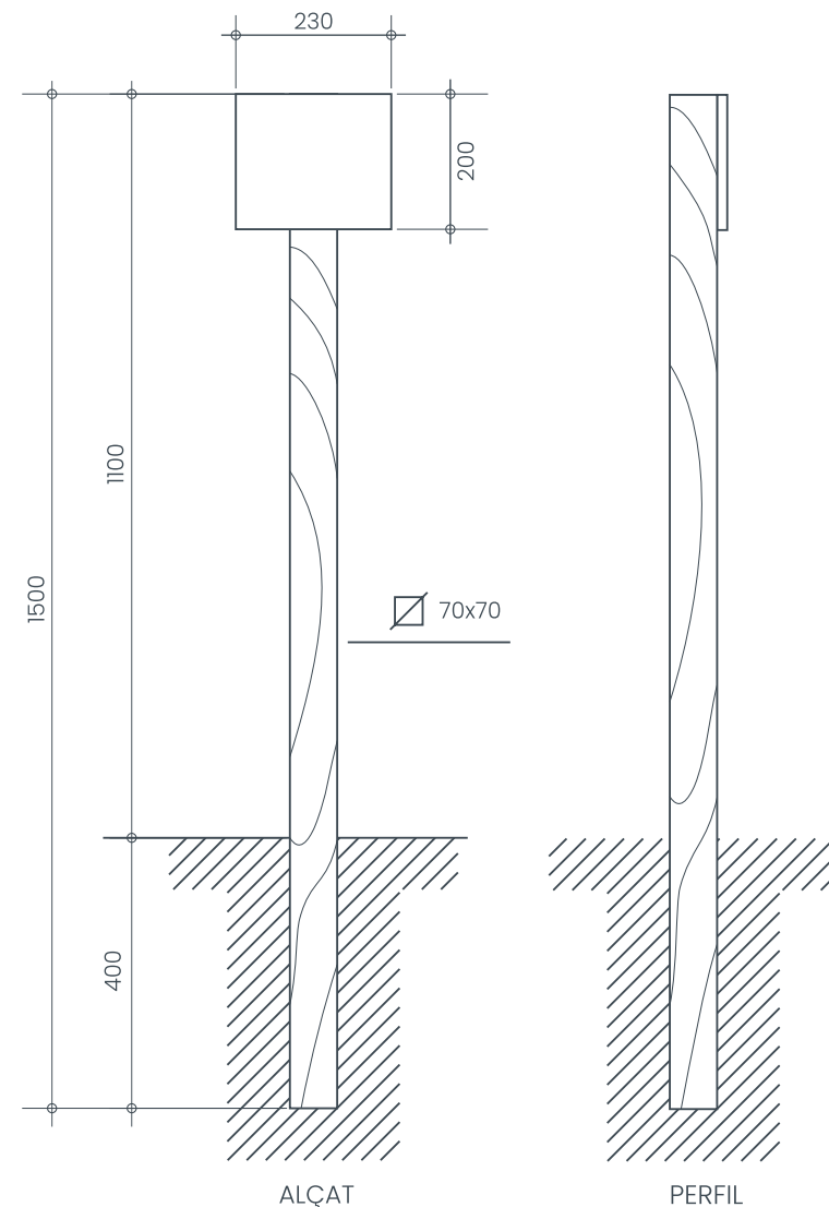
SUPPORT D'ANCORATGE
