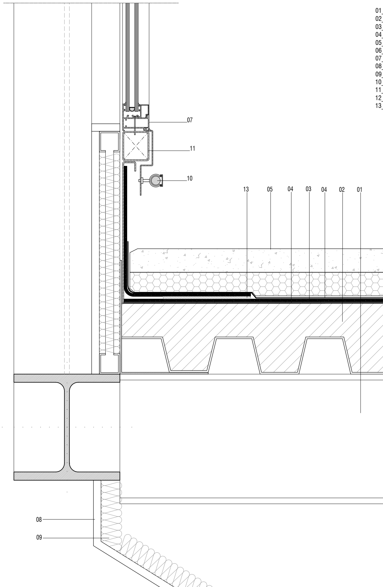
DETALL 1 A1 E.1/2 A3 E.1/4
