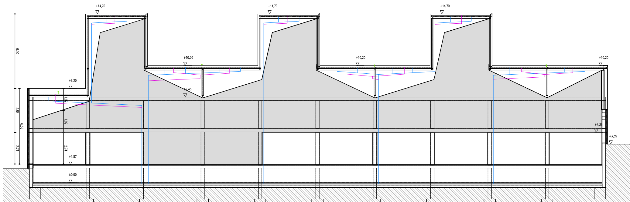
SECCIÓ LONGITUDINAL
