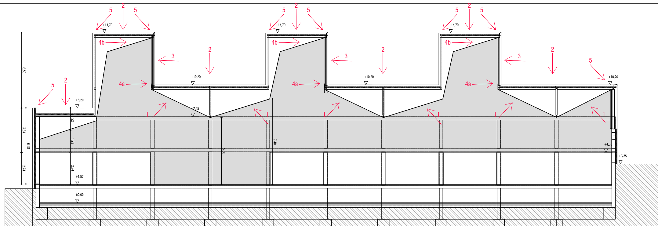
SECCIÓ LONGITUDINAL
