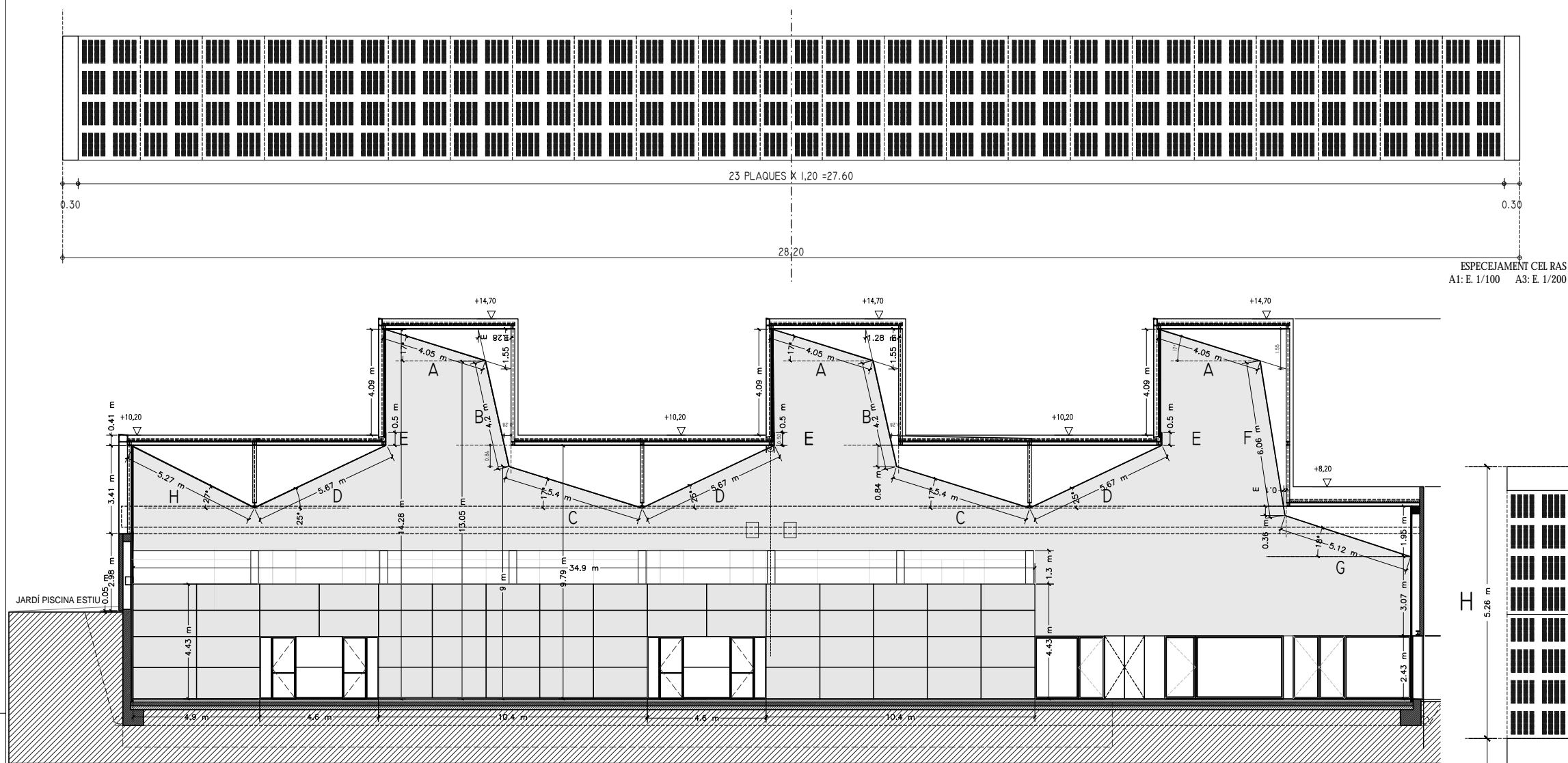
ALÇATA ACCÉS VESTIDORS A1: E. 1/100 A3: E. 1/200
