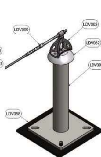
Fig. 4 Configuración de anclaje de un extremo con barra roscada
