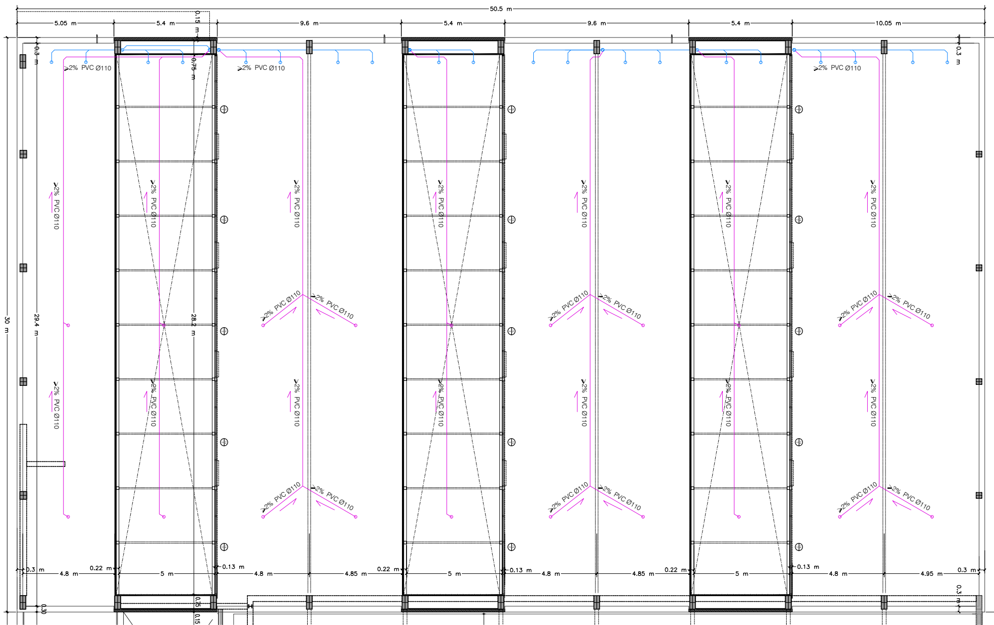
PLANTA COBERTA
