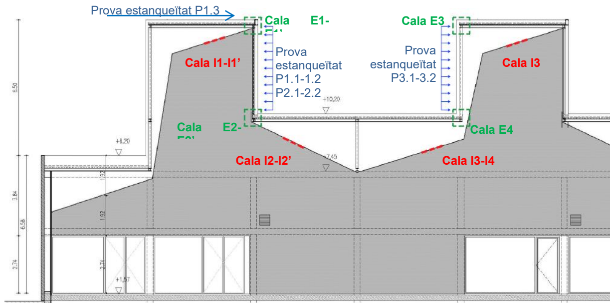
Figura RT-2 Situació de les cales en secció
