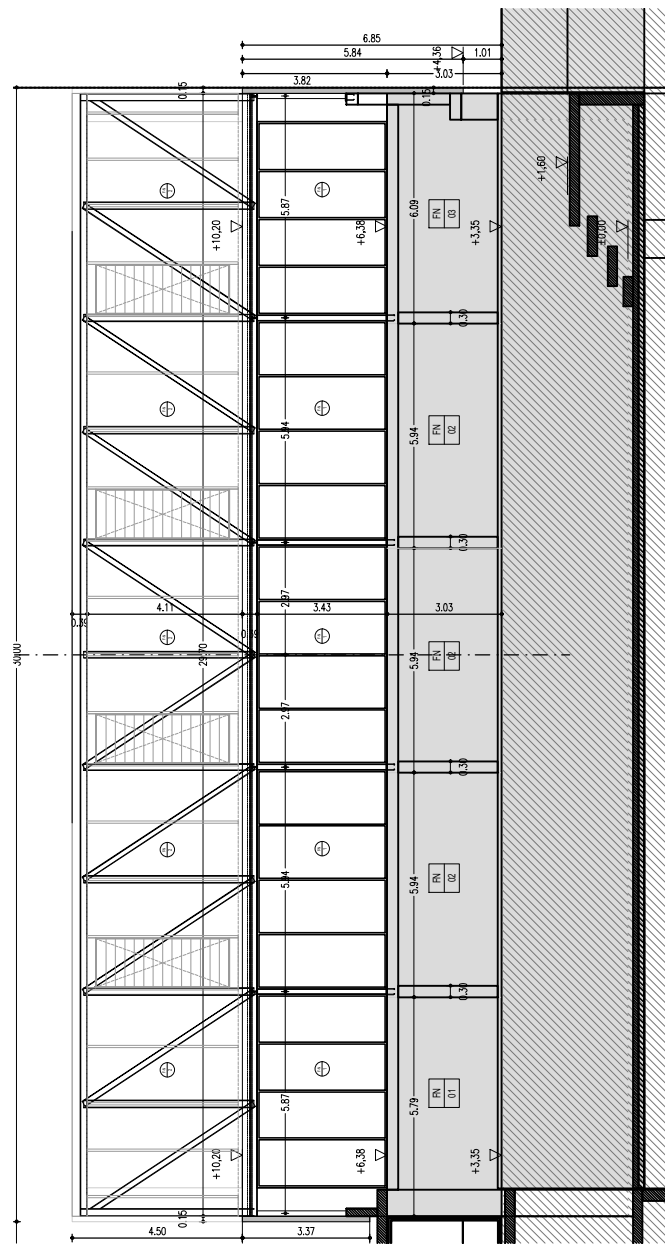
SECCIÓ TRANSVERSAL
