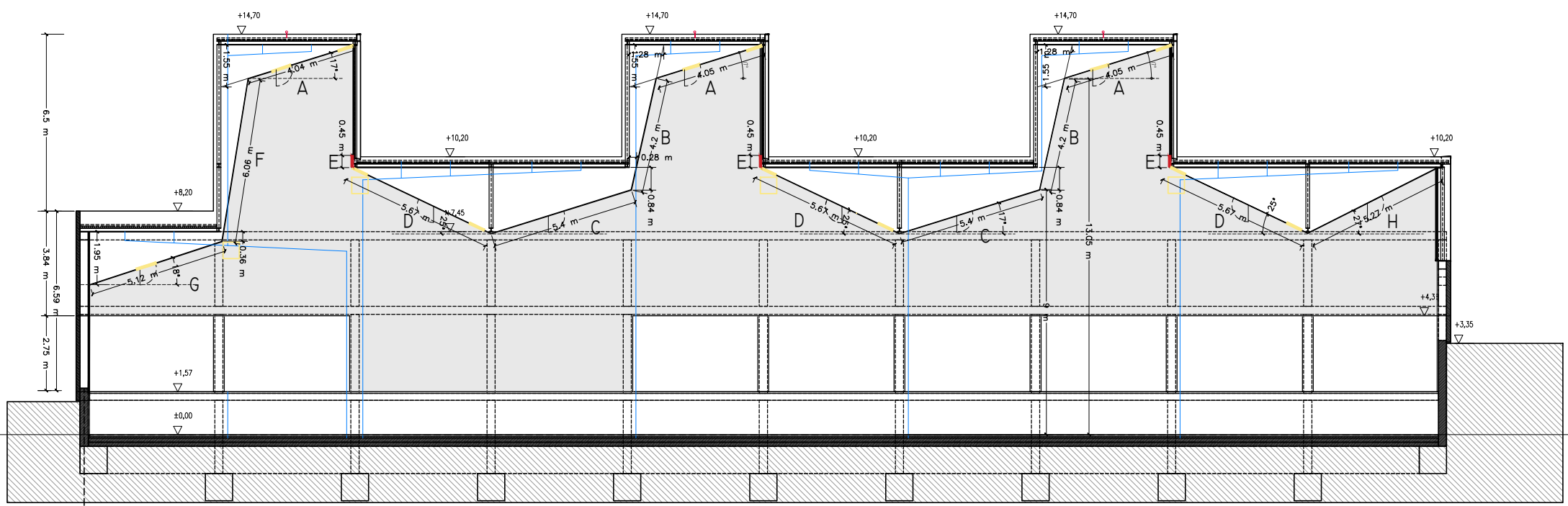
SECCIÓ LONGITUDINAL
