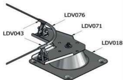
4. Curva en multiposte (NEO)
