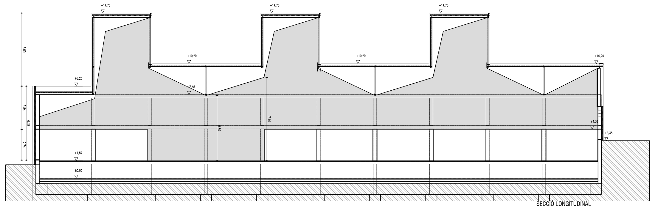
SECCIÓ LONGITUDINAL
