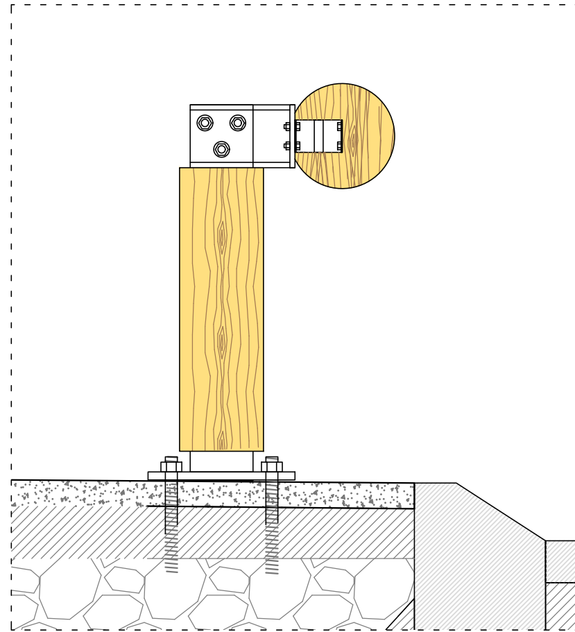
DETALL BARANA DE SEGURETAT TIPUS EURO MB2
