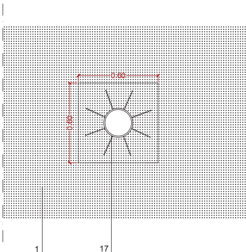
DETALL 4 PLANTA
