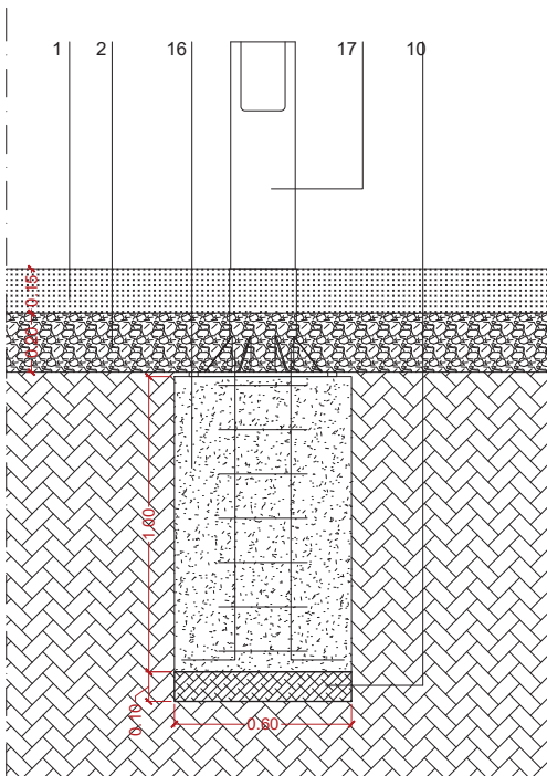
DETALL 4 ALÇAT
