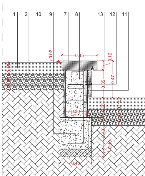
DETALL 2 SECCIÓ
