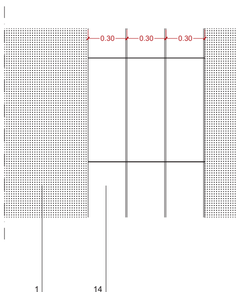
DETALL 3 PLANTA
