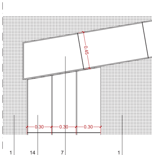
DETALL 5 PLANTA
