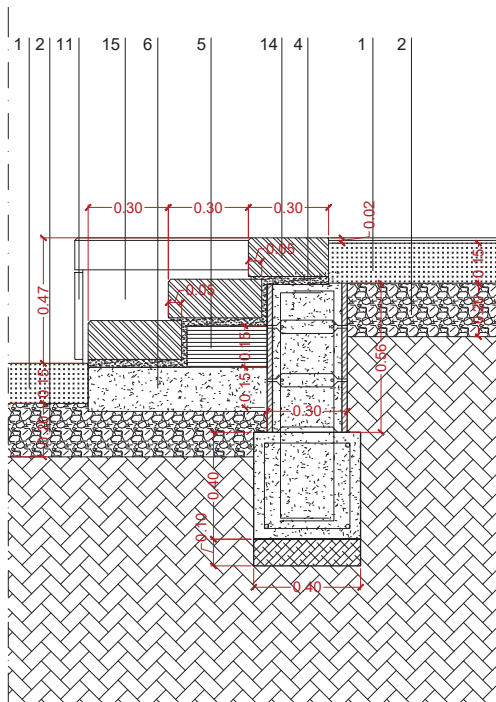
DETALL 5 SECCIÓ
