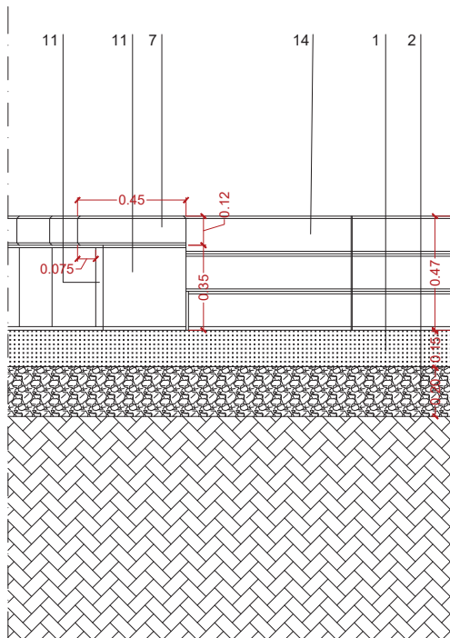
DETALL 5 ALÇAT
