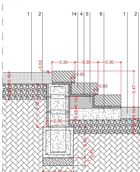
DETALL 3 SECCIÓ
