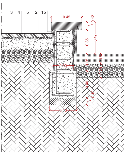
DETALL 1 SECCIÓ
