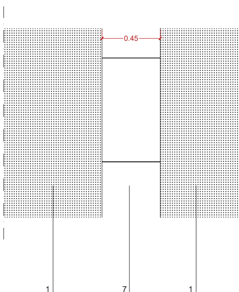
DETALL 2 PLANTA
