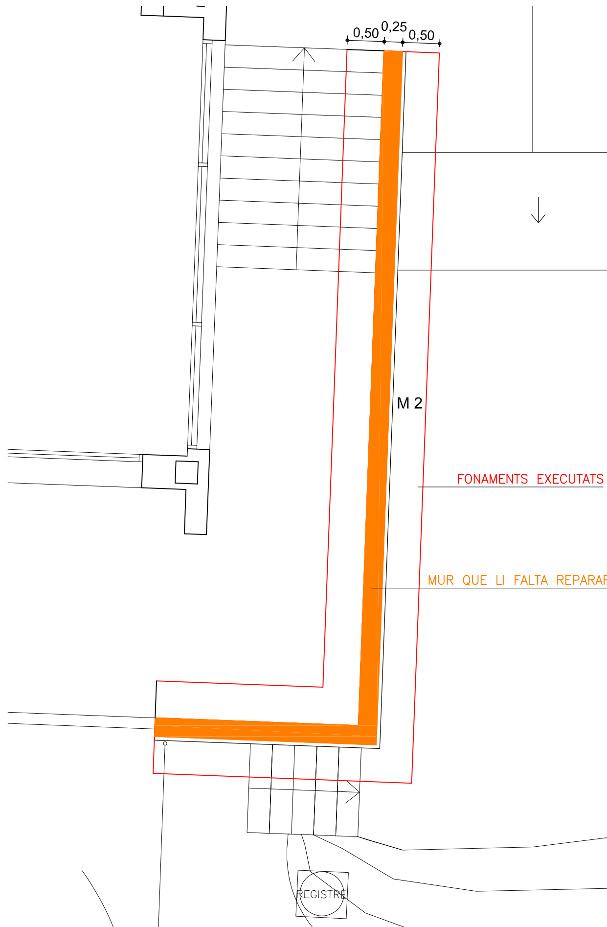
PLANTA FONAMENTS
