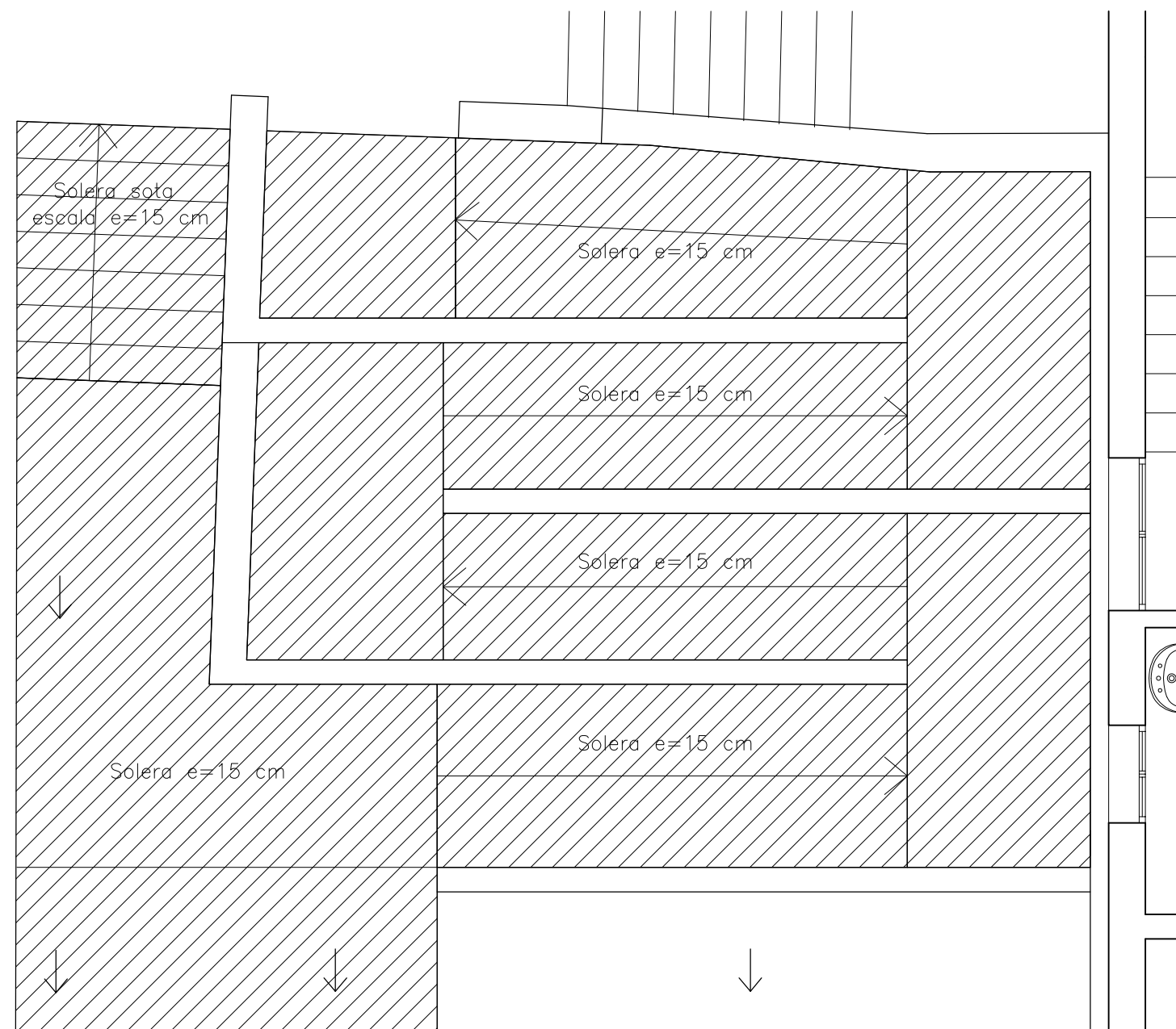
PLANTA SOLERES
