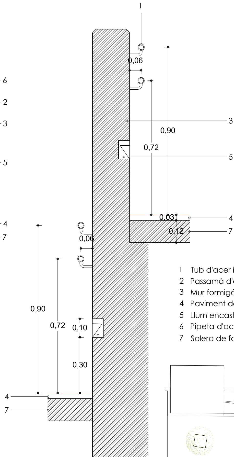
DETALL 2
