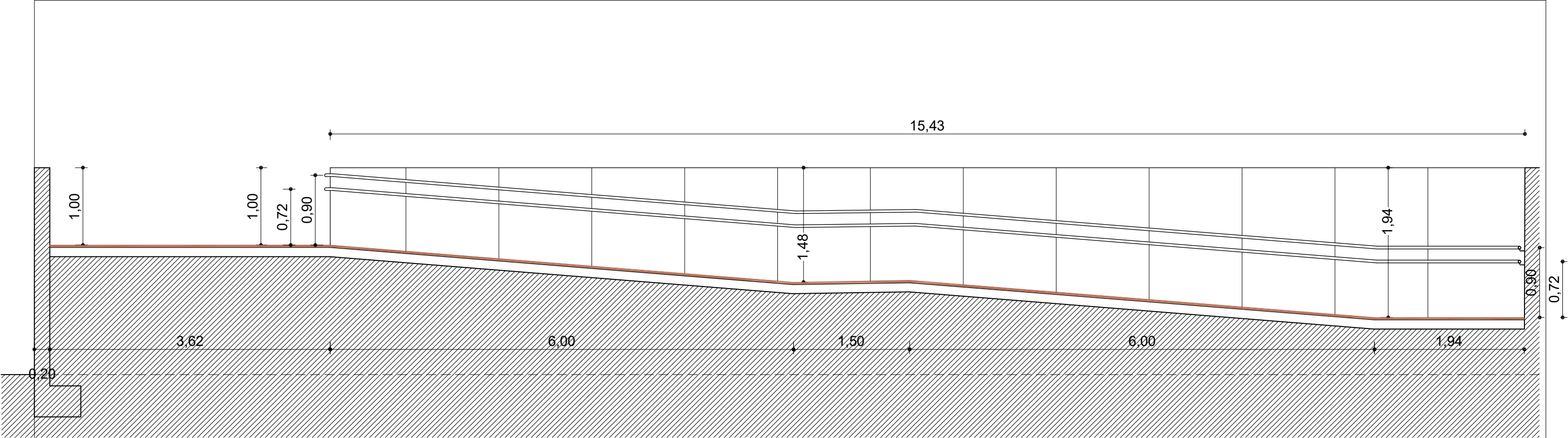
SECCIÓ 3
