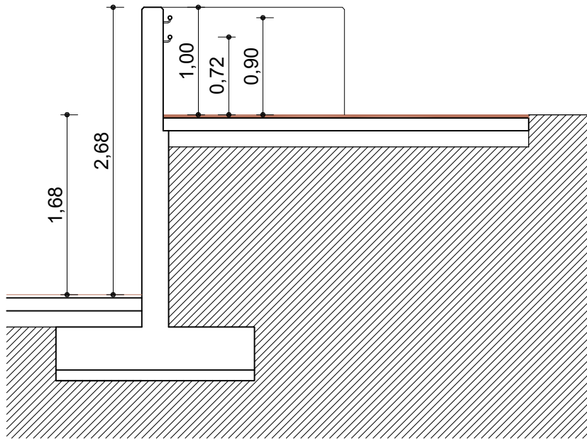
SECCIÓ 4
