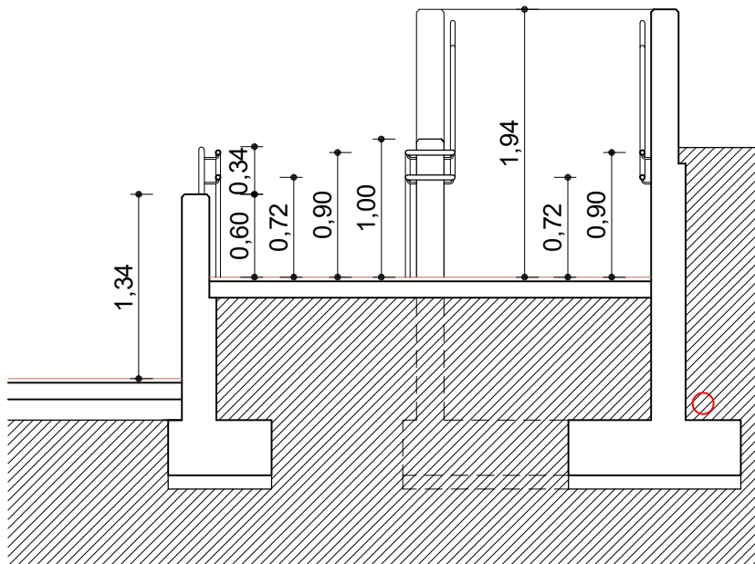
SECCIÓ 6
