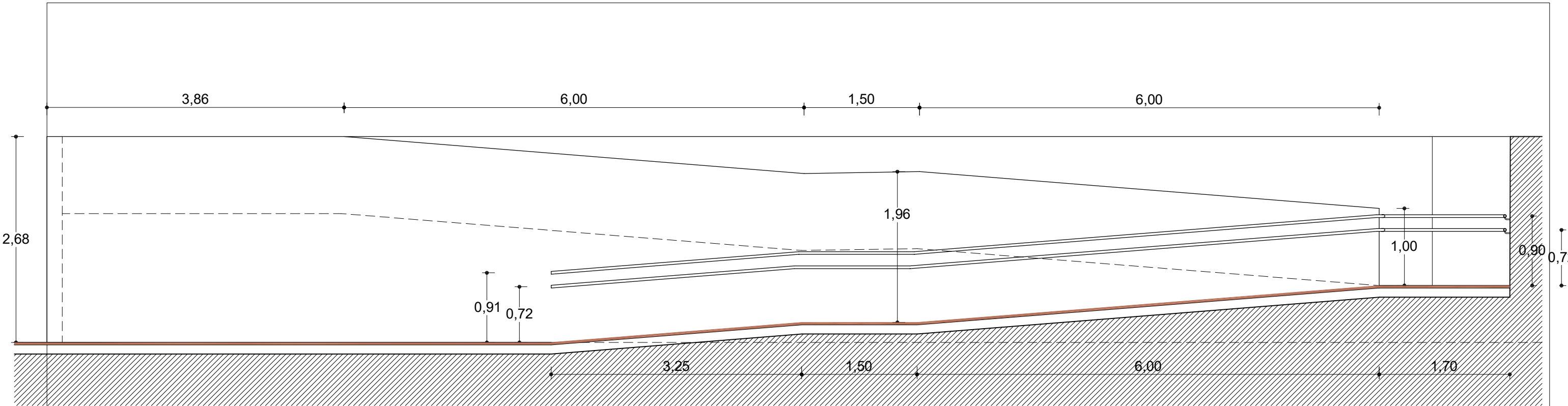
SECCIÓ 2
