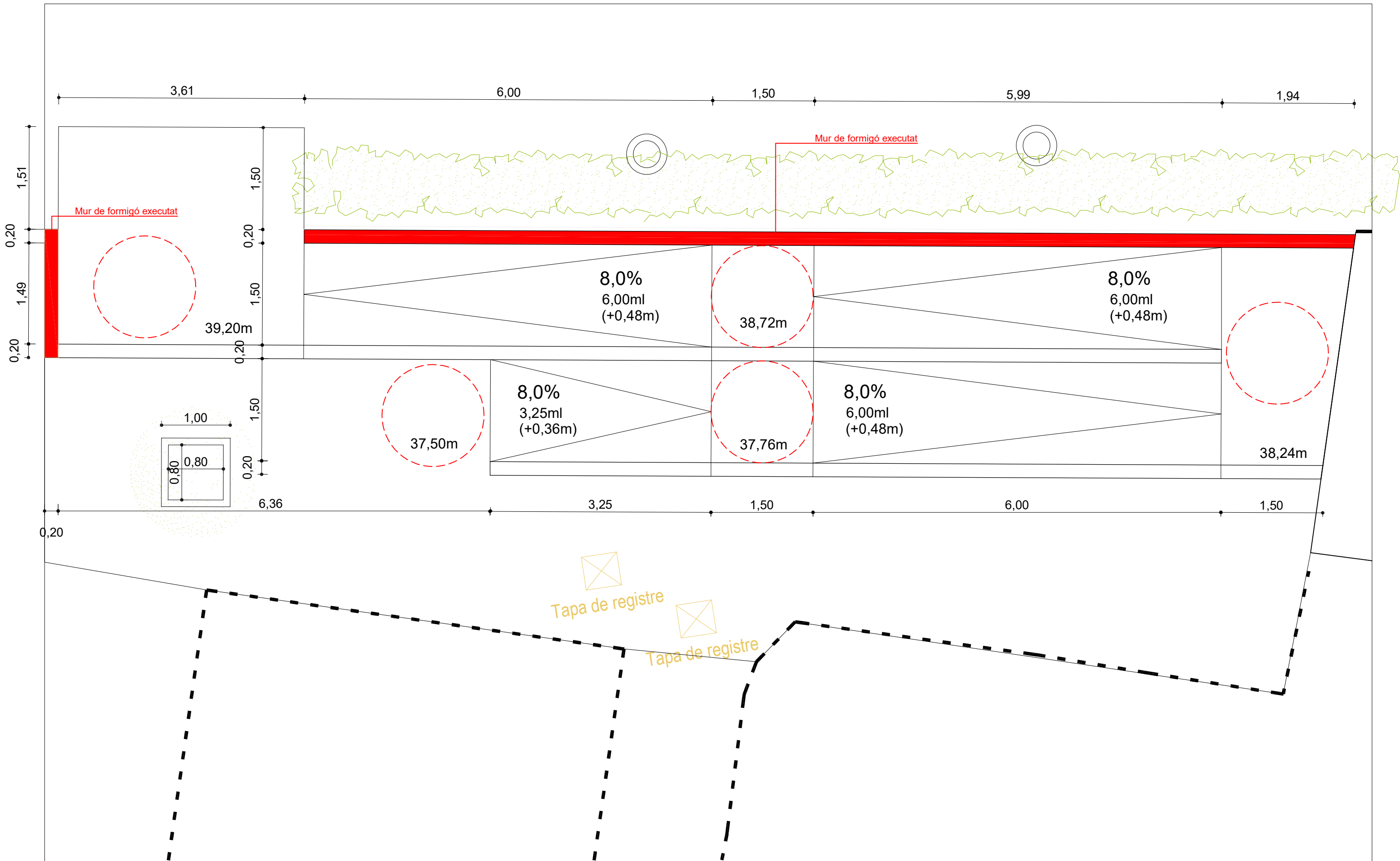
PLANTA
