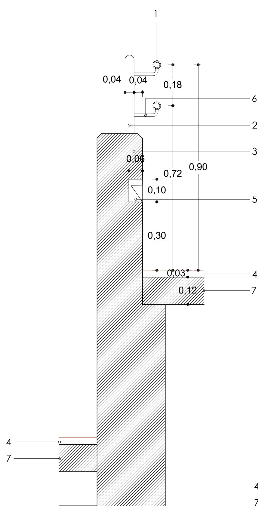
DETALL 1
