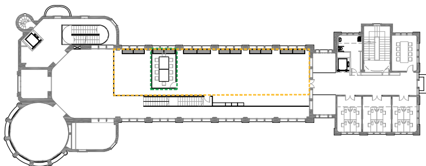
PLANTA ENTRESOL
